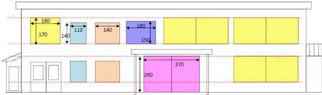
北立面図 S=1/100
