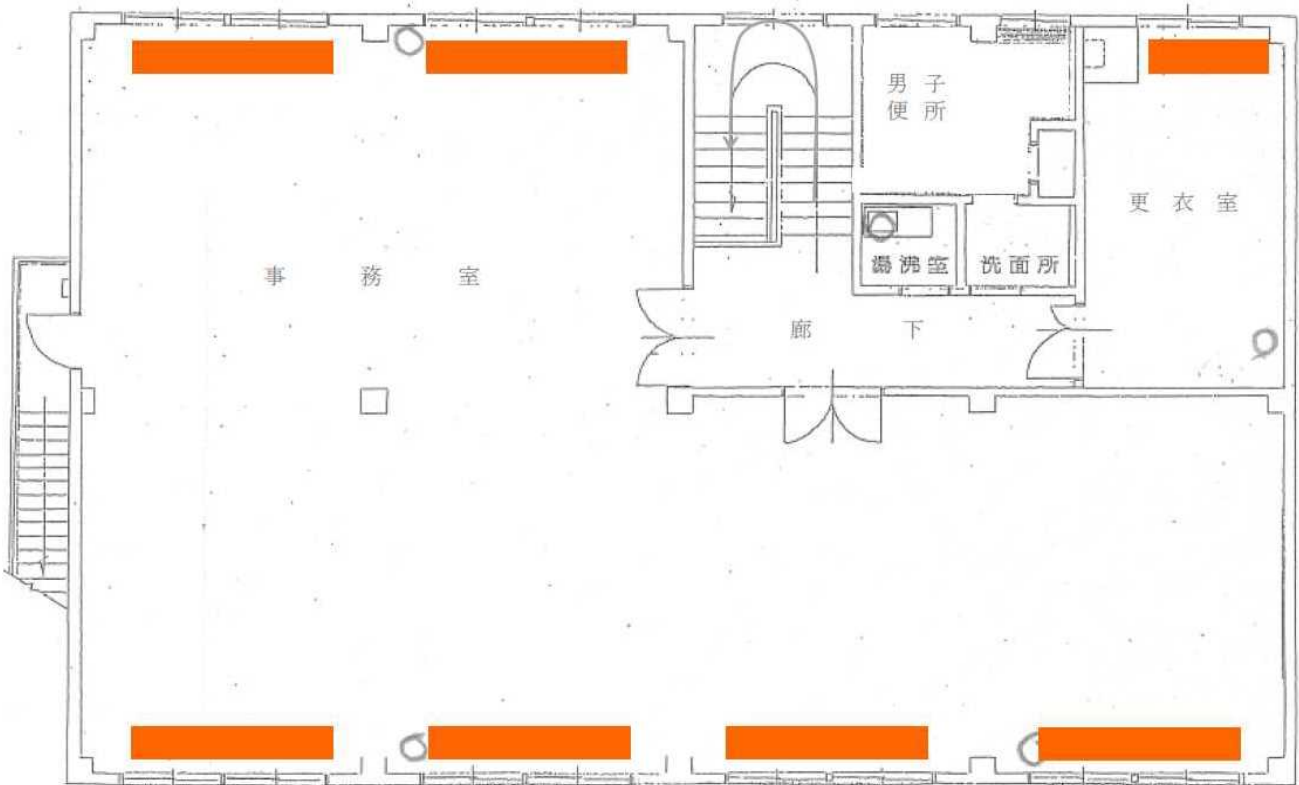
日立パッケージエアコン 7基 ■ 型式:RPF-AP71K
