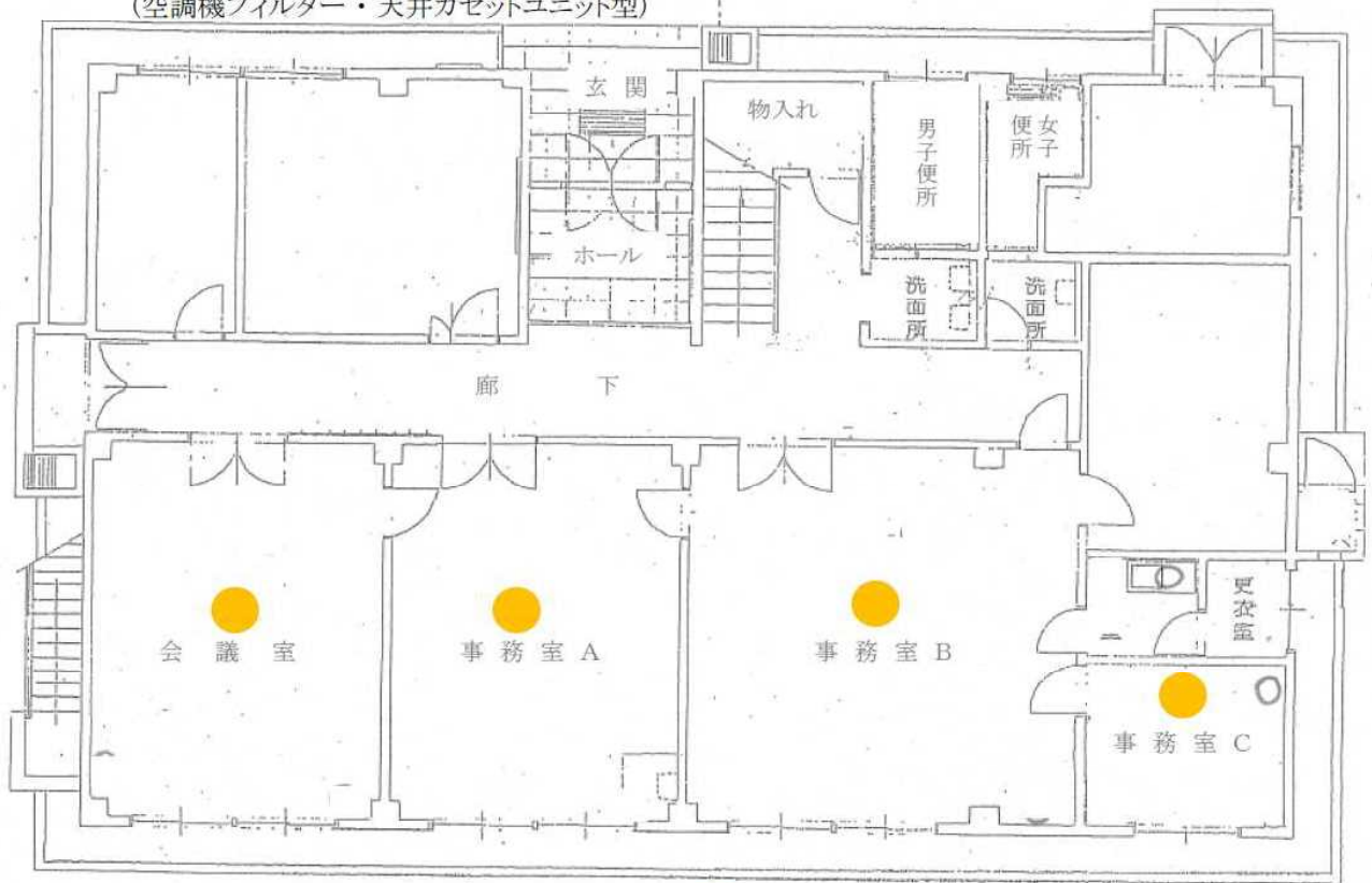
日立パッケージエアコン 4基 ● 会議室・事務室A・事務室B 型式:P-AP160NA 事務室C 型式:P-NP45CWA
