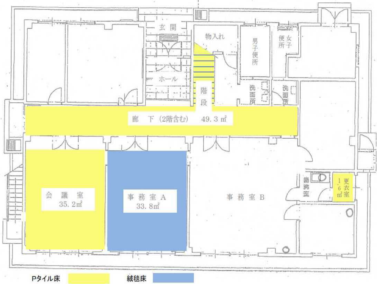
岐阜防衛事務所平面図(床) 1階
