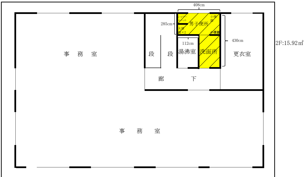
岐阜防衛事務所(2F便所・洗面所・シャワーユニット)
