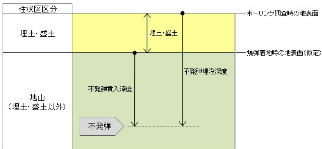
図5. 14 不発弾の貫入深度・埋没深度計算の考え方
