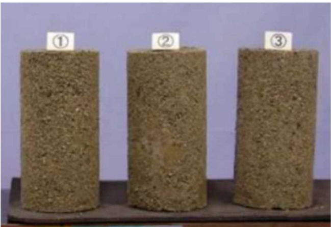
土の試料の一例（Avf-c）
