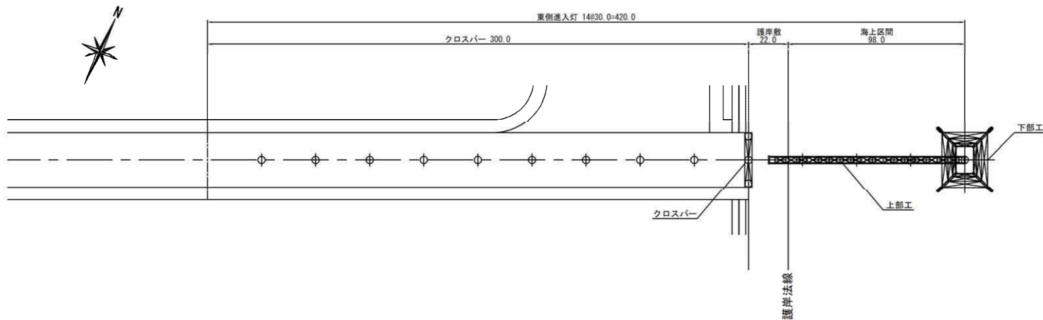
平面図
