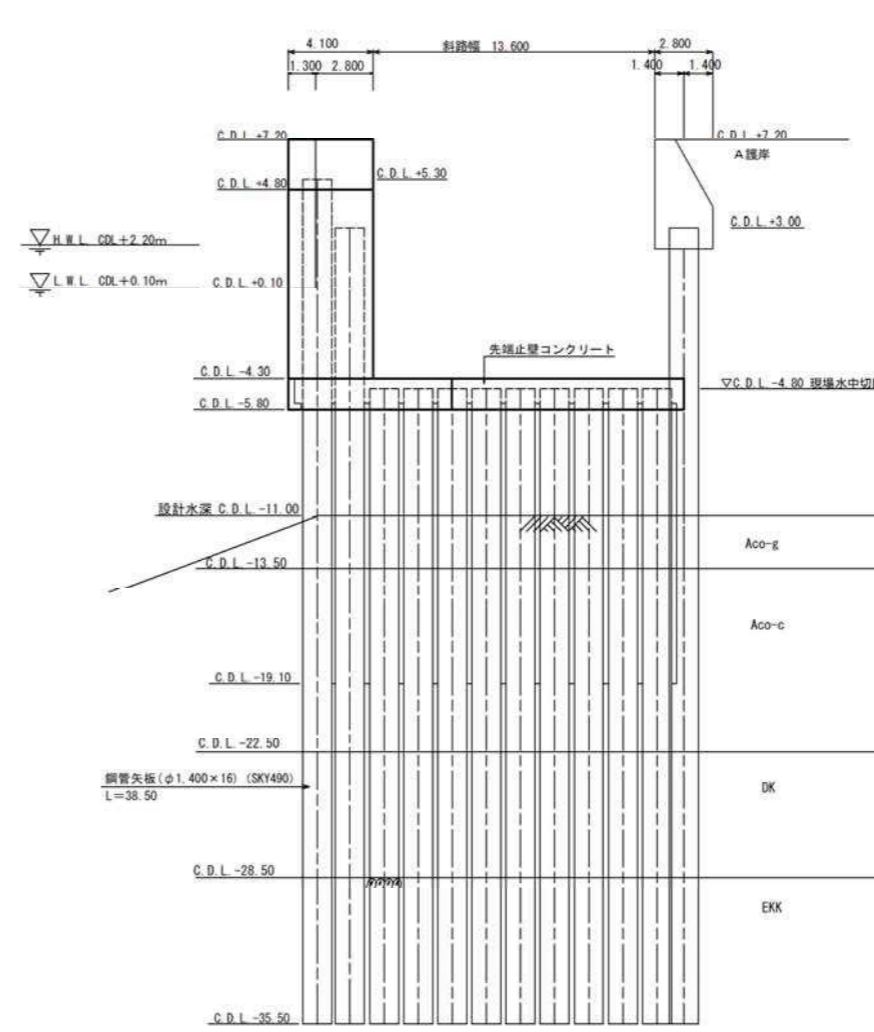
斜路前面壁正面図（自立式）
