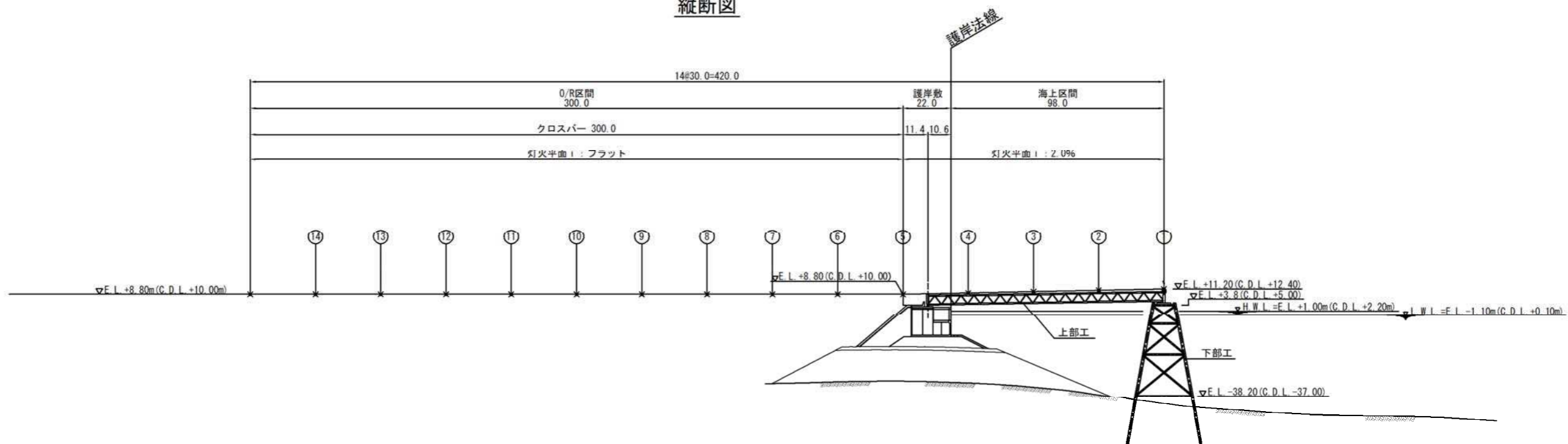
縦断図
