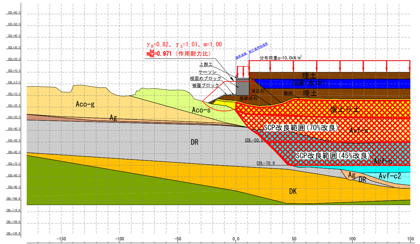
図7 隅角部護岸(HB側) 完成時
