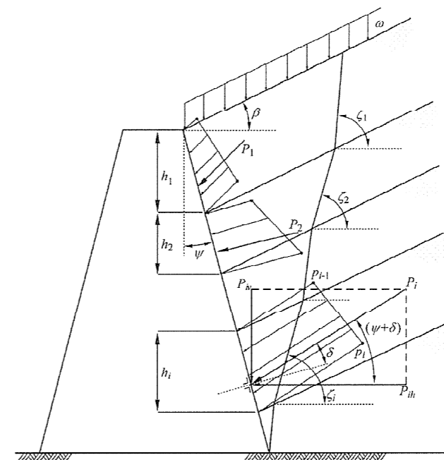
図-2.2.1 土圧
