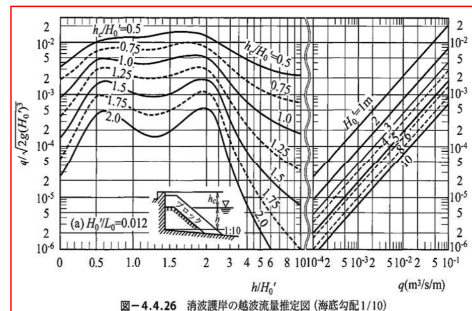
図-4.4.26 消波護岸の越波流量推定図（海底勾配1/10）
