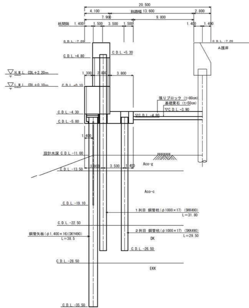
斜路断面図（柵式）
