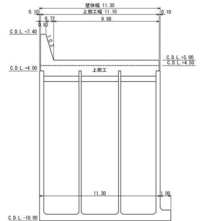
図 3.2-6 断面(隅角部護岸(HB側))
