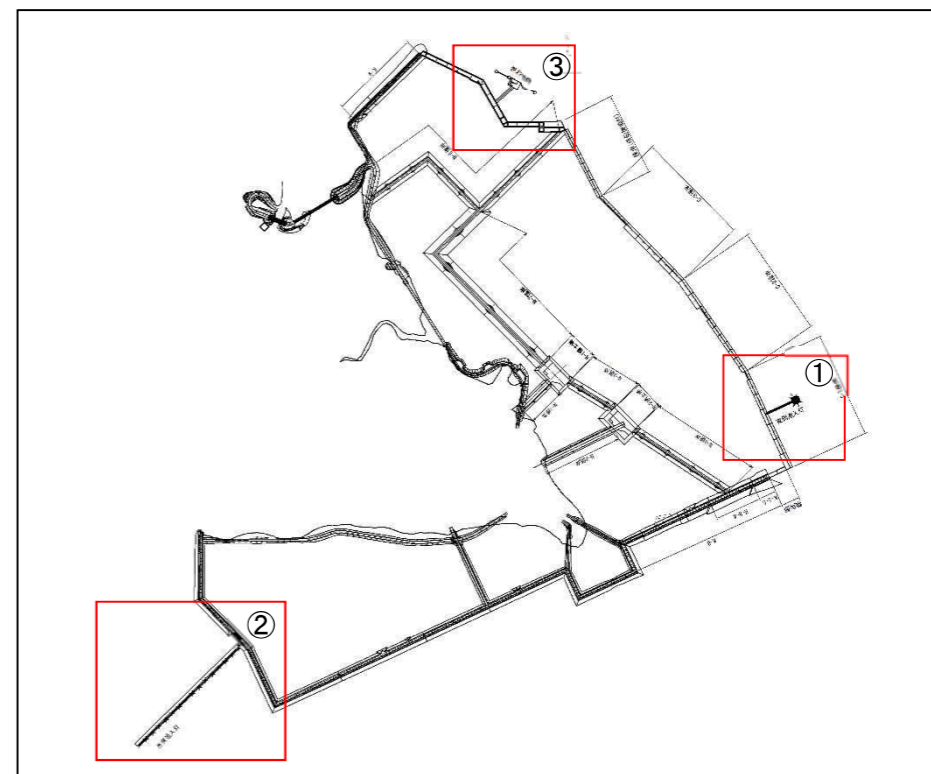
図 3.1-1 対象施設の位置
