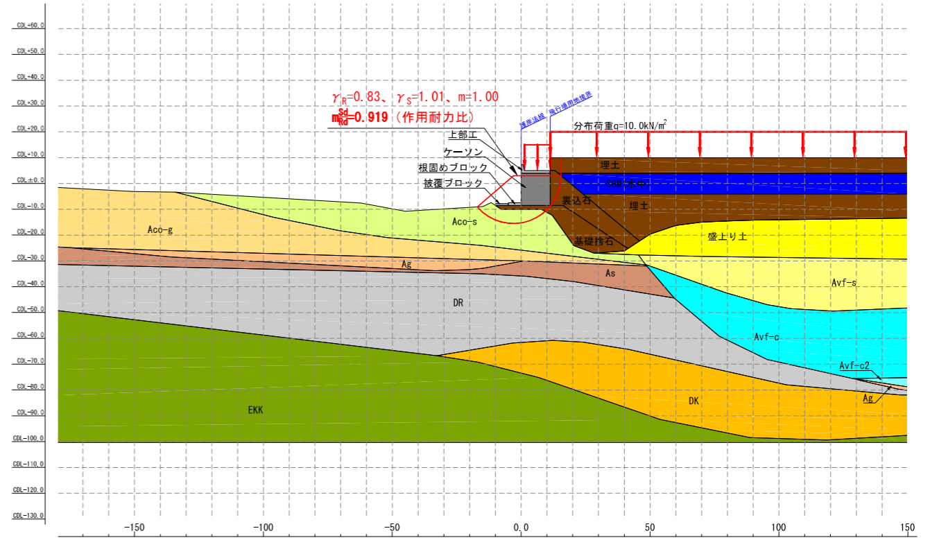
図6 隅角部護岸(傾斜堤側) 完成時
