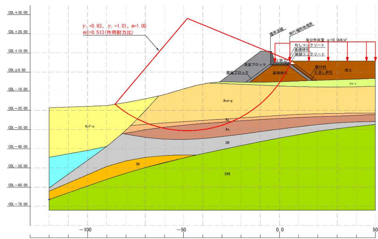
図10 K-8 護岸(K-8-4) 完成時
