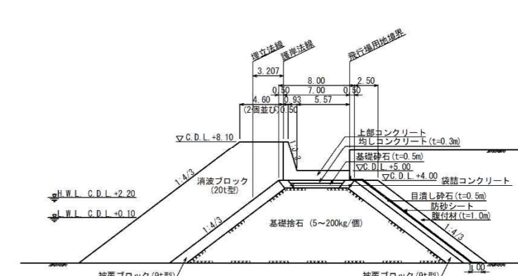
図 3.1-6 K-9 護岸
