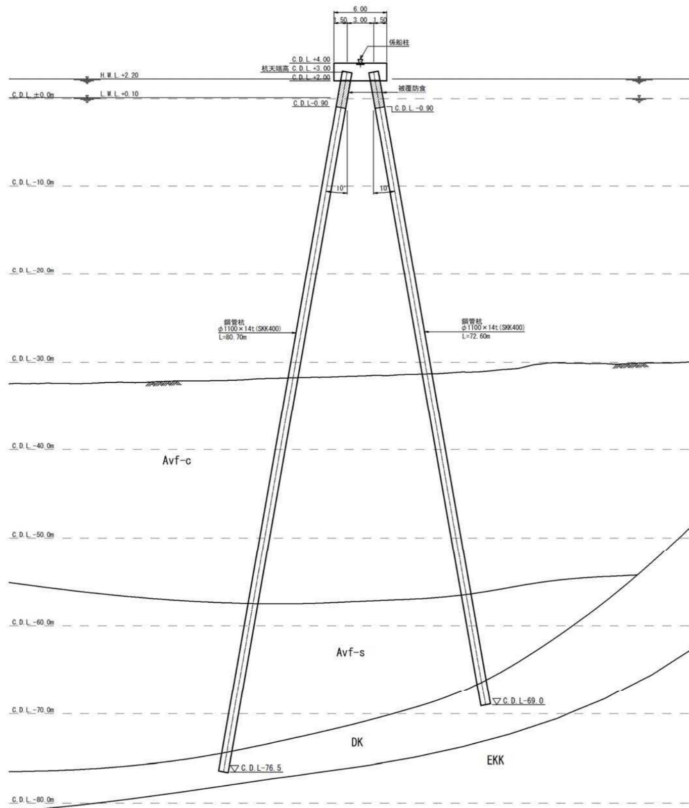
東側 綱取ドルフィン
