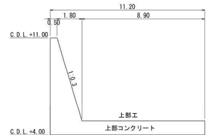
図 3.2-8 断面(K-8 護岸(K-8-5))
