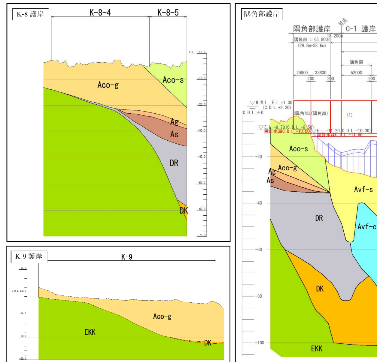
図3 地層縦断図
