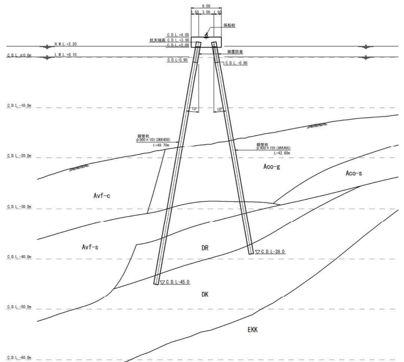
西側 綱取ドルフィン
