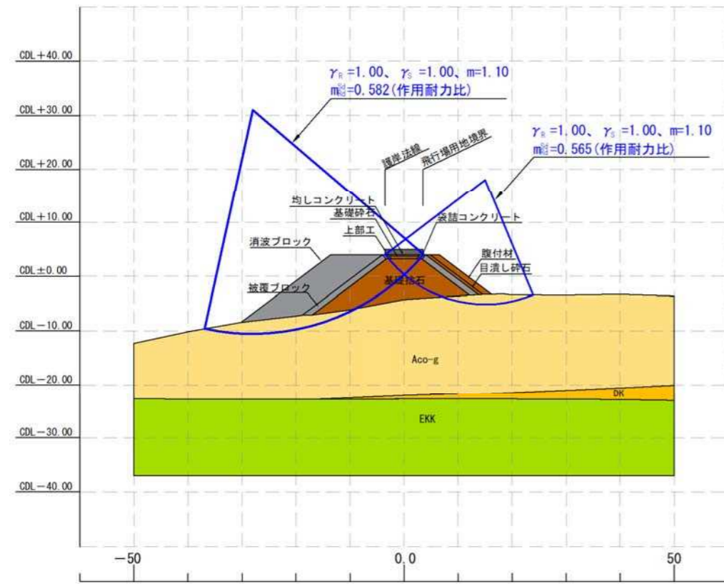
図 12 K-9 護岸 施工時
