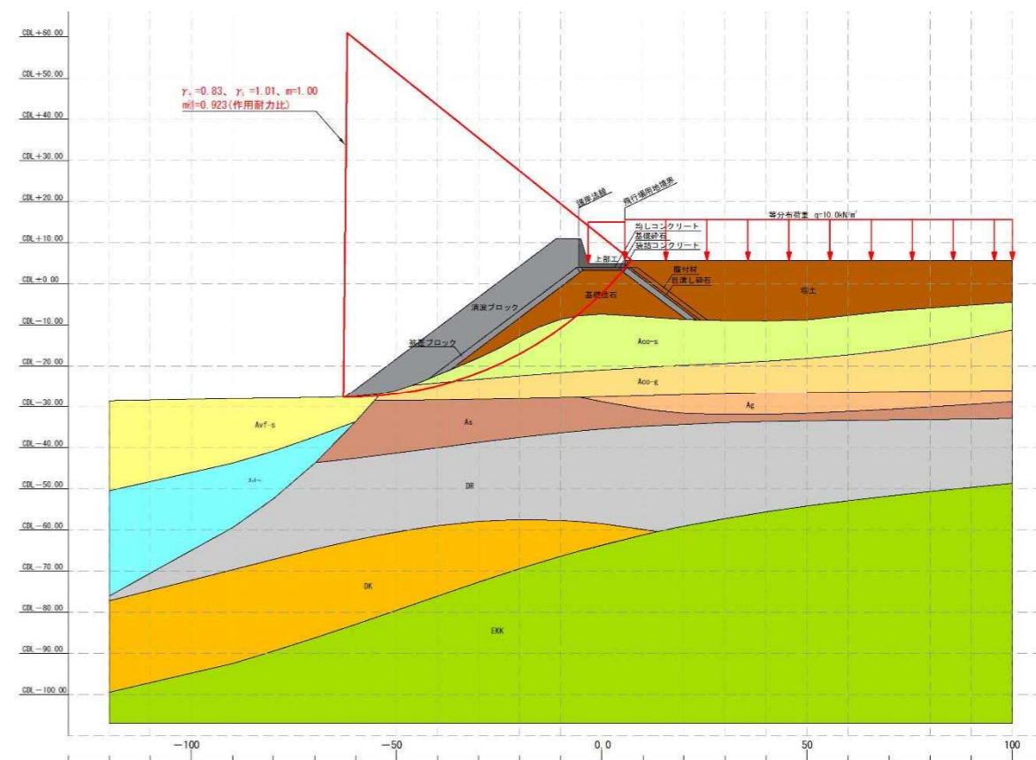
図11 K-8 護岸(K-8-5) 完成時
