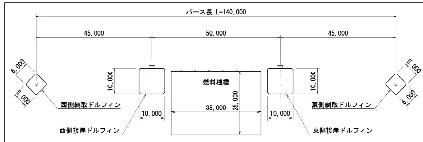
図 4.1-2 燃料棧橋、接岸ドルフィン、綱取ドルフィンの配置図
