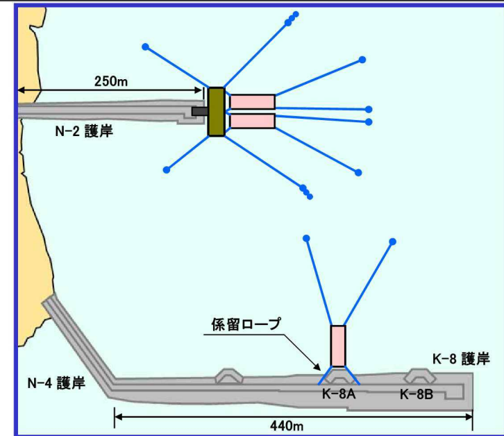
K-8護岸を用いた揚土(イメージ)
