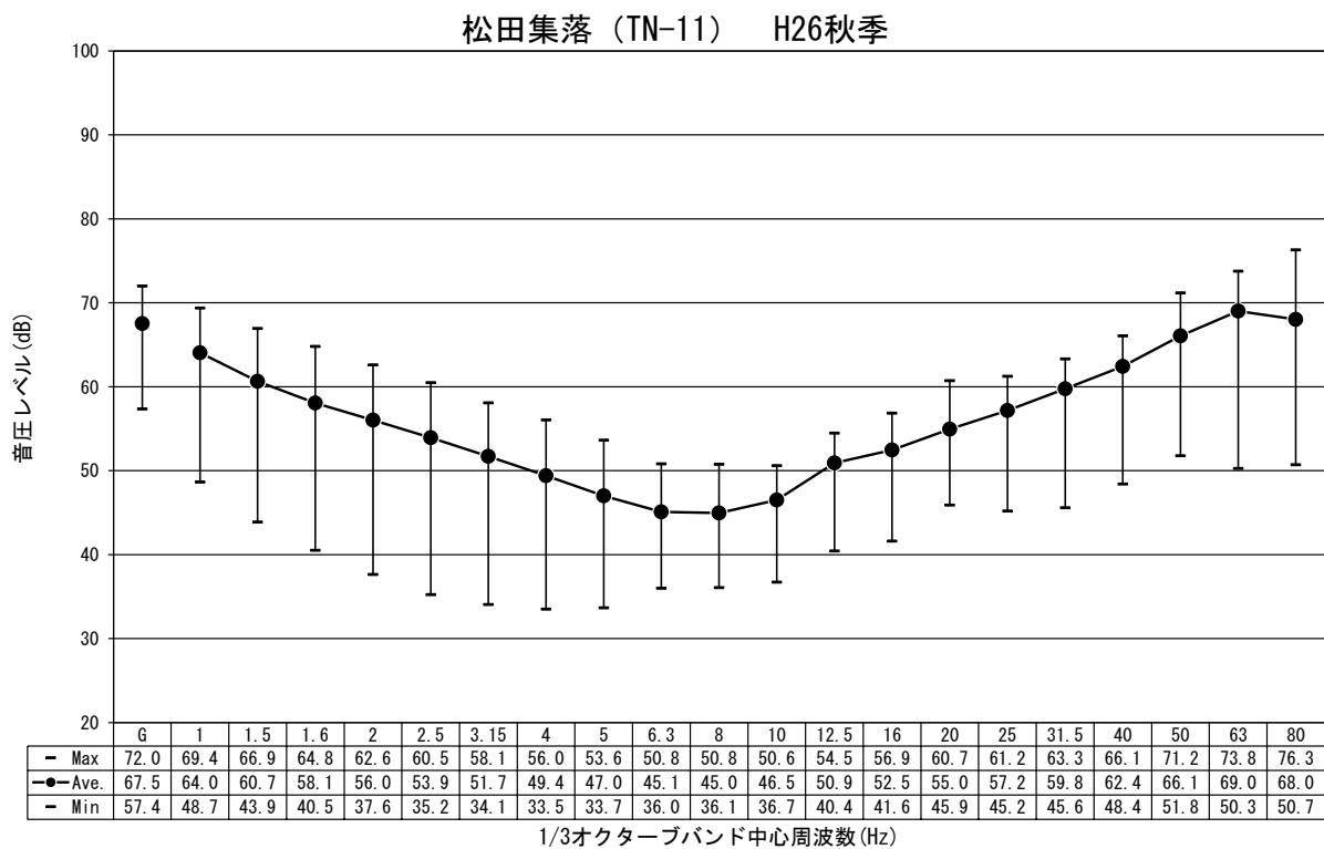
図-2.1.4.7(3) 低周波音の調査結果 (平成26年度秋季)
