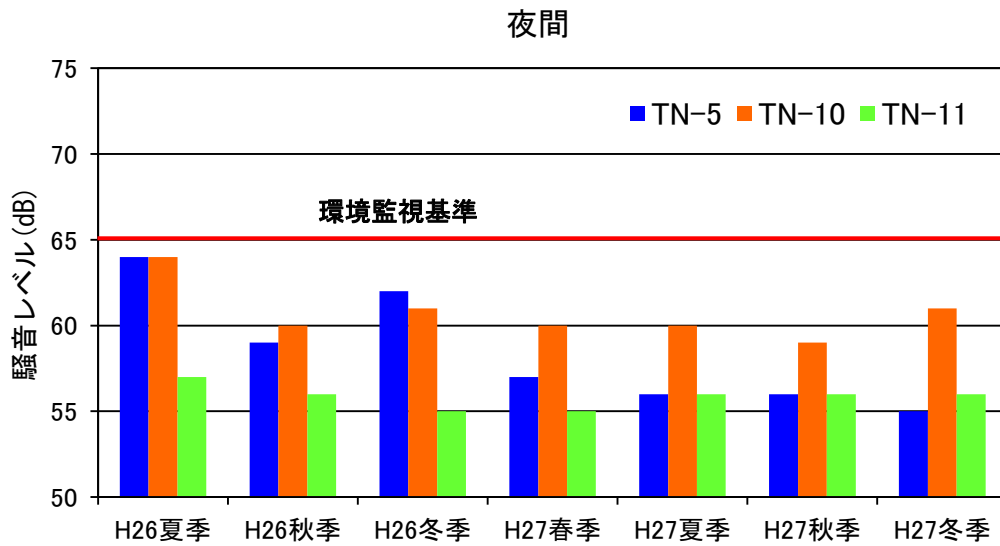
図-2.1.2.1 道路交通騒音の調査結果
