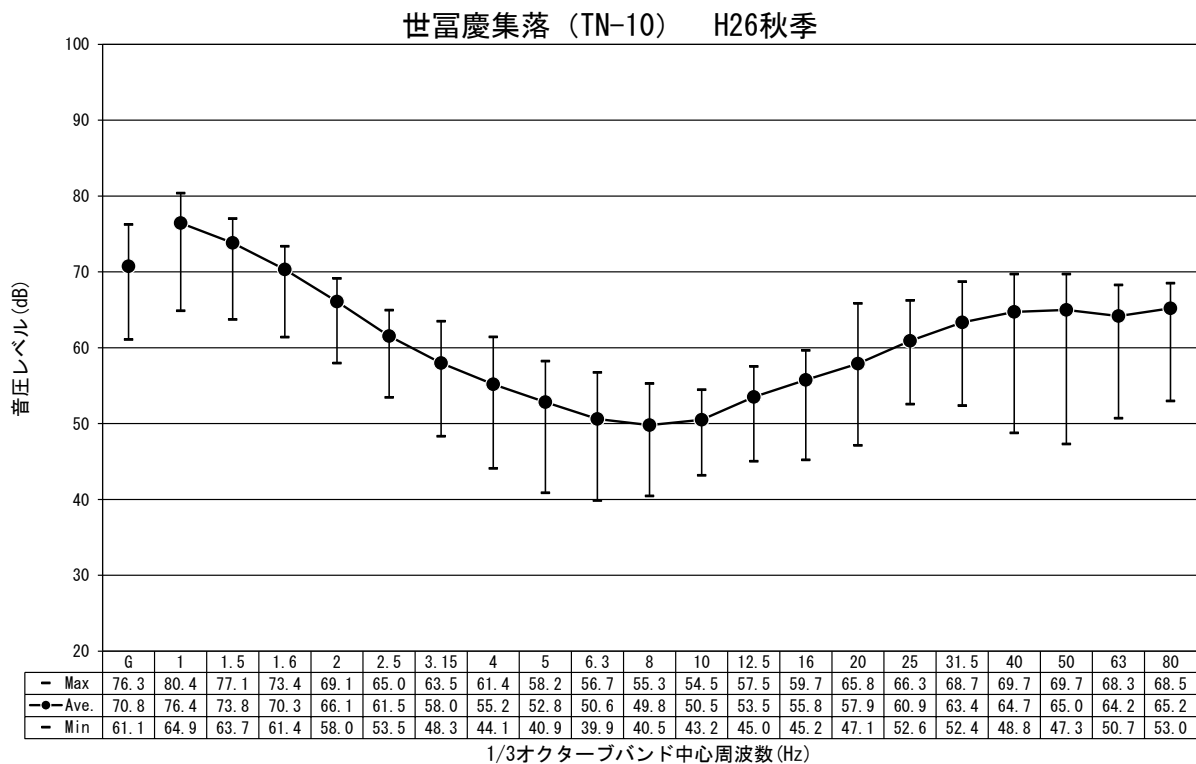
図-2.1.4.7(2) 低周波音の調査結果 (平成26年度秋季)
