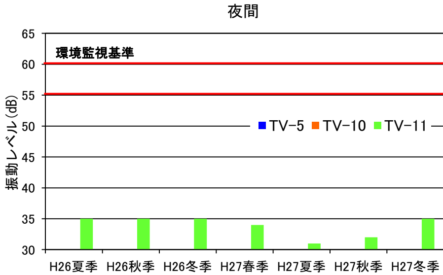
図-2.1.3.1 道路交通振動の調査結果
