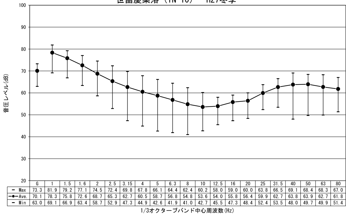
図-2.1.4.12(2) 低周波音の調査結果 (平成 27 年度冬季)
