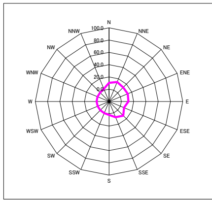
図-2.1.4.5 風向別平均風速、風向別出現頻度 (平成27年度春季から冬季)
