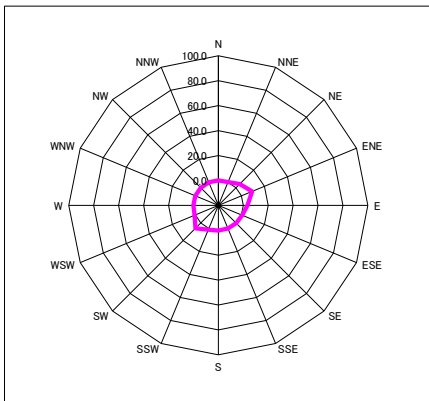
図-2.1.4.18 風向別平均風速、風向別出現頻度(平成27年度秋季)
