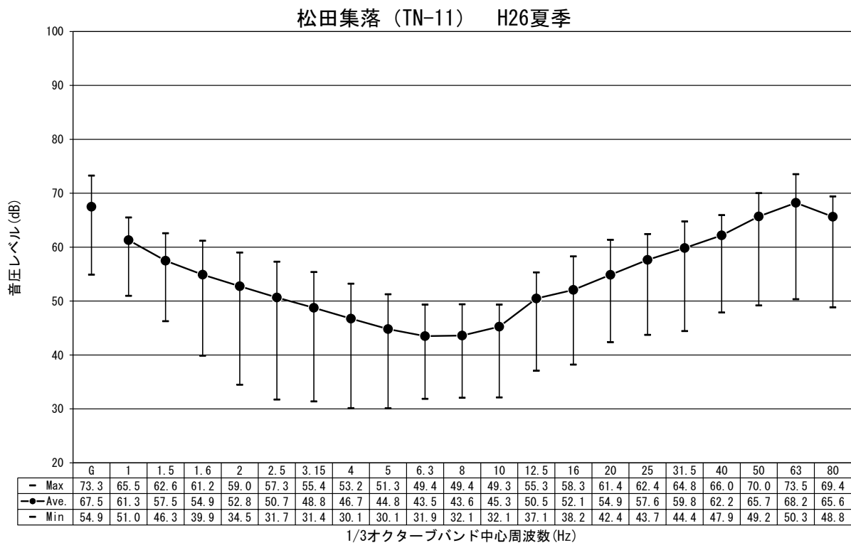
図-2.1.4.6(3) 低周波音の調査結果 (平成26年度夏季)
