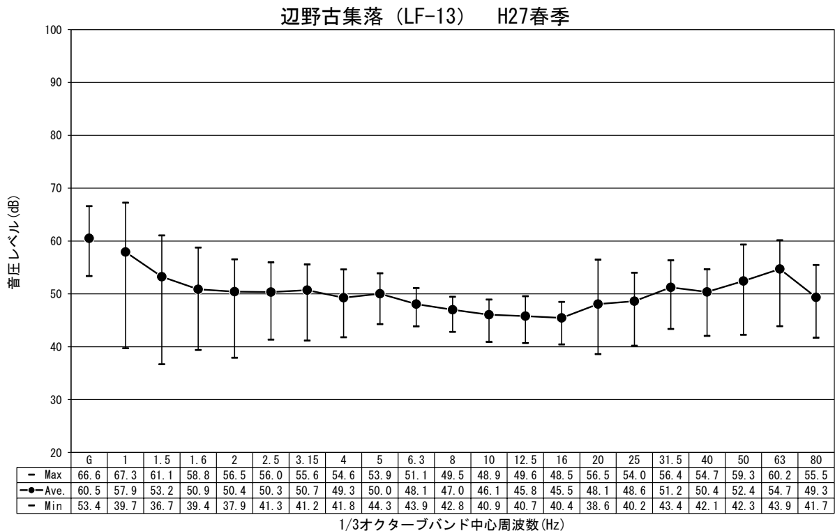
図-2.1.4.1 低周波音の調査結果 (平成27年度春季)
