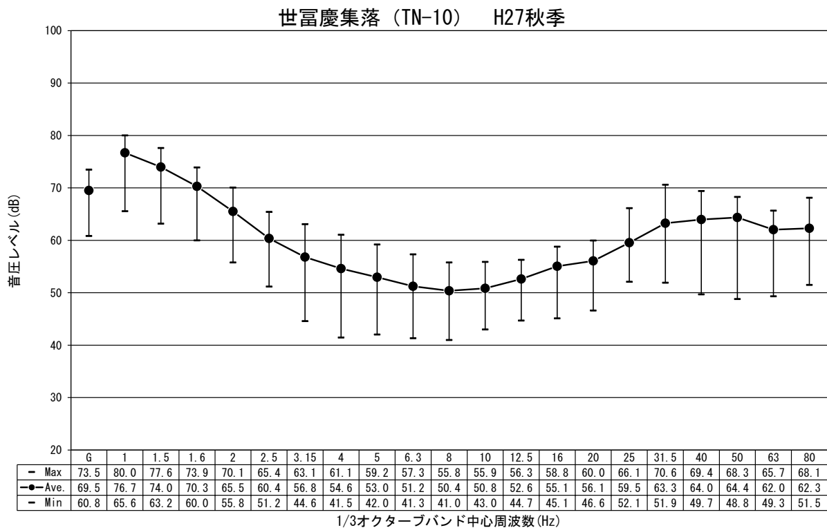
図-2.1.4.11(2) 低周波音の調査結果 (平成 27 年度秋季)
