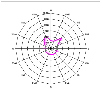
図-2. 1. 1. 10 風向別平均風速、風向別出現頻度 (平成 26 年度冬季)
