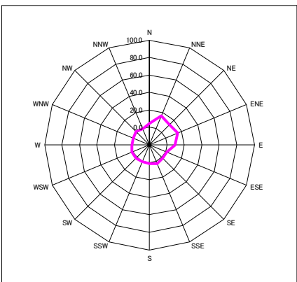
図-2. 1. 1. 12 風向別平均風速、風向別出現頻度 (平成 27 年度夏季)
