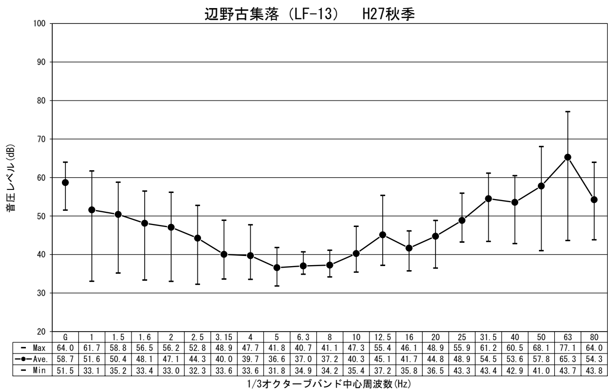
図-2.1.4.3 低周波音の調査結果 (平成 27 年度秋季)
