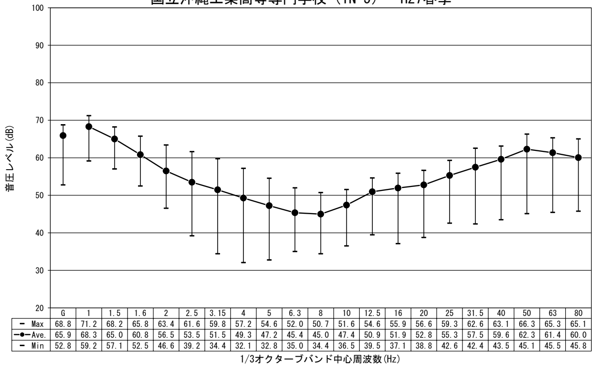
図-2.1.4.9(1) 低周波音の調査結果 (平成 27 年度春季)
