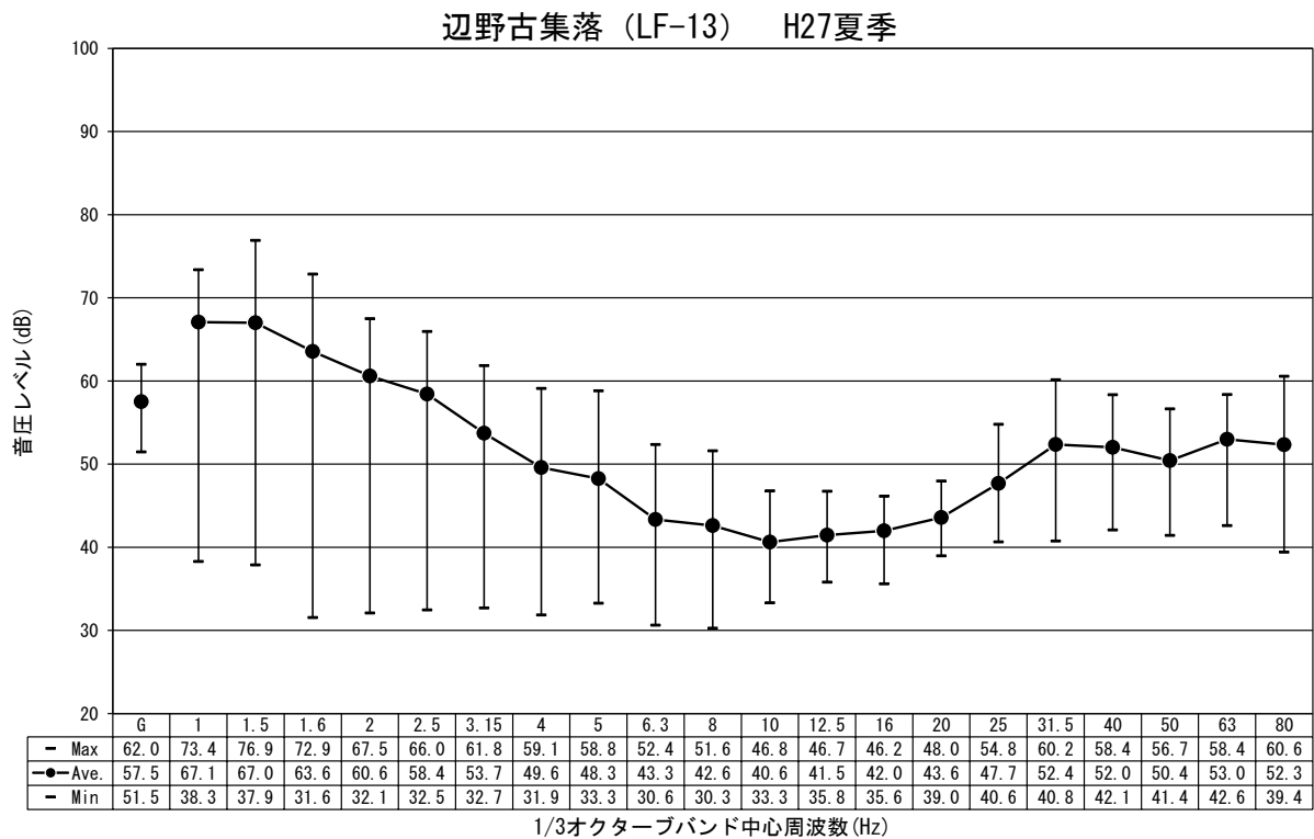
図-2.1.4.2 低周波音の調査結果 (平成 27 年度夏季)
