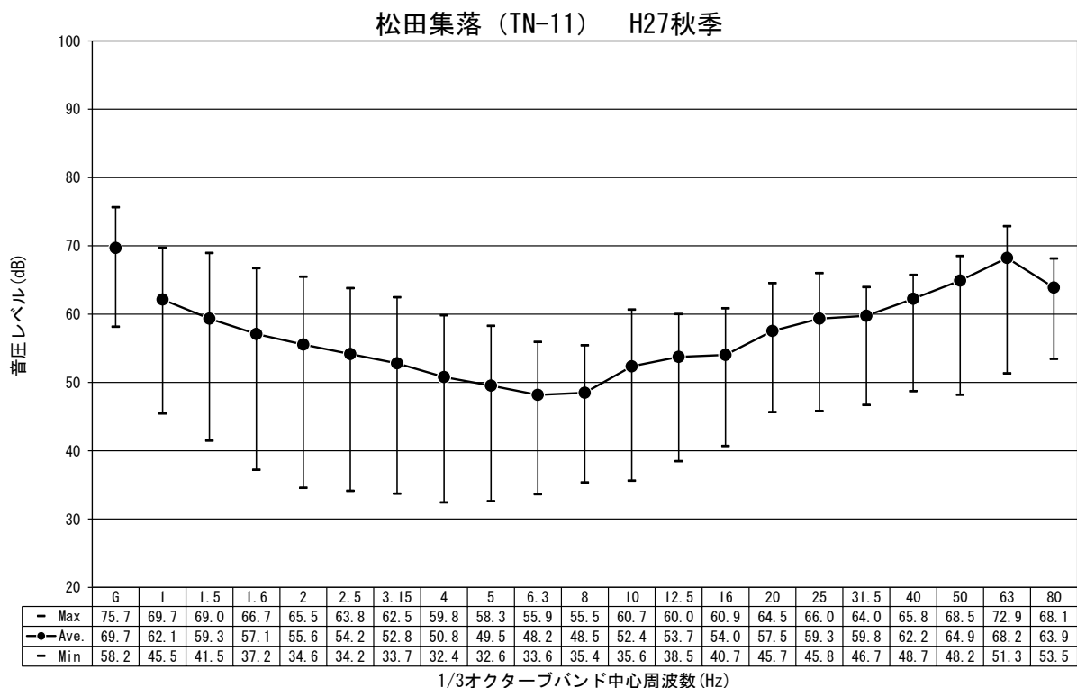
図-2.1.4.11(3) 低周波音の調査結果 (平成 27 年度秋季)
