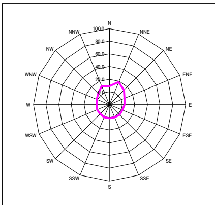
図-2. 1. 1. 4 風向別平均風速、風向別出現頻度 (平成27年度春季)
