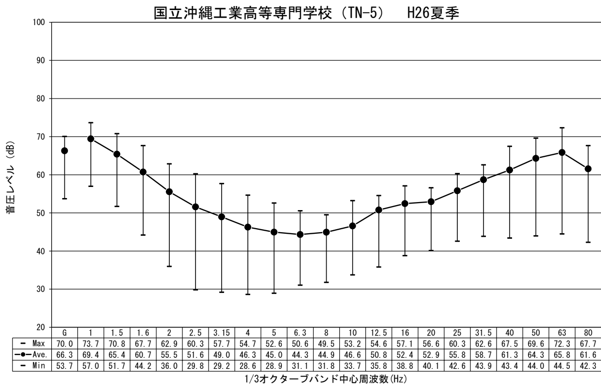
図-2. 1. 4. 6(1) 低周波音の調査結果 (平成 26 年夏季)
