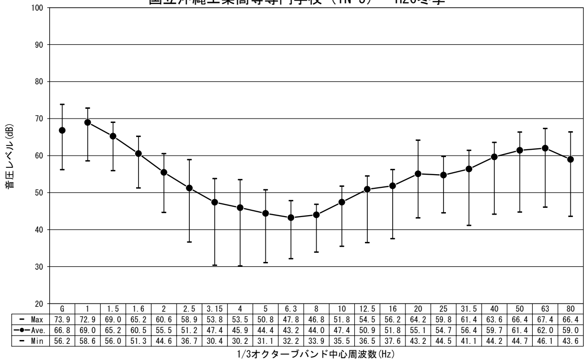
図-2.1.4.8(1) 低周波音の調査結果 (平成 26 年度冬季)
