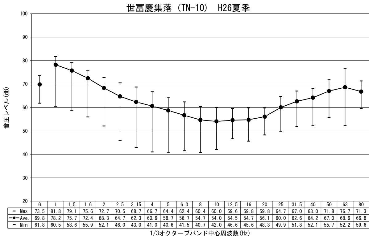
図-2. 1. 4. 6(2) 低周波音の調査結果 (平成 26 年度夏季)
