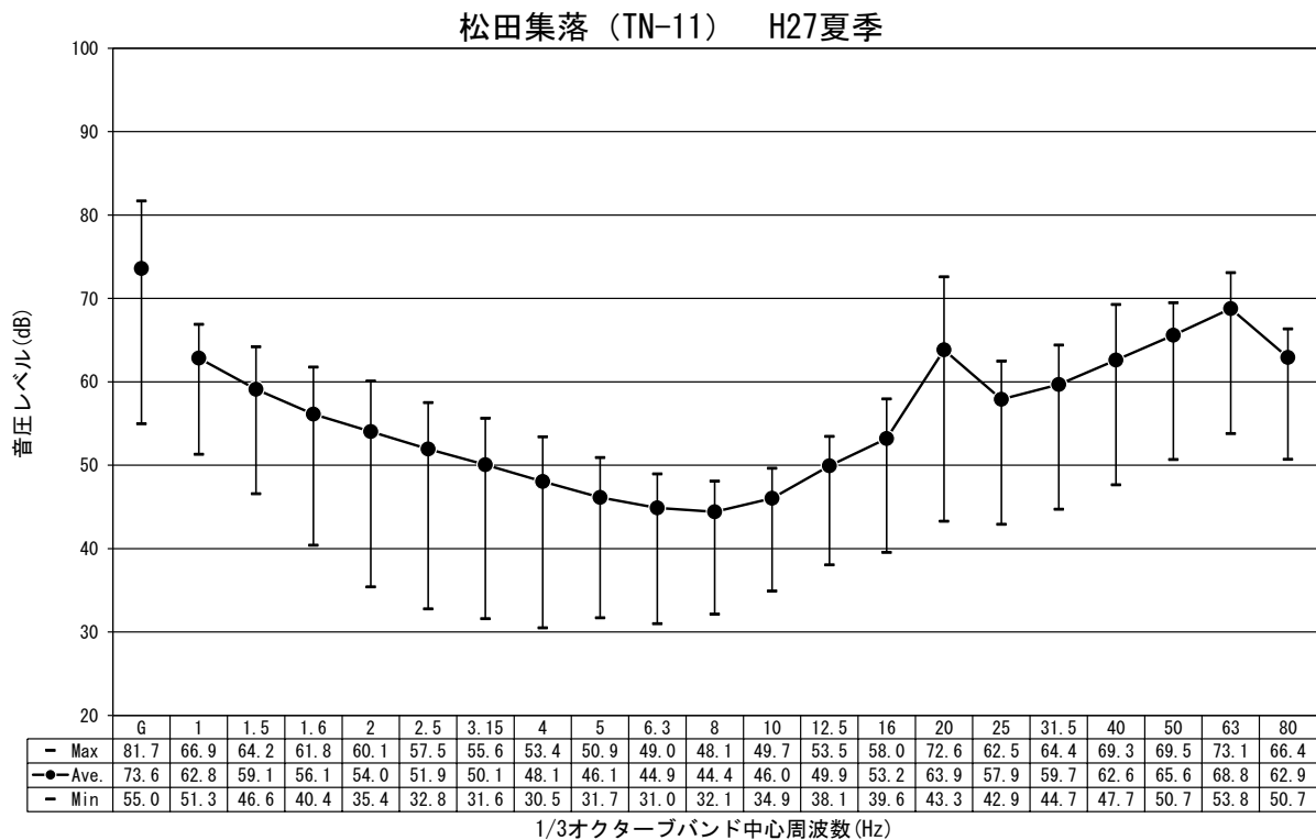
図-2.1.4.10(3) 低周波音の調査結果 (平成 27 年度夏季)
