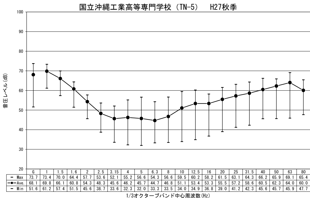
図-2.1.4.11(1) 低周波音の調査結果 (平成 27 年度秋季)
