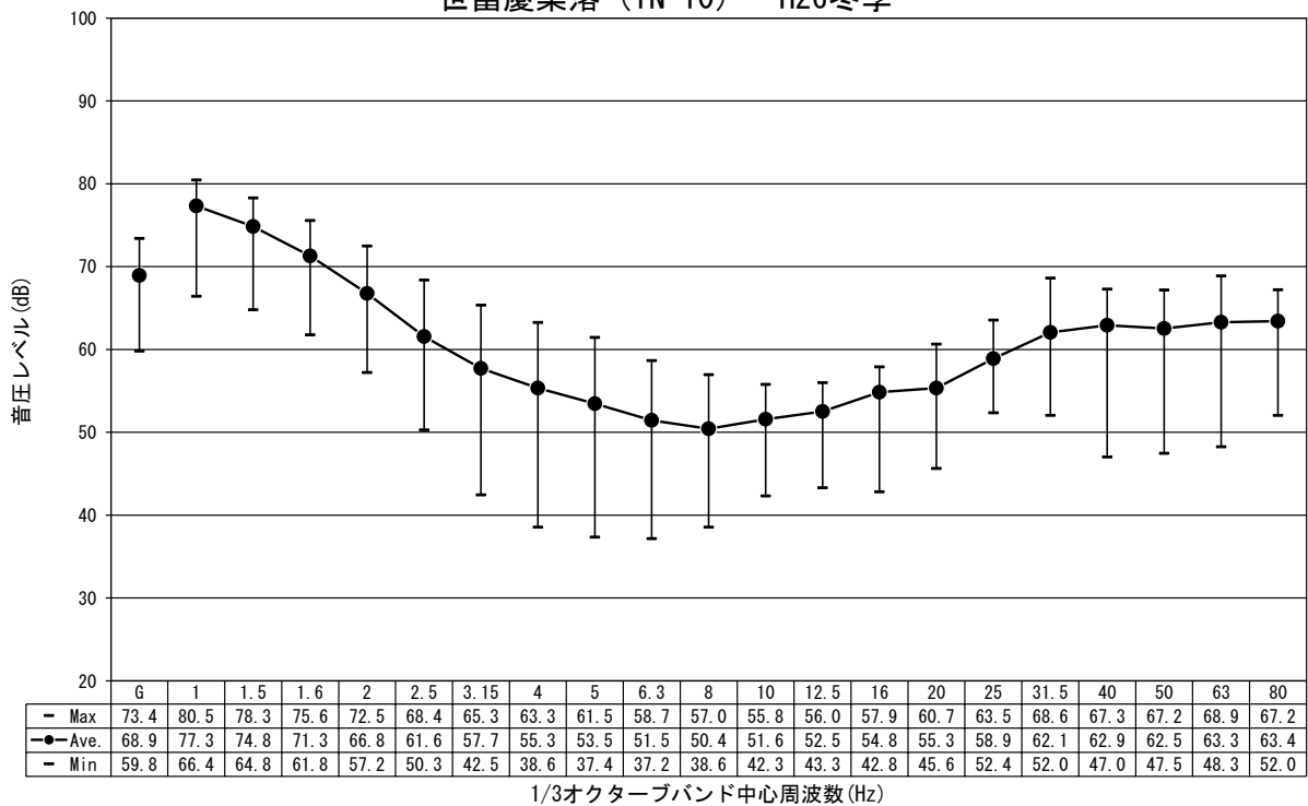
図-2.1.4.8(2) 低周波音の調査結果 (平成 26 年度冬季)
