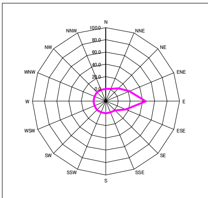
図-2.1.4.16 風向別平均風速、風向別出現頻度(平成27年度春季)
