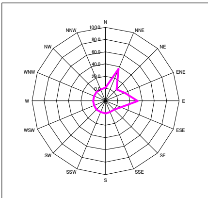
図-2. 1. 1. 9 風向別平均風速、風向別出現頻度 (平成 26 年度秋季)
