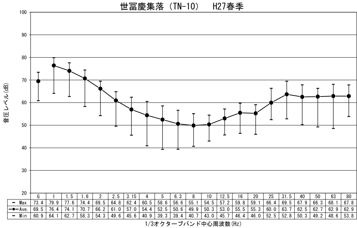
図-2.1.4.9(2) 低周波音の調査結果 (平成 27 年度春季)
