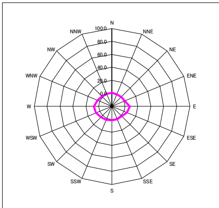
図-2.1.4.13 風向別平均風速、風向別出現頻度(平成26年度夏季)
