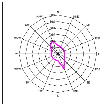
図-2.1.1.6 風向別平均風速、風向別出現頻度 (平成27年度秋季)
