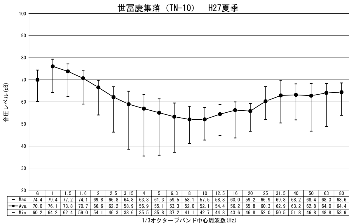
図-2.1.4.10(2) 低周波音の調査結果 (平成 27 年度夏季)
