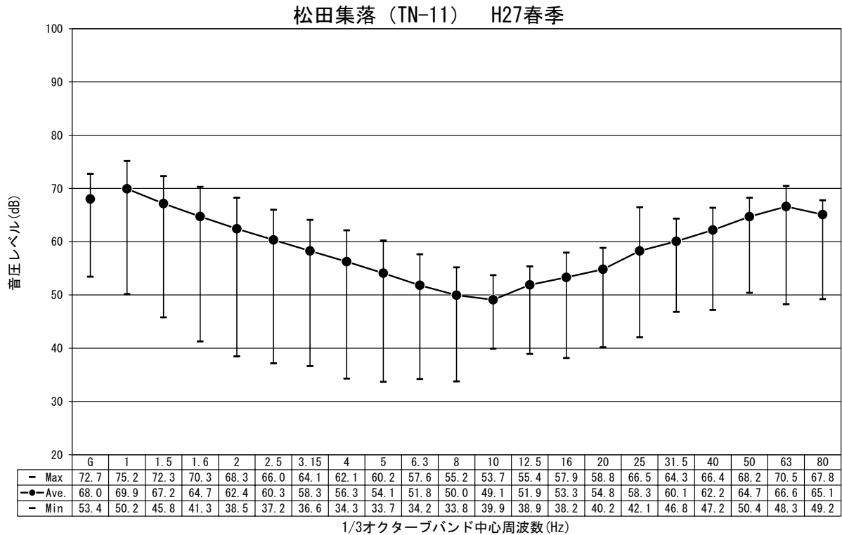
図-2.1.4.9(3) 低周波音の調査結果 (平成 27 年度春季)
