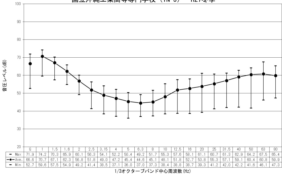
図-2.1.4.12(1) 低周波音の調査結果 (平成 27 年度冬季)
