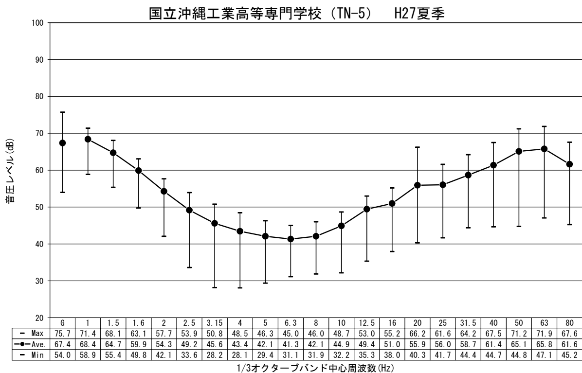
図-2.1.4.10(1) 低周波音の調査結果 (平成 27 年度夏季)
