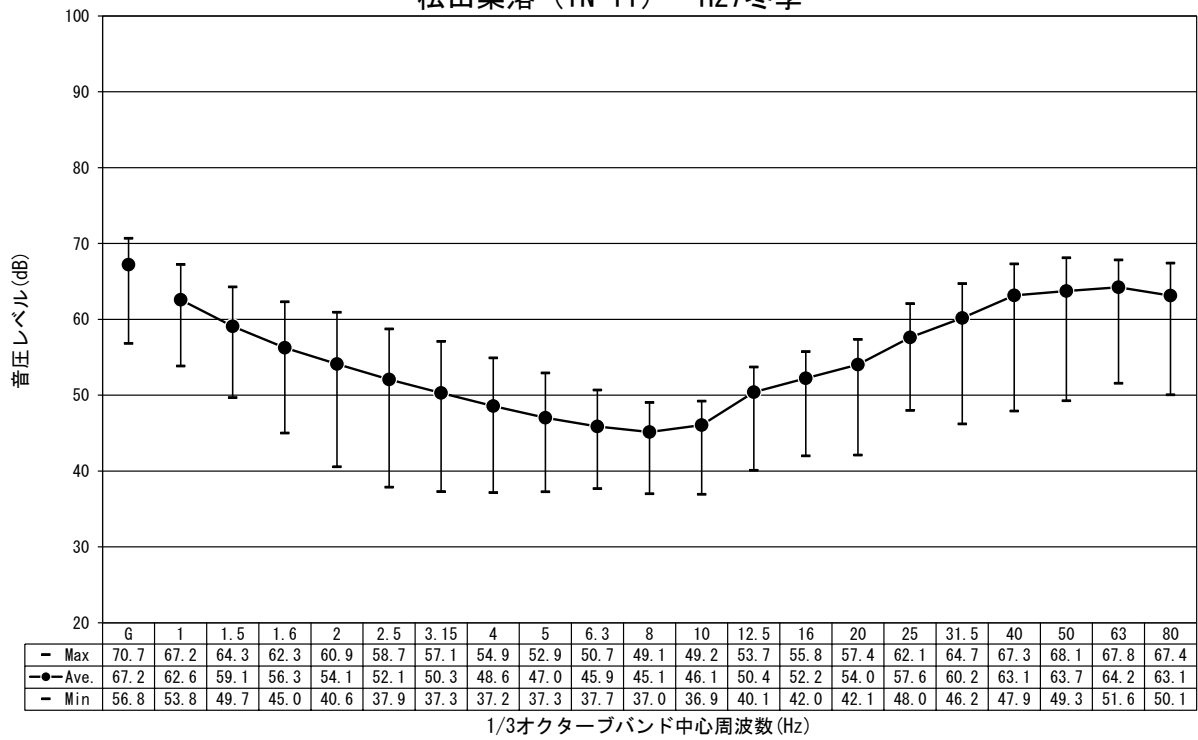
図-2.1.4.12(3) 低周波音の調査結果 (平成 27 年度冬季)
