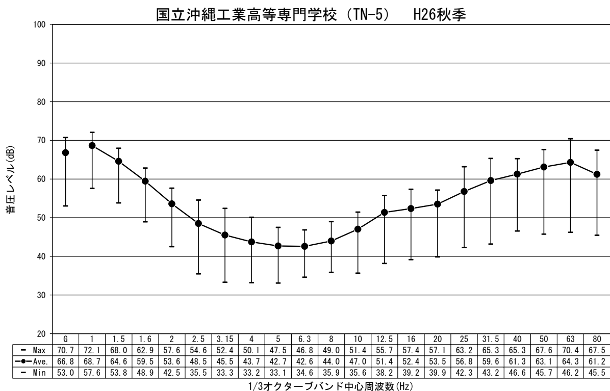
図-2.1.4.7(1) 低周波音の調査結果 (平成26年度秋季)
