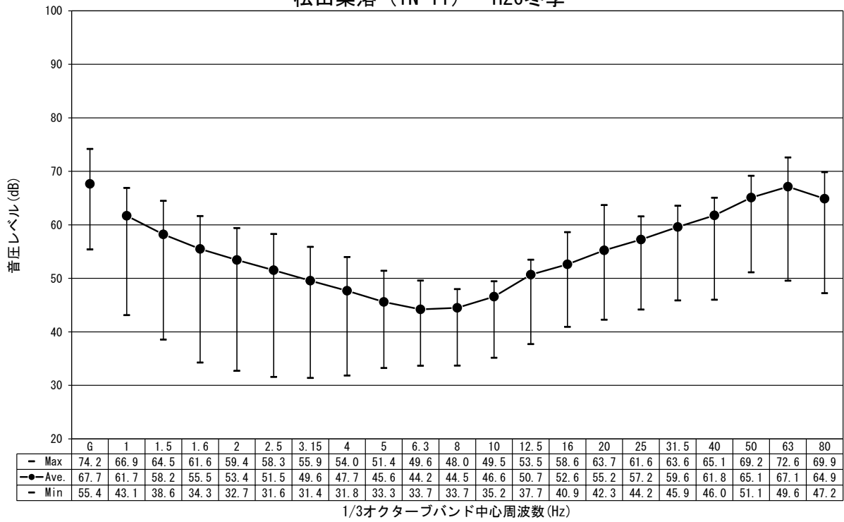
図-2.1.4.8(3) 低周波音の調査結果 (平成 26 年度冬季)
