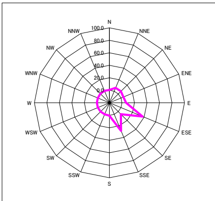
図-2. 1. 1. 13 風向別平均風速、風向別出現頻度 (平成 27 年度秋季)
