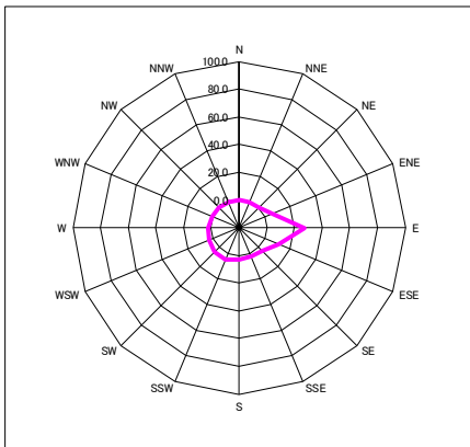
図-2.1.4.15 風向別平均風速、風向別出現頻度(平成26年度冬季)
