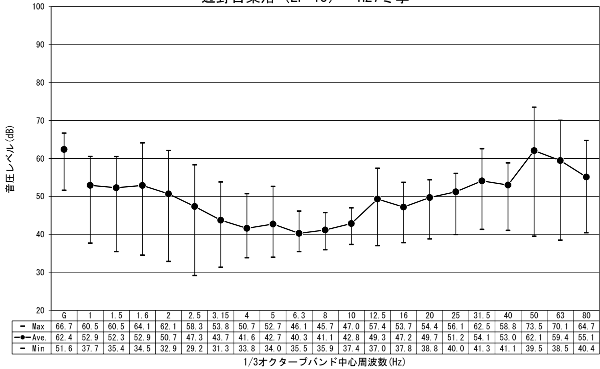
図-2.1.4.4 低周波音の調査結果 (平成 27 年度冬季)
