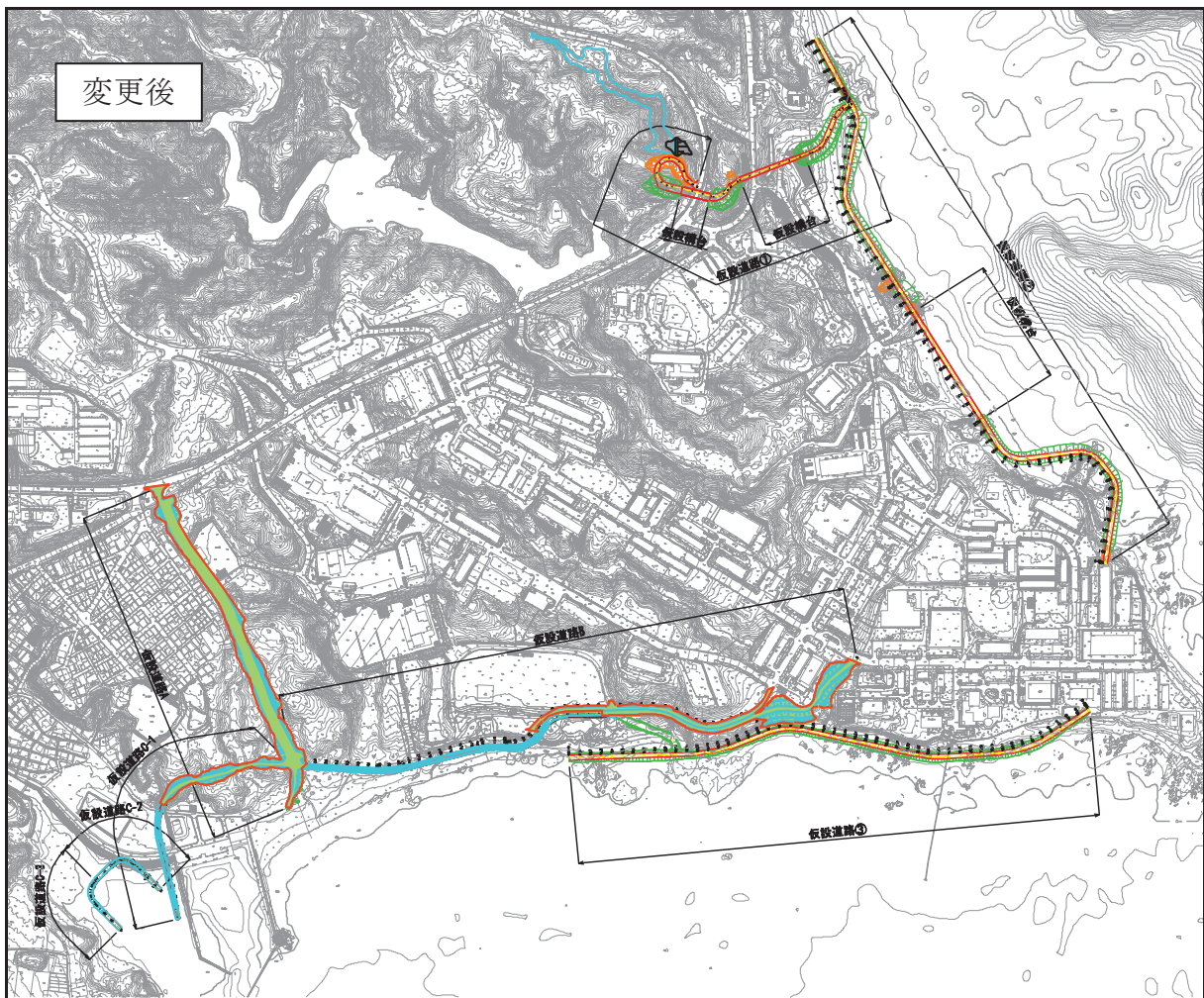
図-2.4.3 工事用仮設道路平面図（上：変更前、下：変更後）
