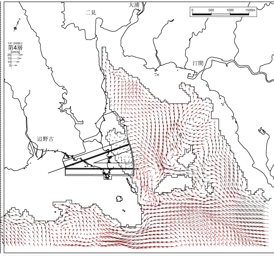
図-6.9.2.3.63(16) 供用時の流速ベクトルの変化
