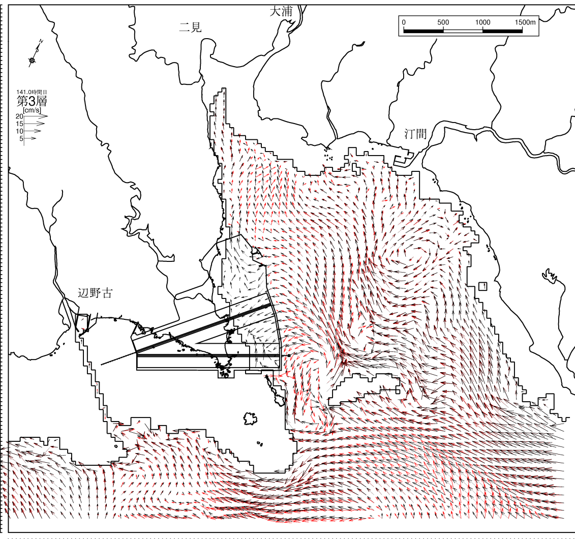
図-6.9.2.3.63(15) 供用時の流速ベクトルの変化
