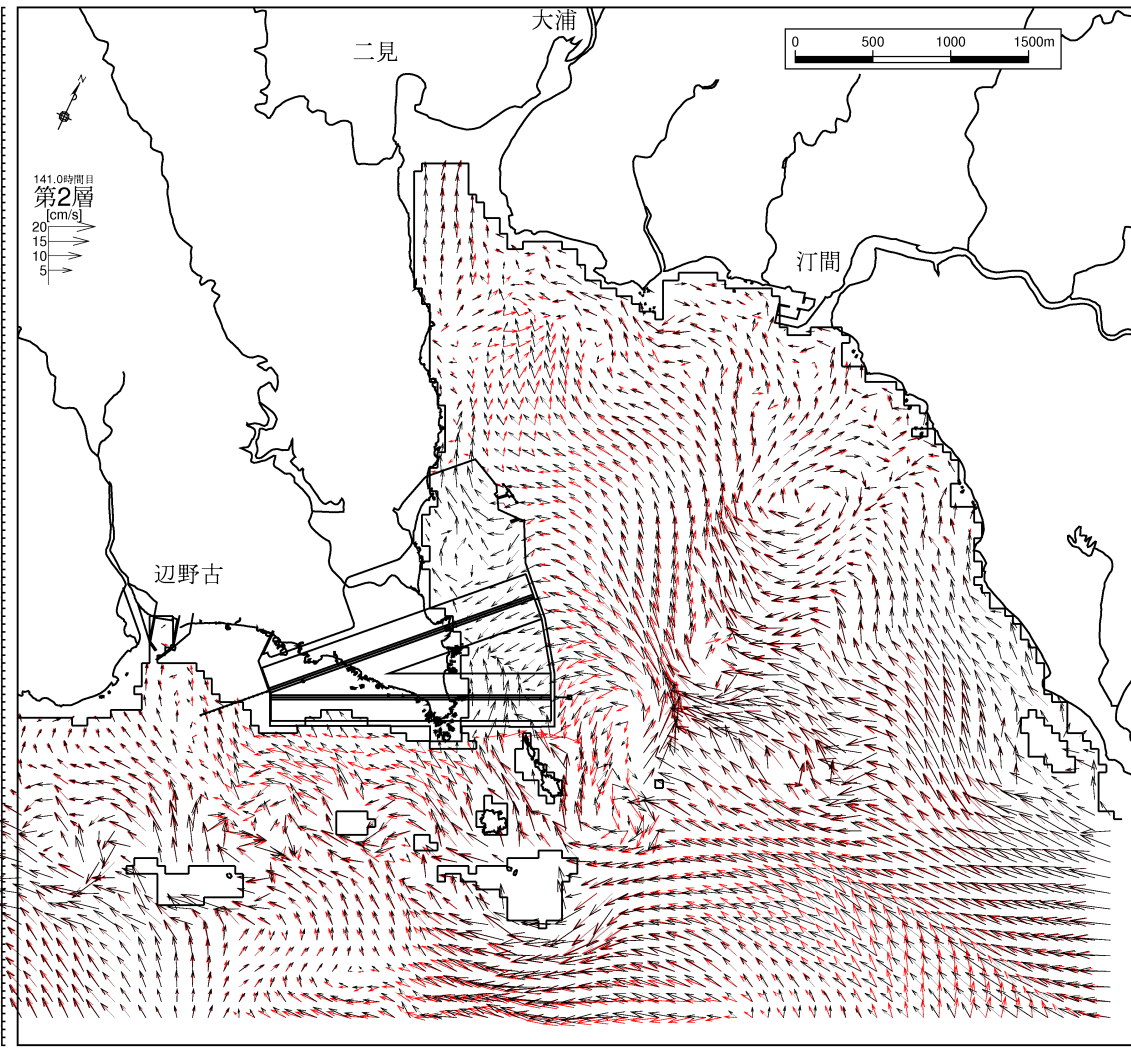
図-6.9.2.3.63(14) 供用時の流速ベクトルの変化
