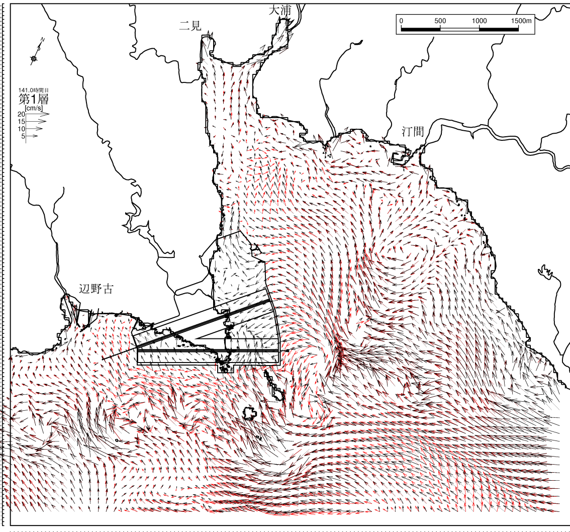
図-6.9.2.3.63(13) 供用時の流速ベクトルの変化
