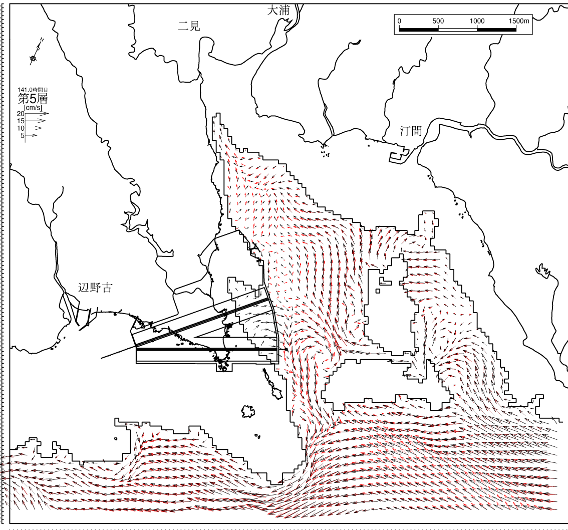
図-6.9.2.3.63(17) 供用時の流速ベクトルの変化
