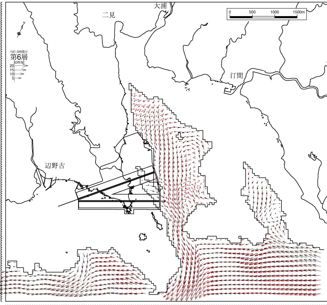
図-6.9.2.3.63(18) 供用時の流速ベクトルの変化
