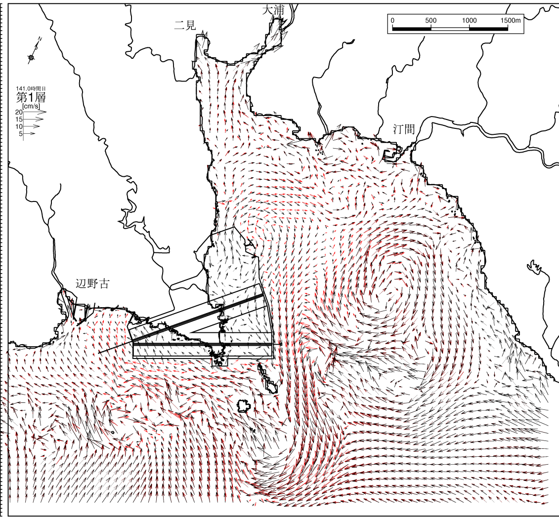
図-6.9.2.3.61(13) 供用時の流速ベクトルの変化
