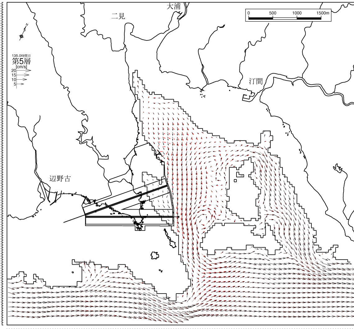
図-6.9.2.3.61(11) 供用時の流速ベクトルの変化
