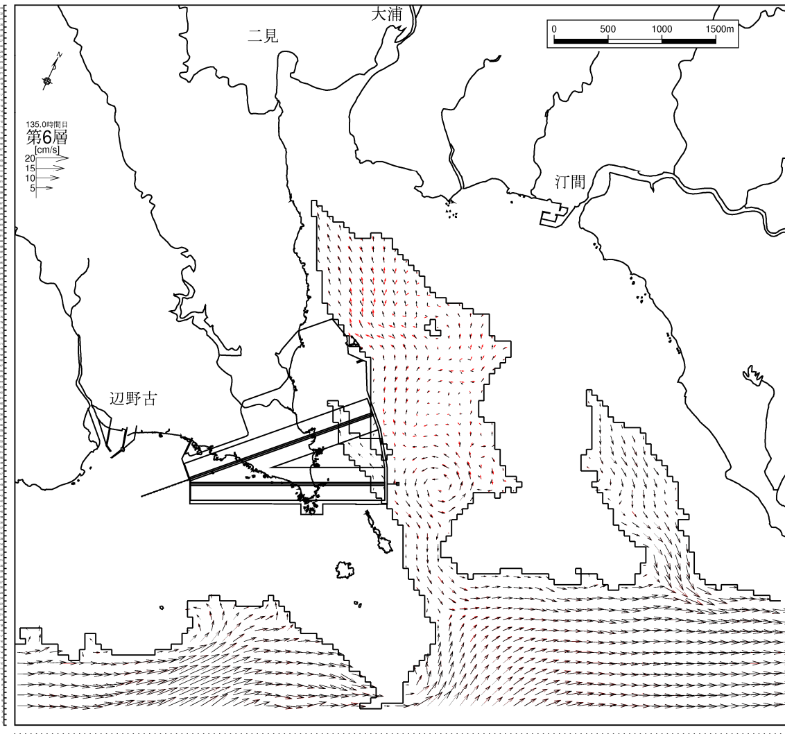
図-6.9.2.3.61(12) 供用時の流速ベクトルの変化
