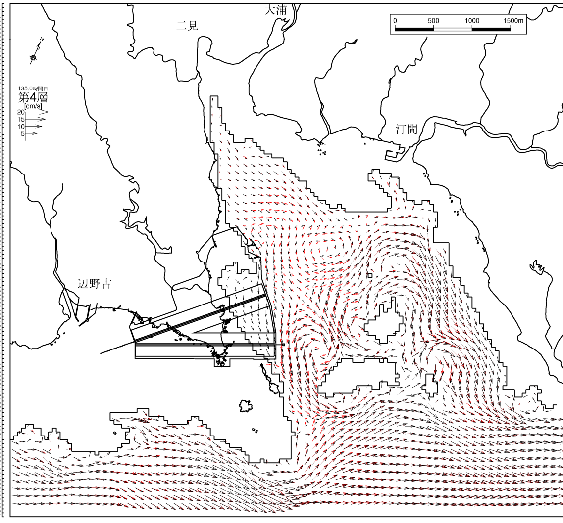
図-6.9.2.3.61(10) 供用時の流速ベクトルの変化
