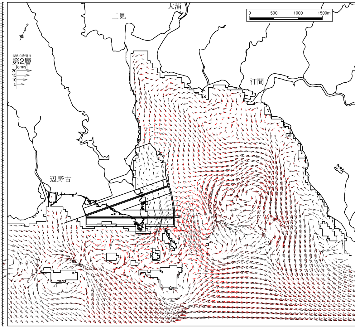
図-6.9.2.3.61(8) 供用時の流速ベクトルの変化
