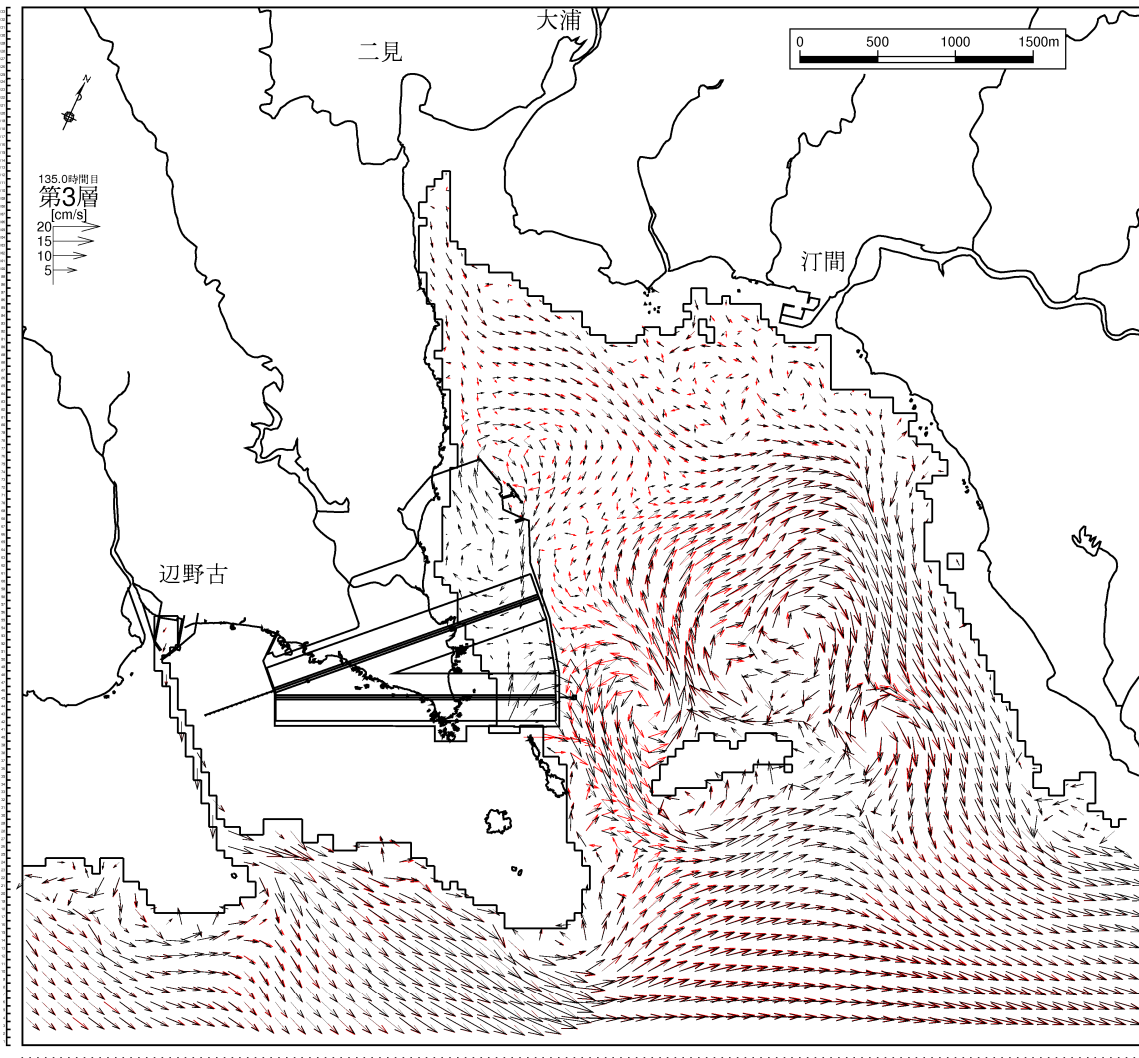
図-6.9.2.3.61(9) 供用時の流速ベクトルの変化
