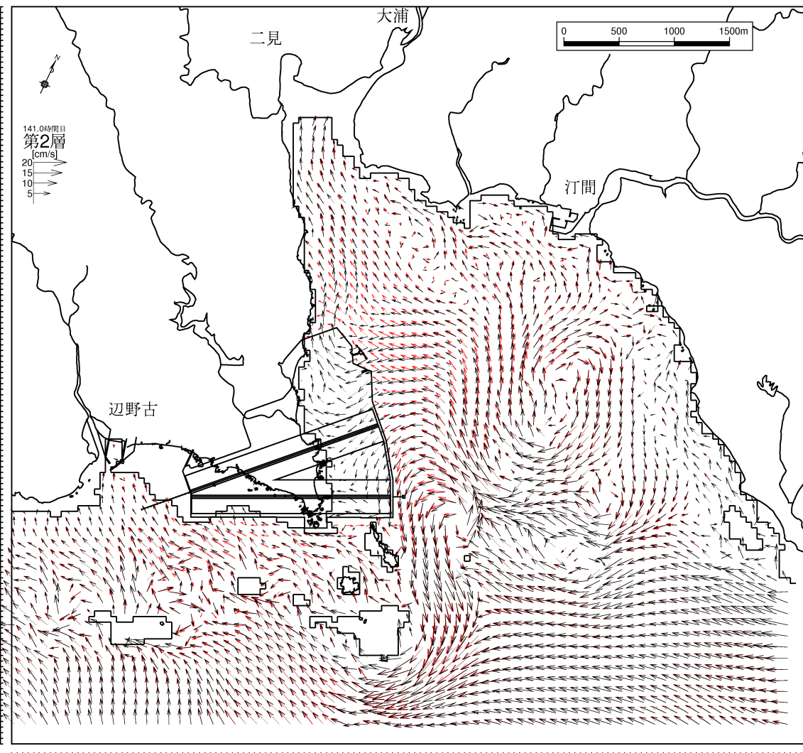
図-6.9.2.3.61(14) 供用時の流速ベクトルの変化
