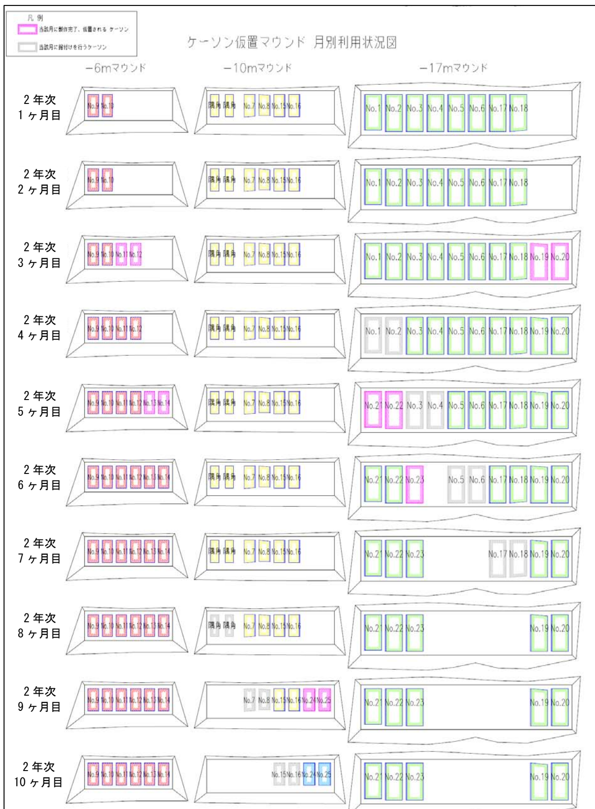
図-2.4.2.47(2) 海上ヤード（ケーソン仮置きマウンド）の月別利用状況図 （2年次1～10ヶ月目）
