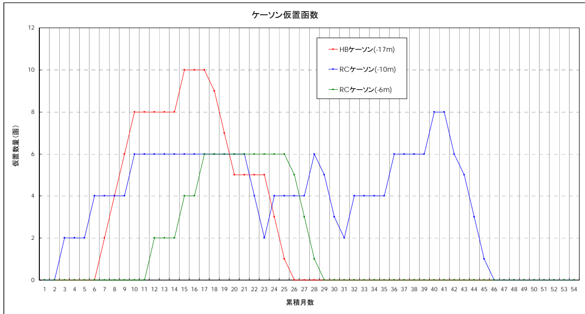
図-2.4.2.49 ケーソン月別仮置函数
