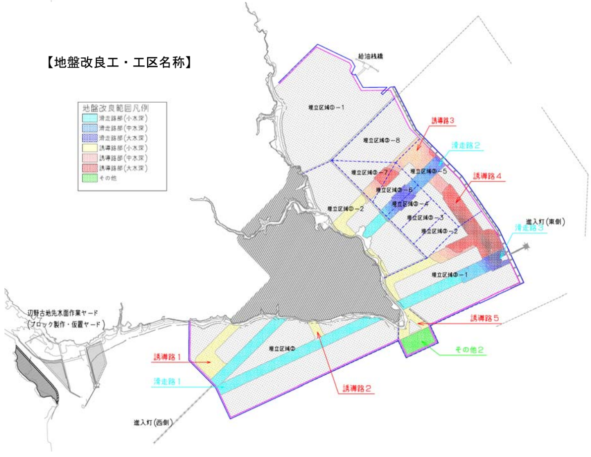
図-2.4.2.20 埋立工・地盤改良工 工区名称
