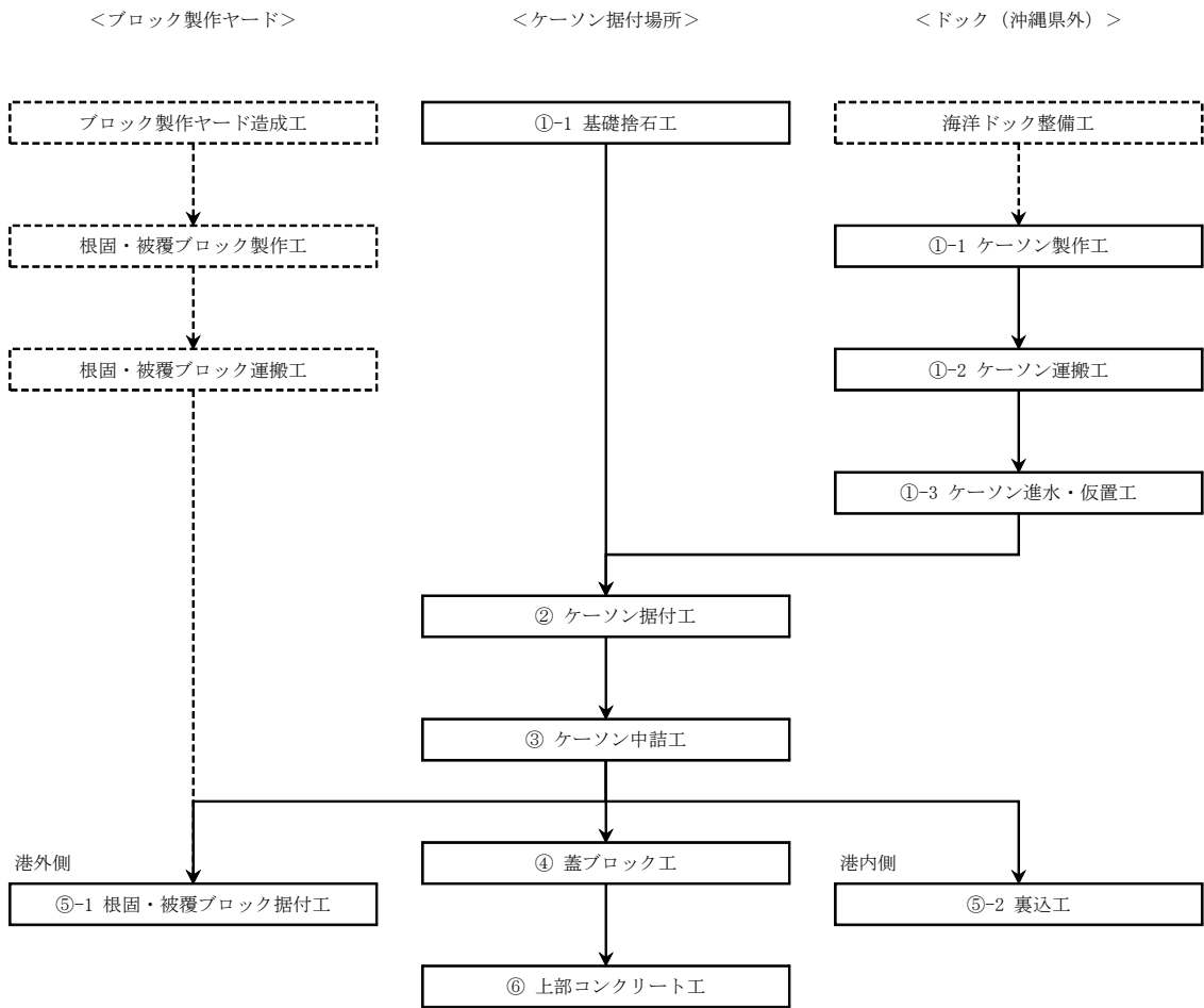
図-2.4.2.9 ケーソン式護岸 施工フロー (ハイブリッドケーソン)
