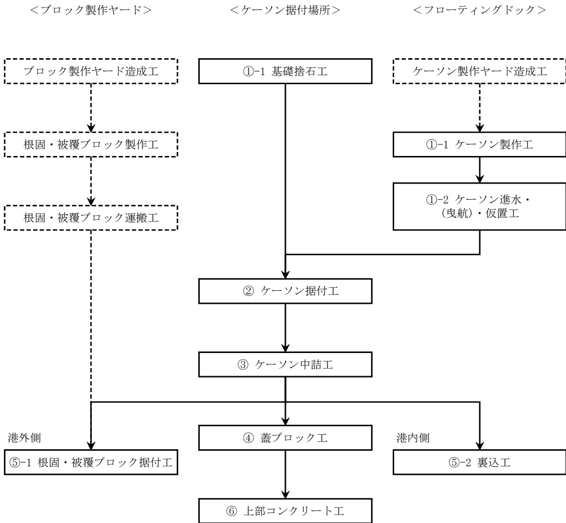
図-2.4.2.8 ケーソン式護岸 施工フロー (RC ケーソン)
