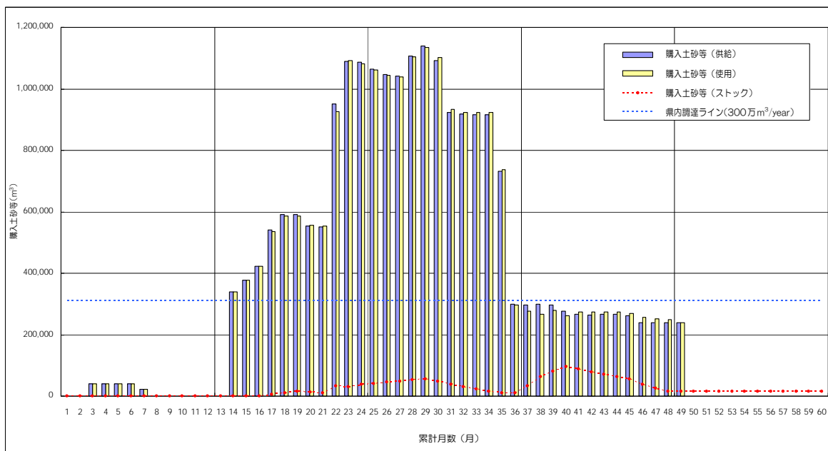
図-2.4.2.39 埋立・地盤改良用土砂（購入土砂等）月別使用・搬入・ストック量
