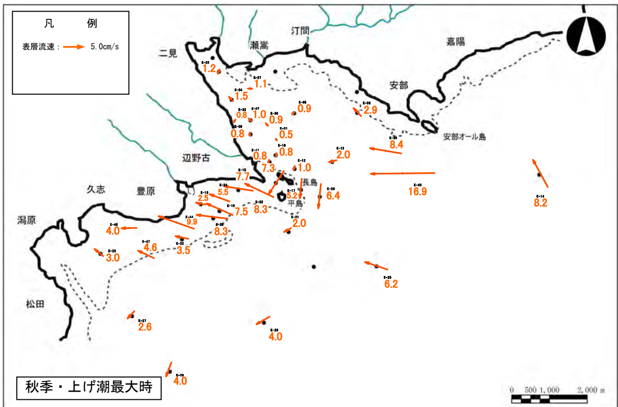
図-6.9.1.5(3) 調和解析結果に基づく表層の平均大潮期流況分布 (平成20年度秋季)
