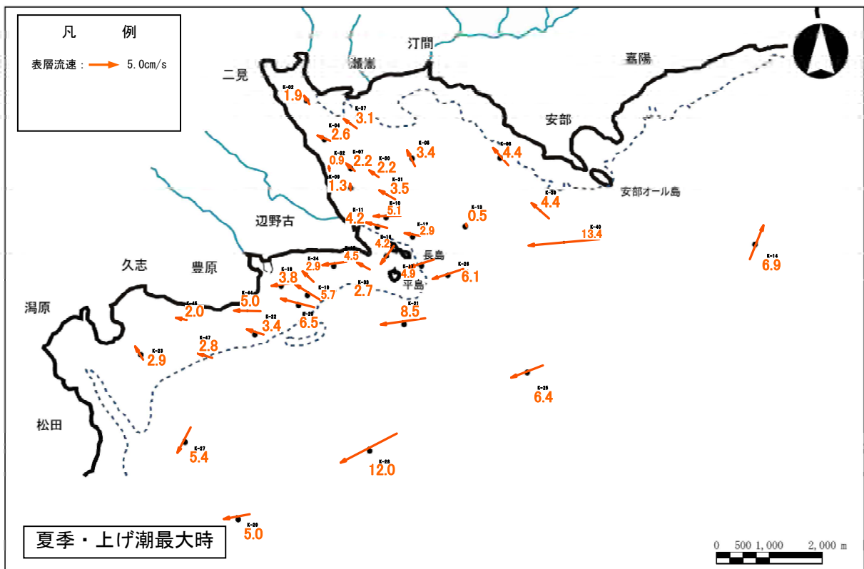
図-6. 9. 1. 5(2) 調和解析結果に基づく表層の平均大潮期流況分布 (平成 20 年度夏季)
