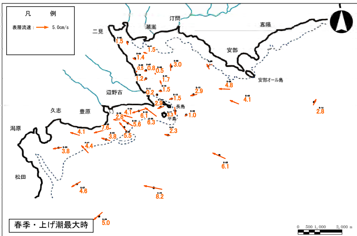
図-6.9.1.5(1) 調和解析結果に基づく表層の平均大潮期流況分布 (平成 20 年度春季)
