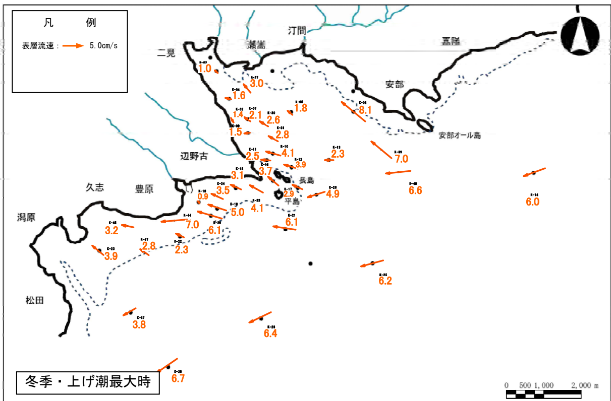
図-6. 9. 1. 5(4) 調和解析結果に基づく表層の平均大潮期流況分布 (平成 20 年度冬季)
