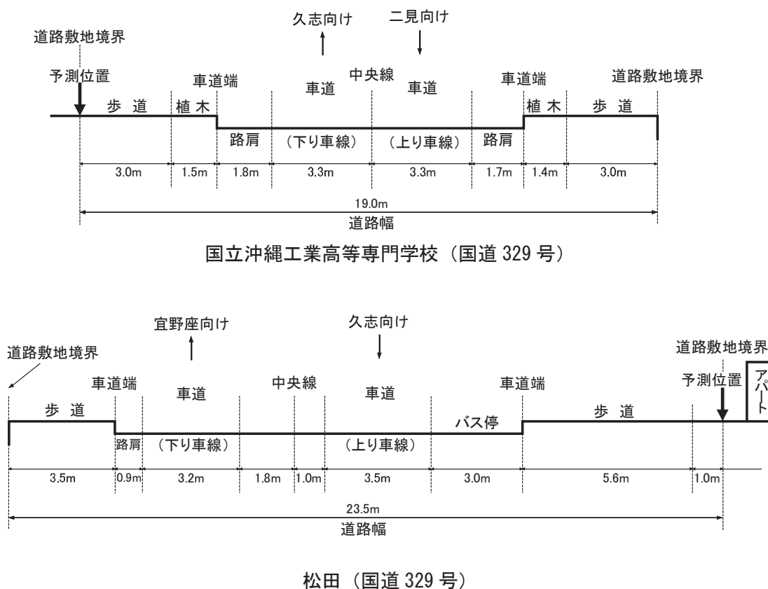
図-6.4.2.2.4 予測地点の道路構造
