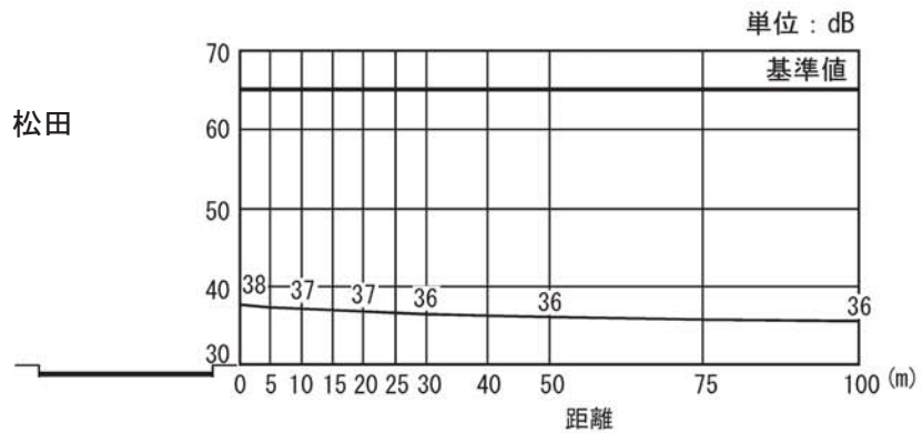
図-6.4.2.1.13 道路交通振動の距離減衰
