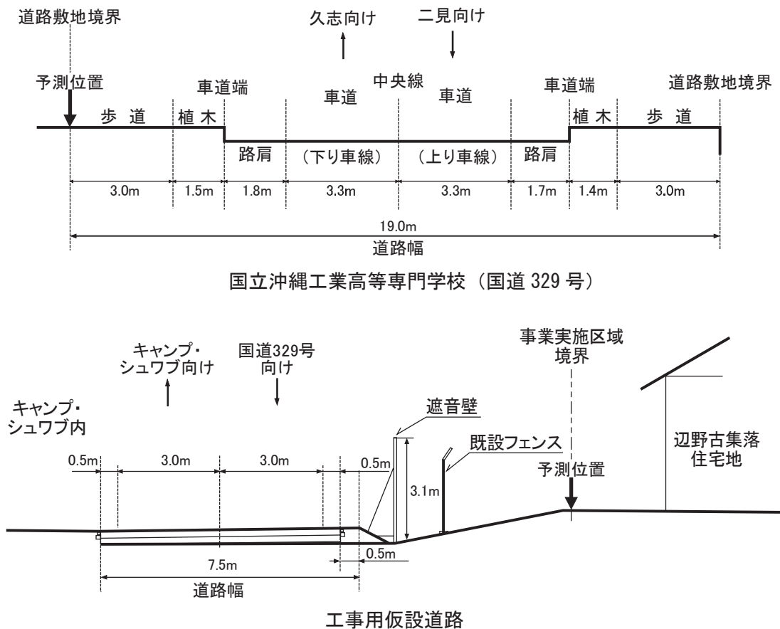
図-6.4.2.1.9 予測地点の道路構造
