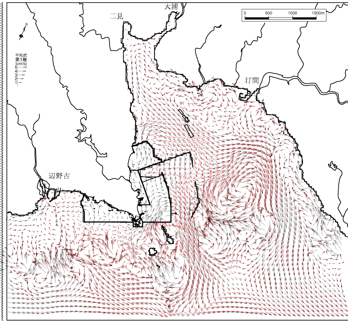
図-6.9.2.1.15(13) 4年次4ヶ月目の流速ベクトルの変化(夏季) 第1層[0~2m]、恒流(平均流)
