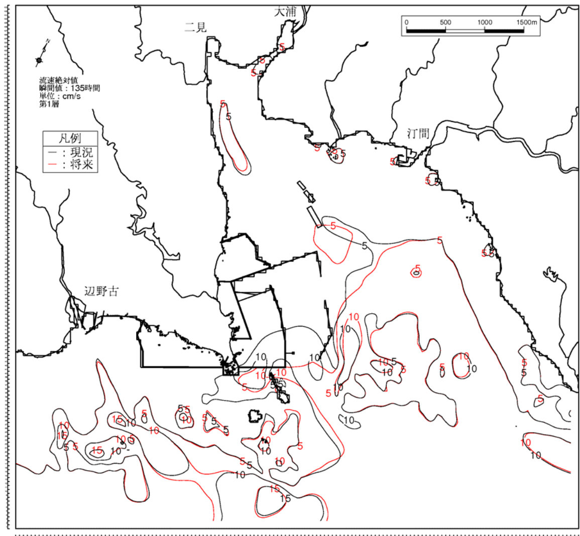
図-6.9.2.1.16(1) 4年次4ヶ月目の流速分布の変化(夏季) 第1層[0~2m]、下げ潮時
