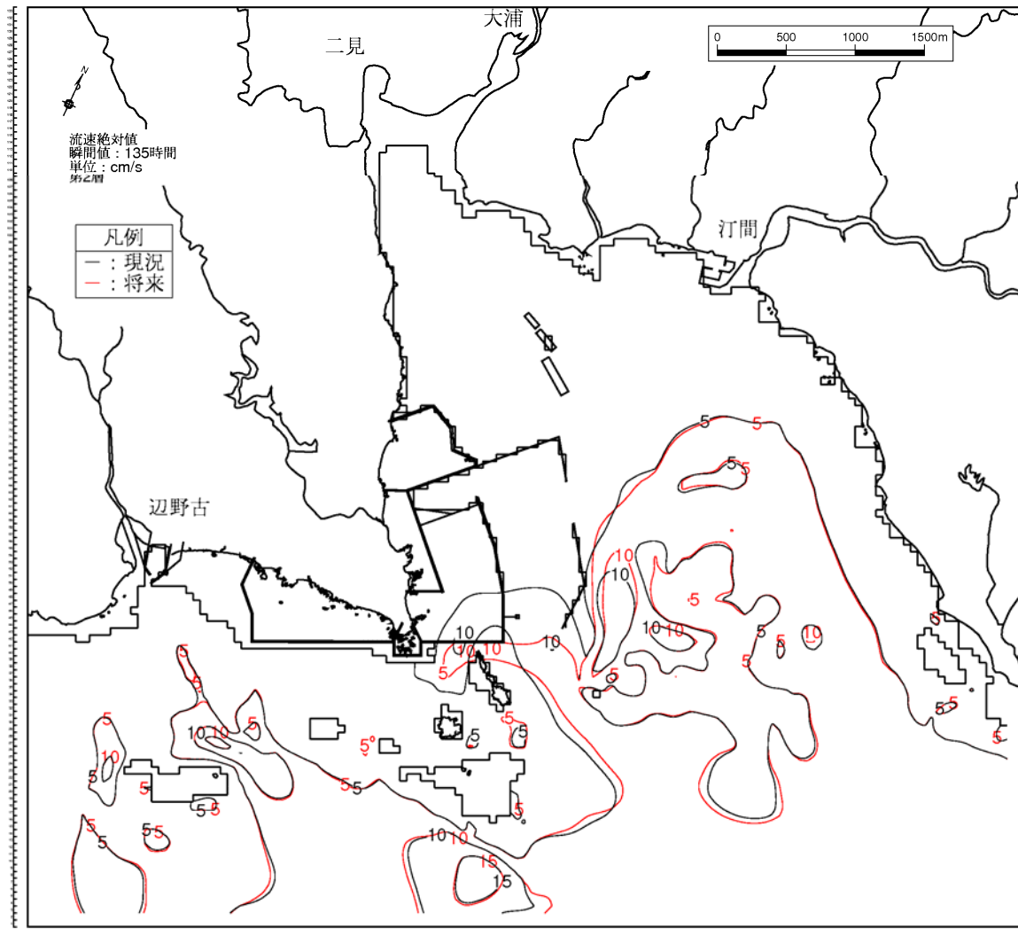
図-6.9.2.1.16(2) 4年次4ヶ月目の流速分布の変化(夏季) 第2層[2~4m]、下げ潮時
