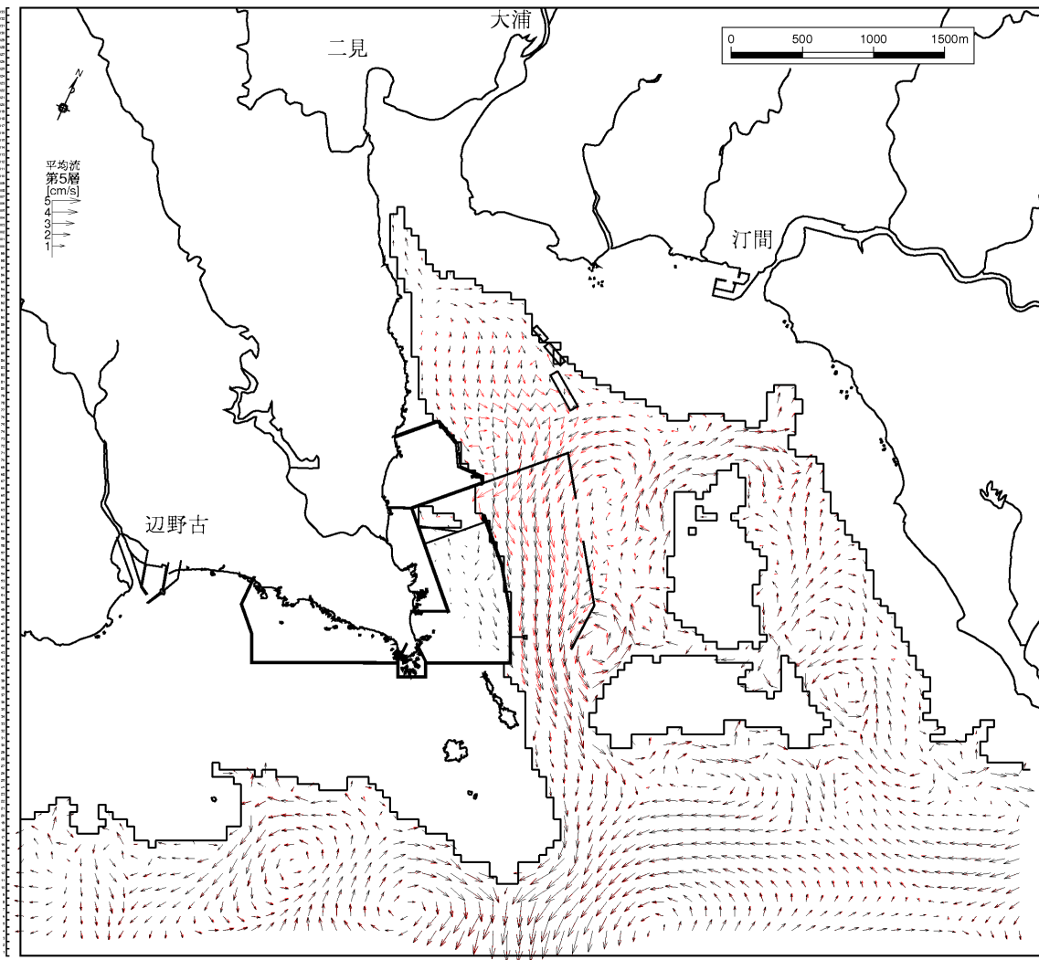
図-6.9.2.1.15(17) 4年次4ヶ月目の流速ベクトルの変化(夏季) 第5層[10~20m]、恒流(平均流)
