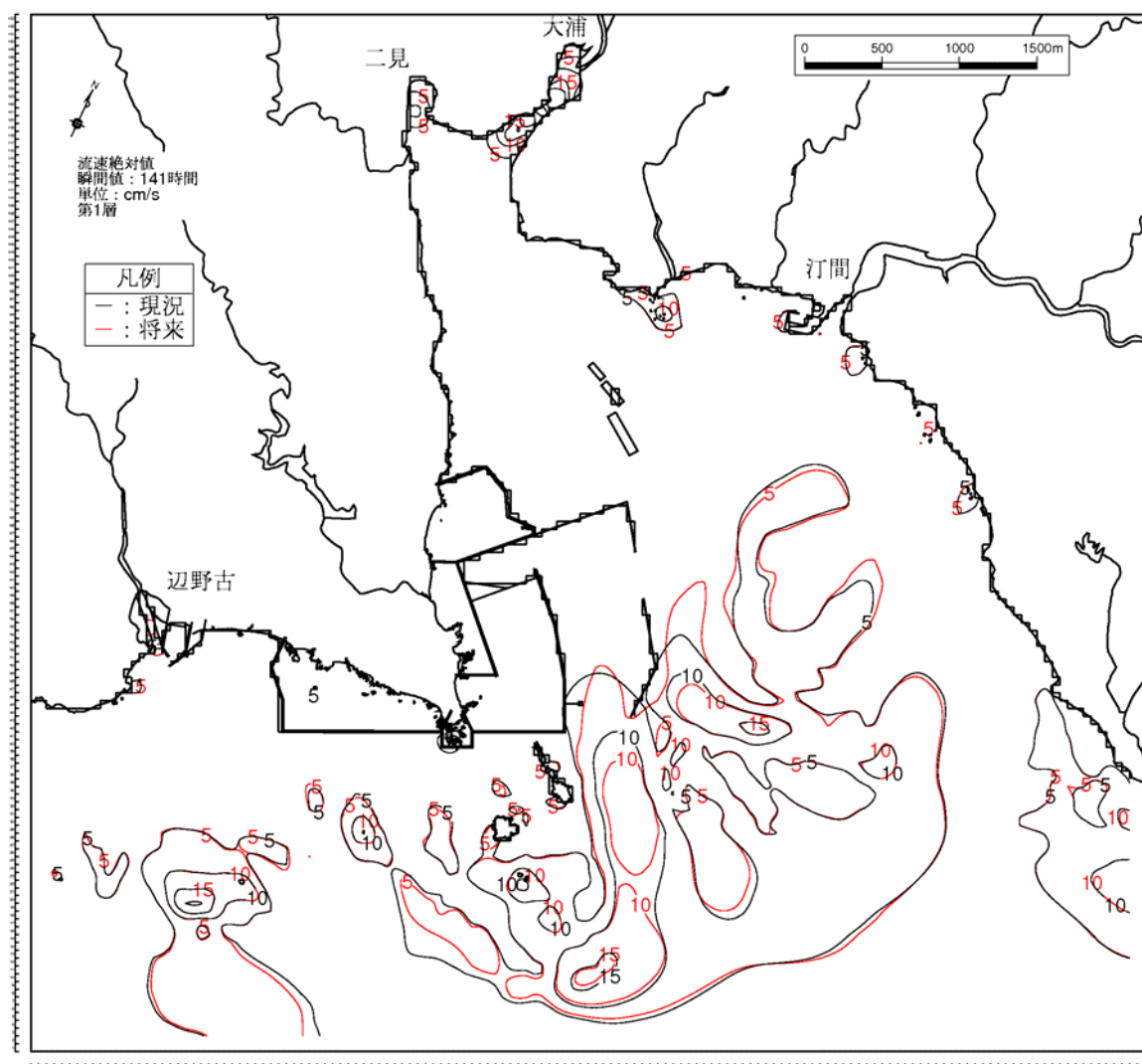
図-6.9.2.1.16(7) 4年次4ヶ月目の流速分布の変化(夏季) 第1層[0~2m]、上げ潮時
