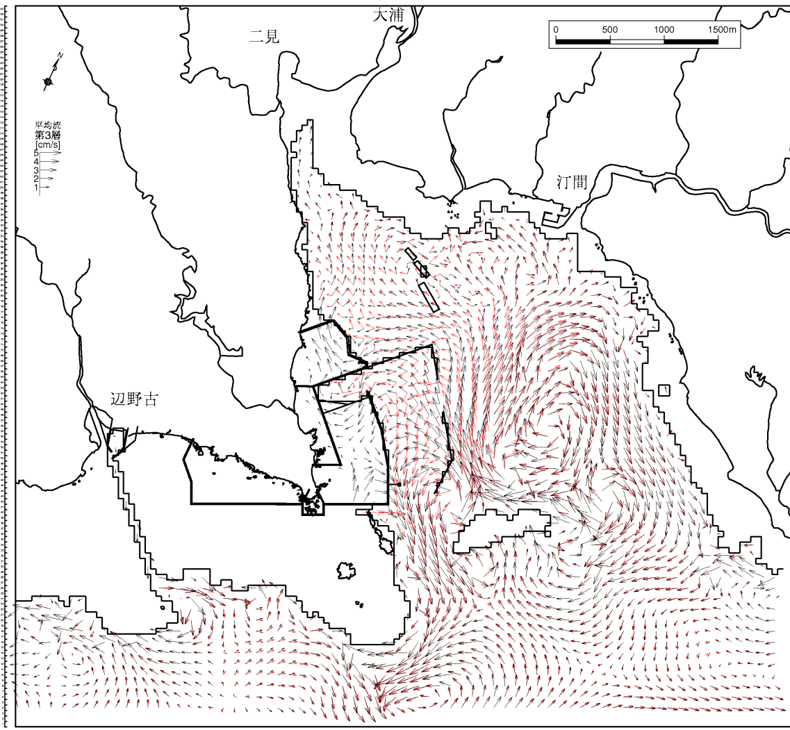
図-6.9.2.1.15(15) 4年次4ヶ月目の流速ベクトルの変化(夏季) 第3層[4~6m]、恒流(平均流)
