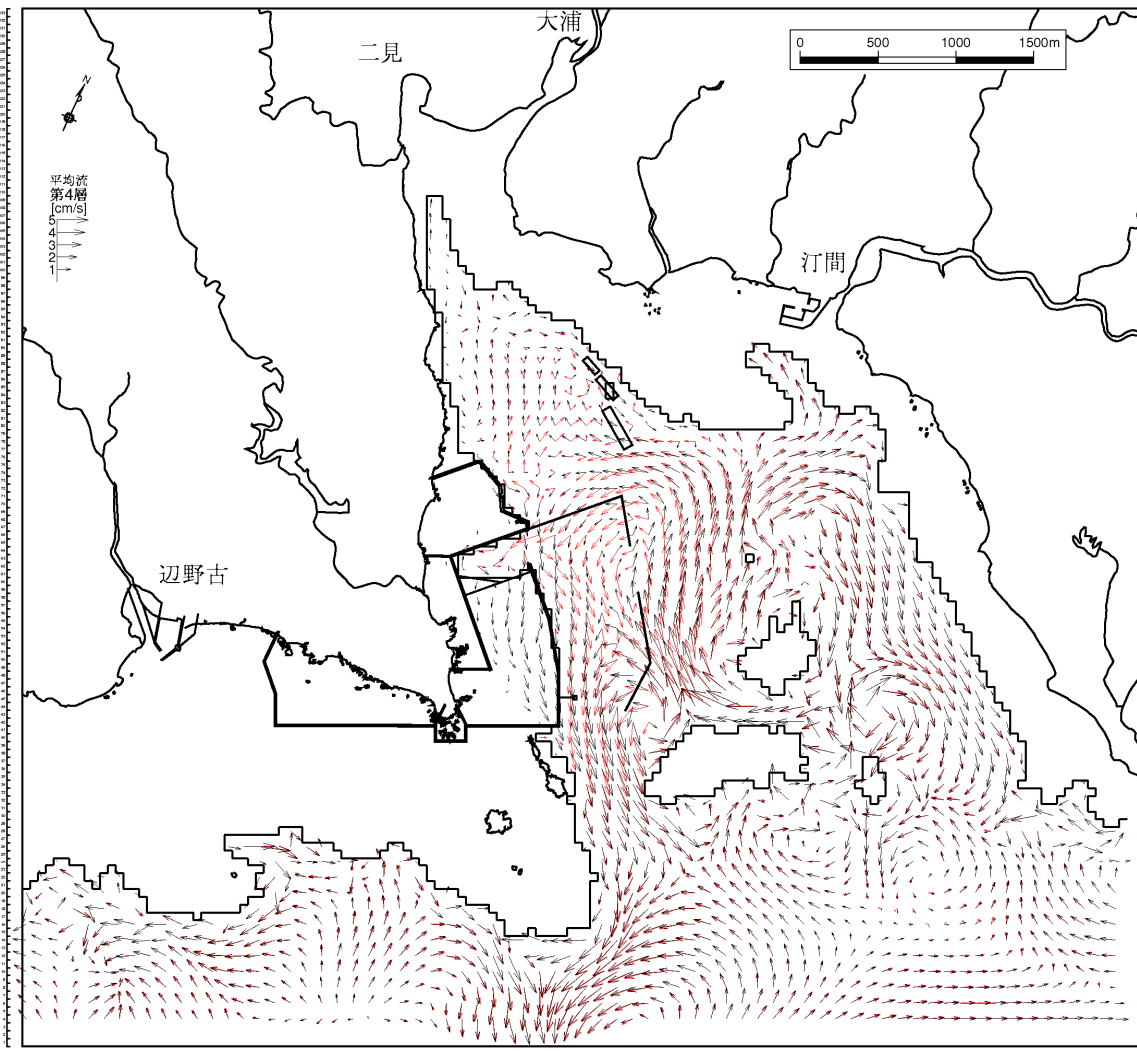
図-6.9.2.1.15(16) 4年次4ヶ月目の流速ベクトルの変化(夏季) 第4層[6~10m]、恒流(平均流)
