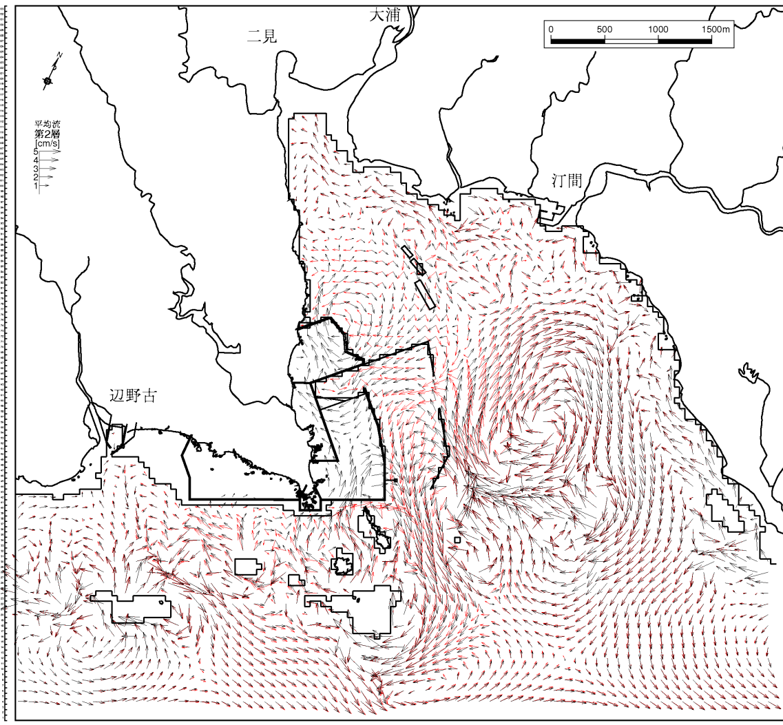
図-6.9.2.1.15(14) 4年次4ヶ月目の流速ベクトルの変化(夏季) 第2層[2~4m]、恒流(平均流)
