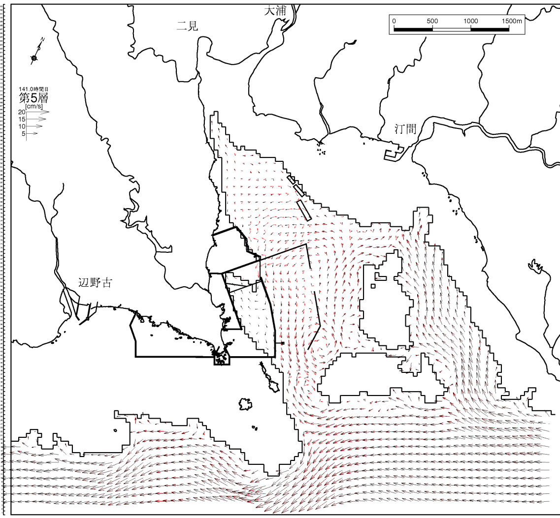
図-6.9.2.1.15(11) 4年次4ヶ月目の流速ベクトルの変化(夏季) 第5層[10~20m]、上げ潮時
