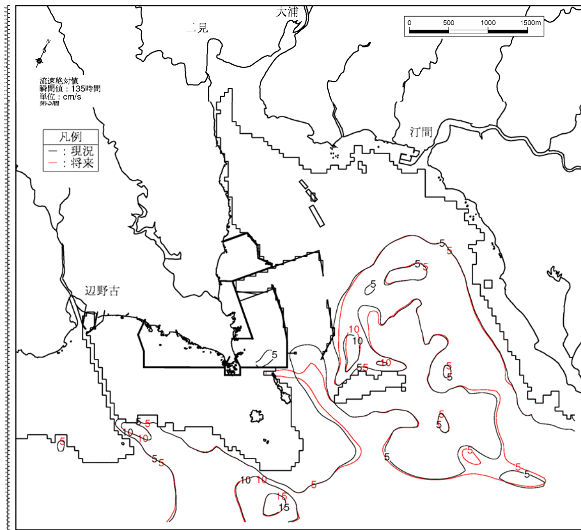
図-6.9.2.1.16(3) 4年次4ヶ月目の流速分布の変化(夏季) 第3層[4~6m]、下げ潮時
