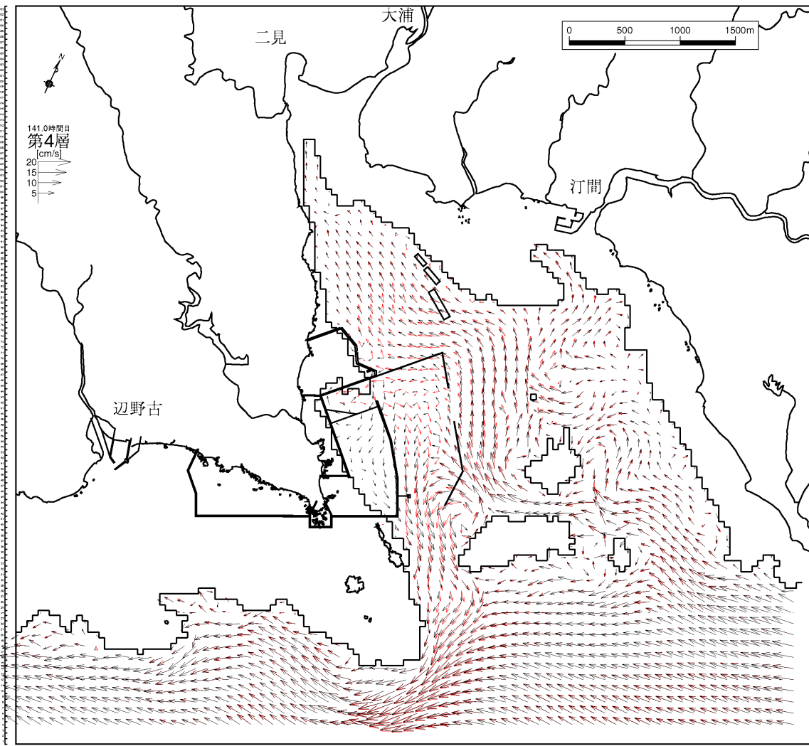
図-6.9.2.1.15(10) 4年次4ヶ月目の流速ベクトルの変化(夏季) 第4層[6~10m]、上げ潮時
