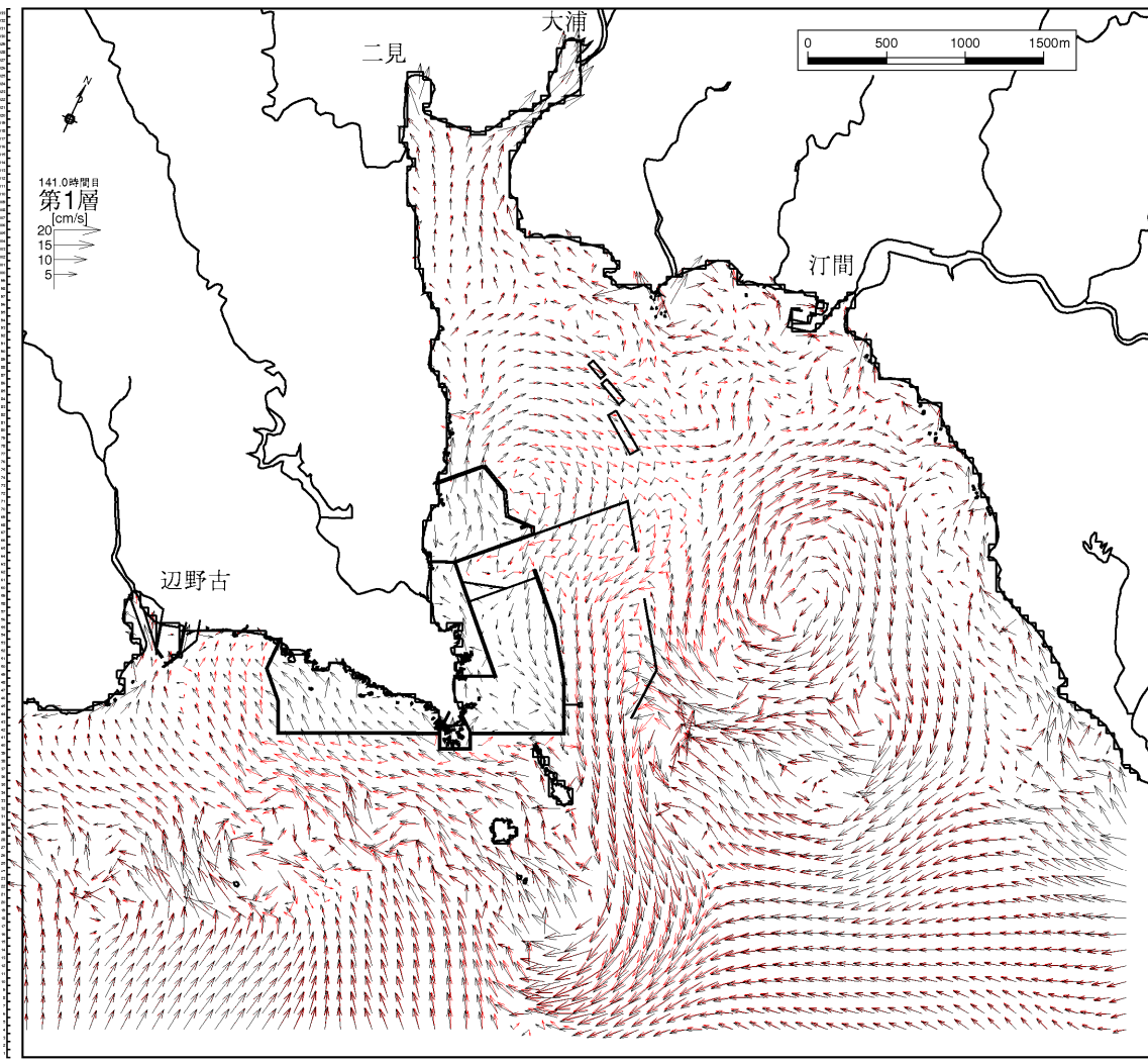
図-6.9.2.1.15(7) 4年次4ヶ月目の流速ベクトルの変化(夏季) 第1層[0~2m]、上げ潮時
