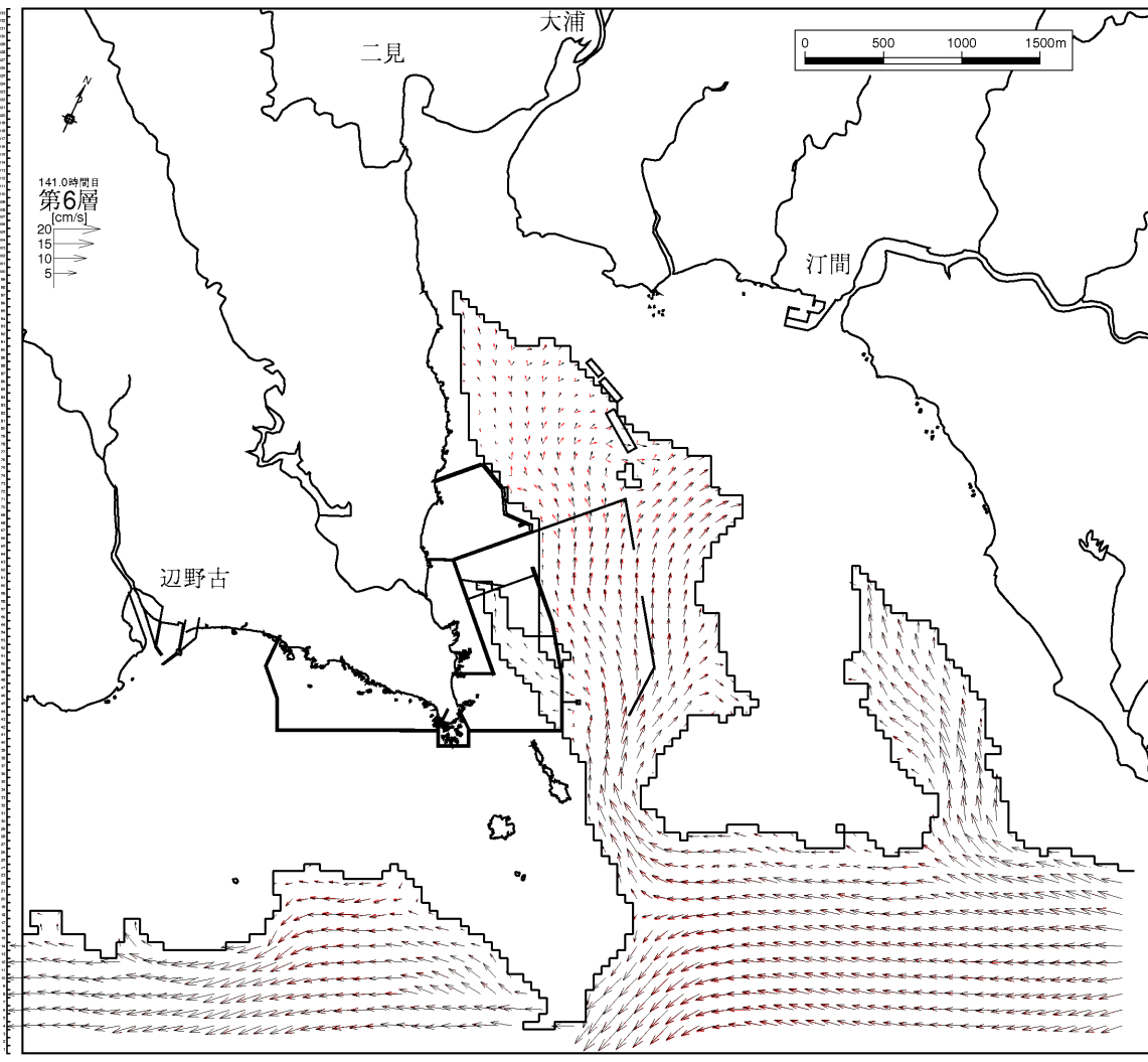
図-6.9.2.1.15(12) 4年次4ヶ月目の流速ベクトルの変化(夏季) 第6層[20m以深]、上げ潮時
