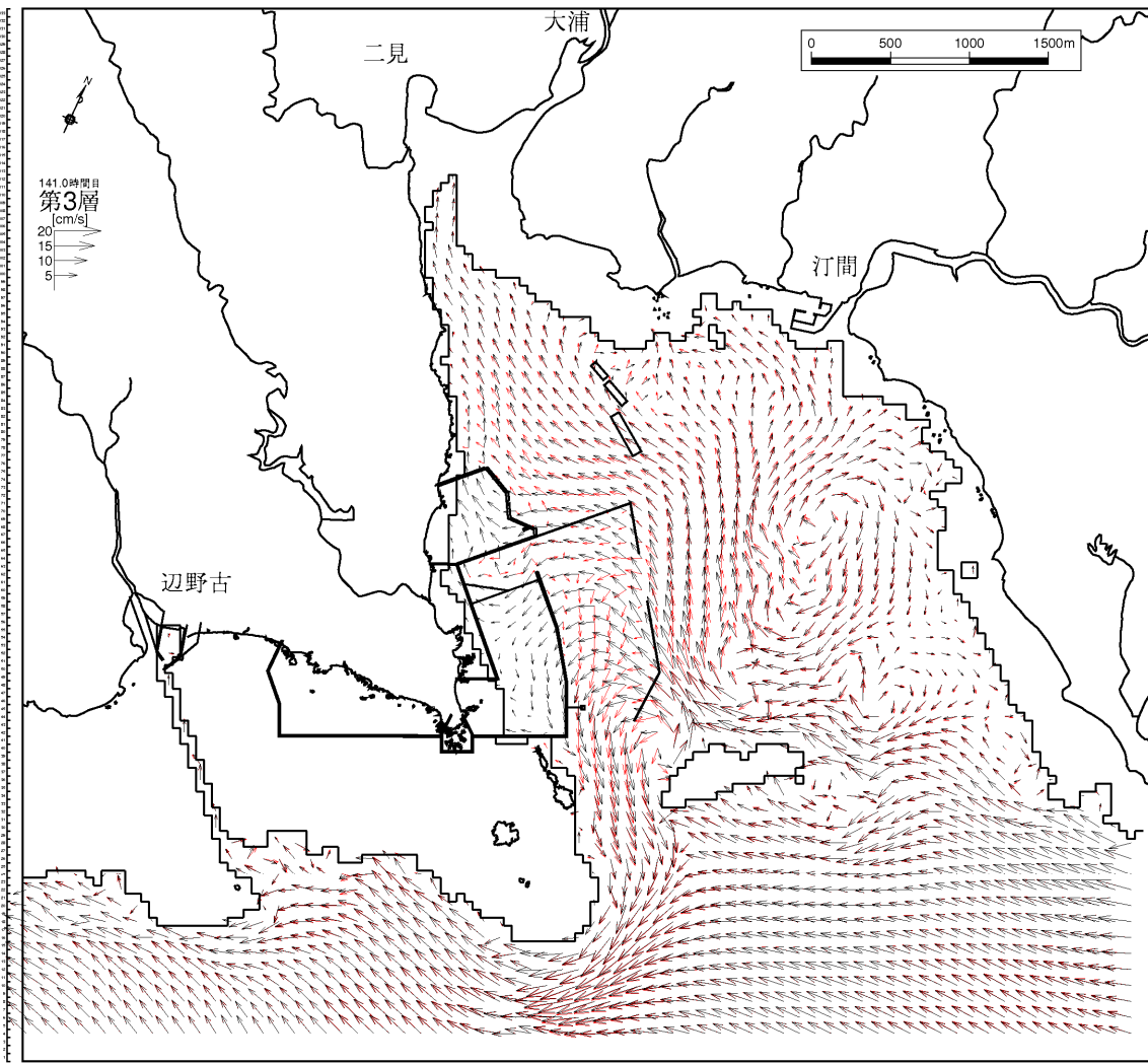
図-6.9.2.1.15(9) 4年次4ヶ月目の流速ベクトルの変化(夏季) 第3層[4~6m]、上げ潮時
