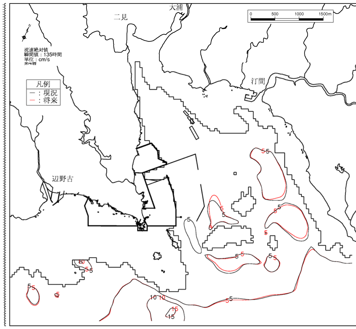
図-6.9.2.1.16(4) 4年次4ヶ月目の流速分布の変化(夏季) 第4層[6~10m]、下げ潮時
