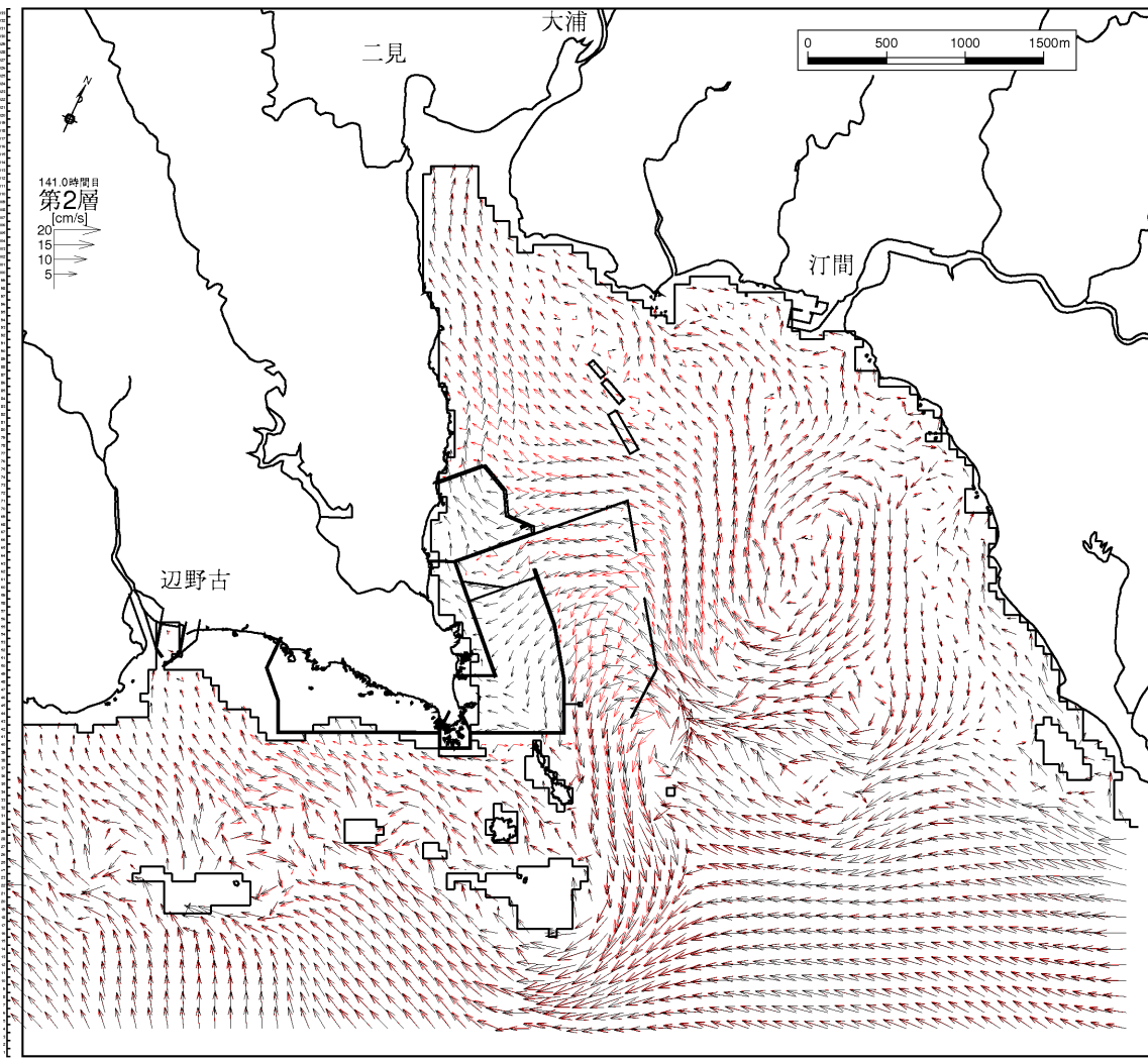
図-6.9.2.1.15(8) 4年次4ヶ月目の流速ベクトルの変化(夏季) 第2層[2~4m]、上げ潮時
