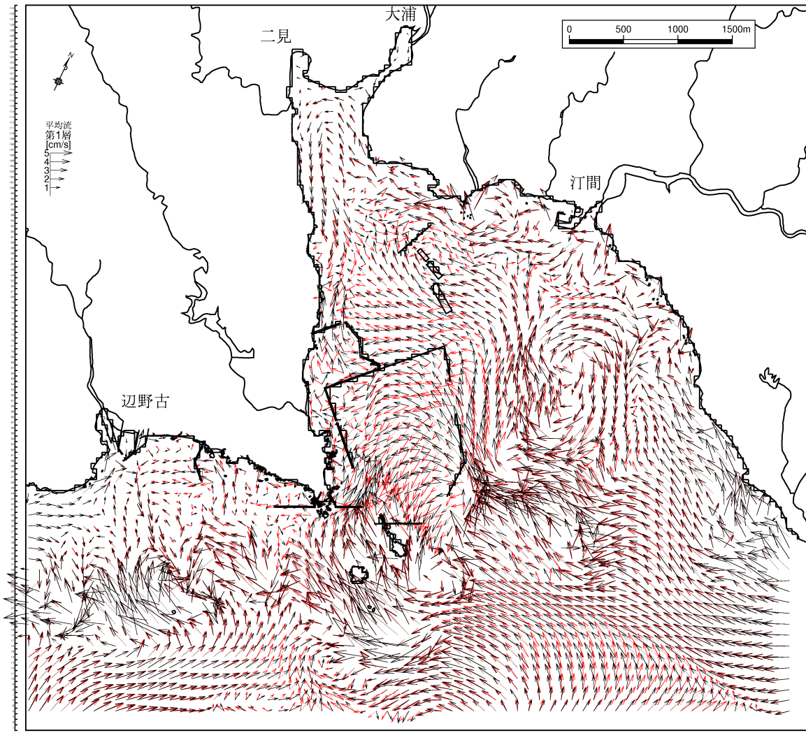
図-6.9.2.1.7(1) 1年次10ヶ月目の流速ベクトルの変化(冬季、全展張)
