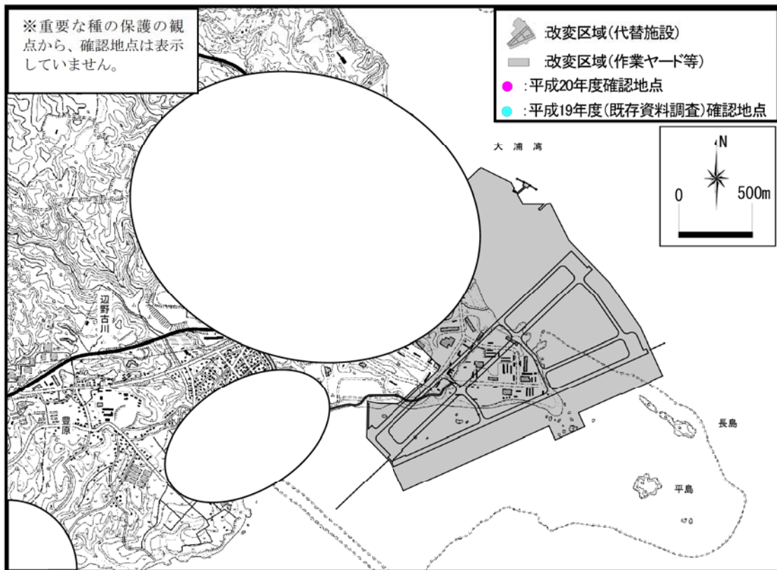
リュウキュウウチキゴキブリの確認地点
