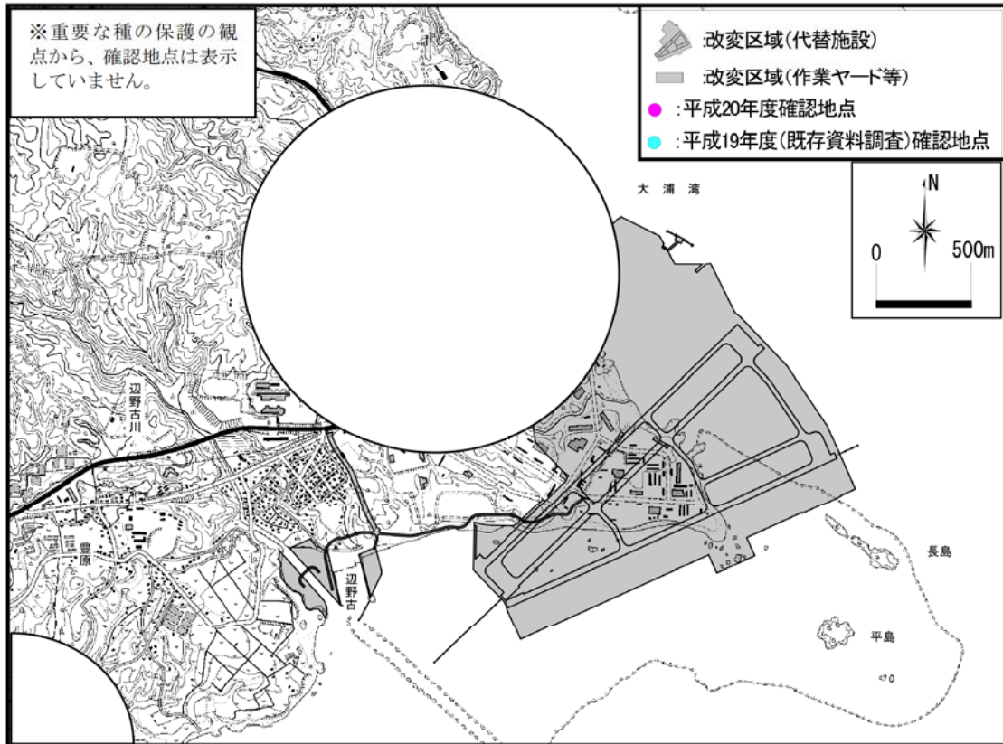
マダラゴキブリの確認地点
