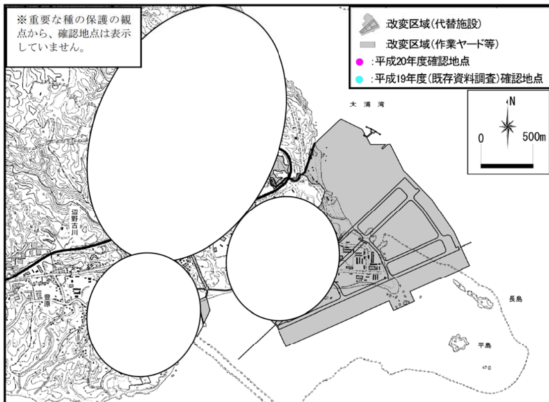
ハロウエルアマガエルの確認地点
