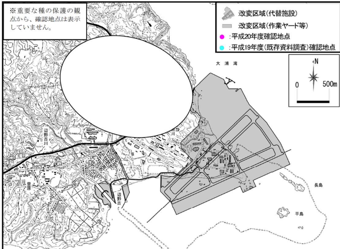
オニヤンマの確認地点
