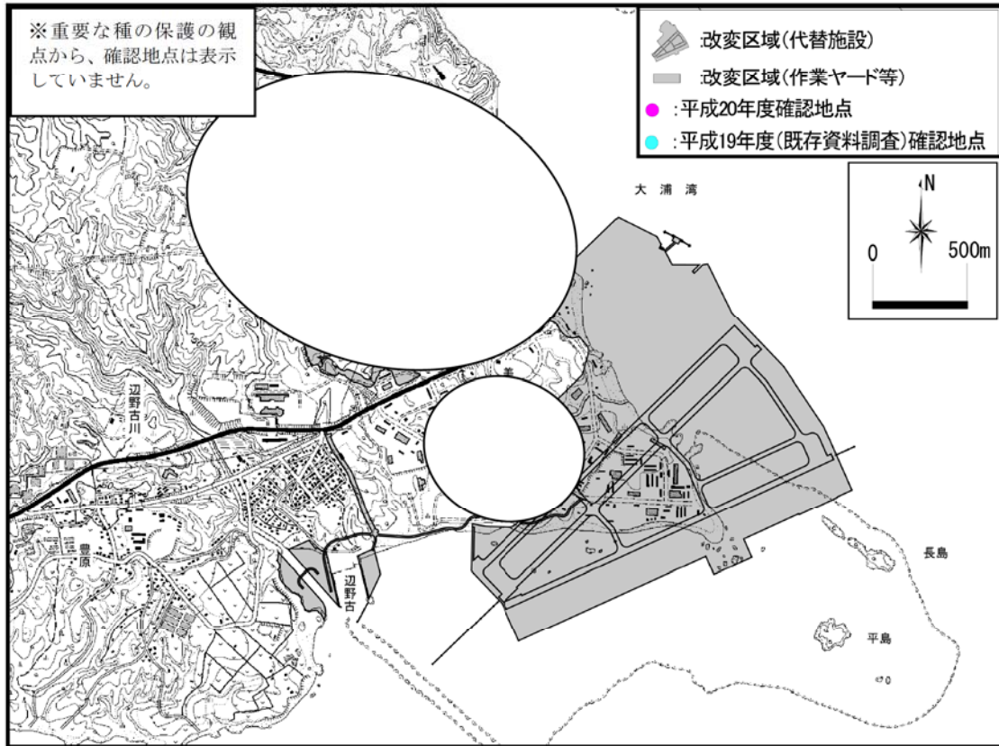
リュウキュウトンボの確認地点
