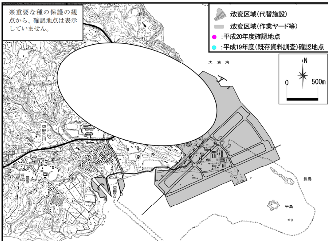
オキナワサラサヤマの確認地点
