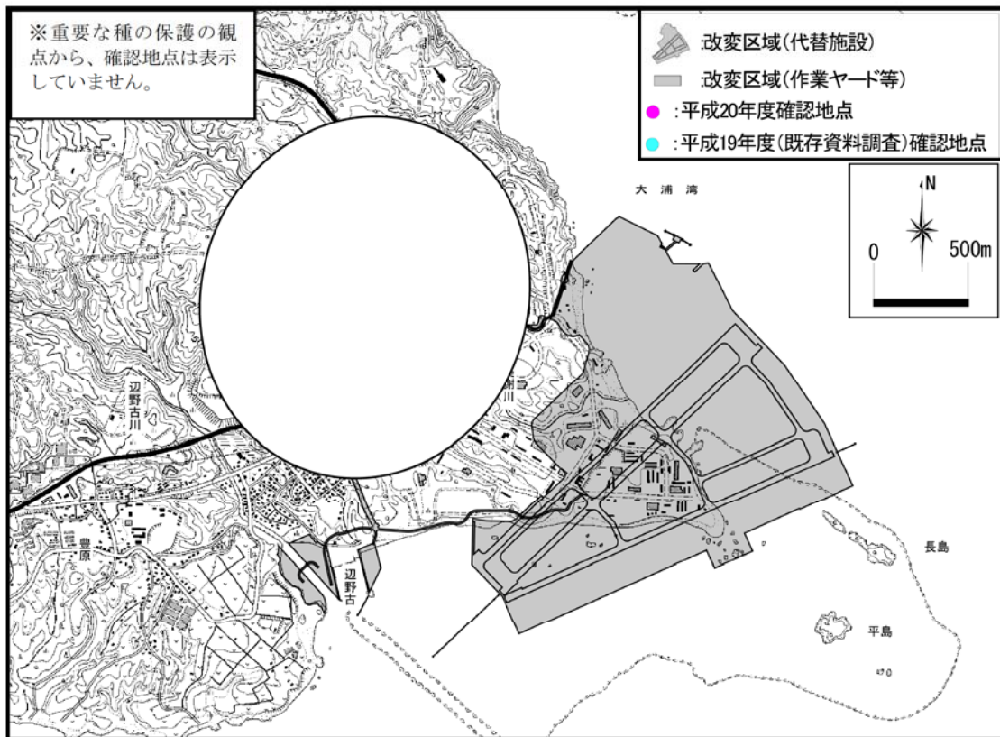
ズングリウマの確認地点
