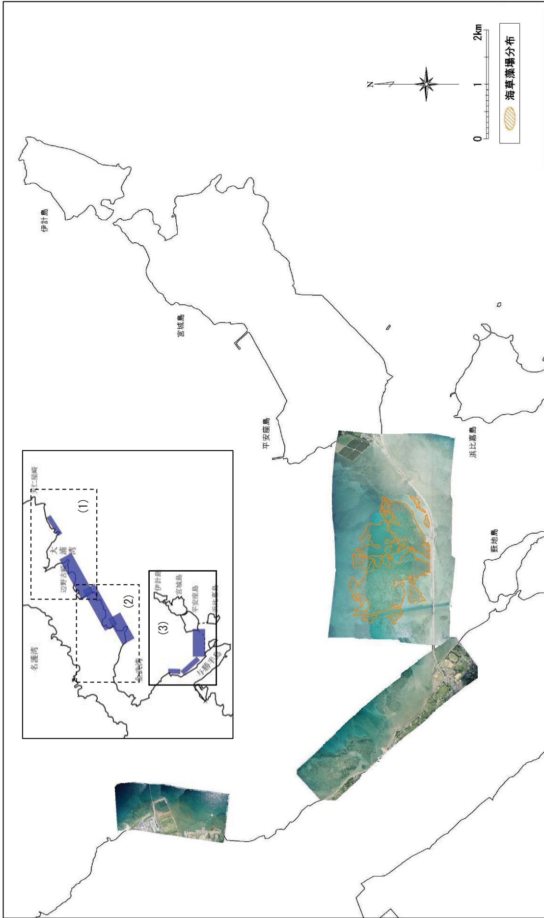
図-6.16.1.27(3) 航空写真に基づく海藻藻場の分布状況（平成19年10月10～12日撮影、(3)）
