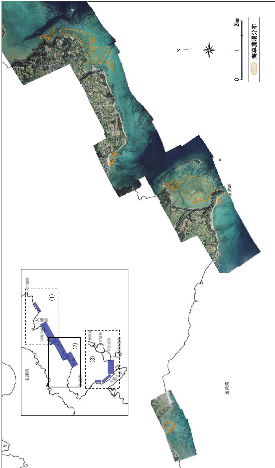
図-6.16.1.27(2) 航空写真に基づく海草藻場の分布状況（平成19年10月10～12日撮影、(2)）
