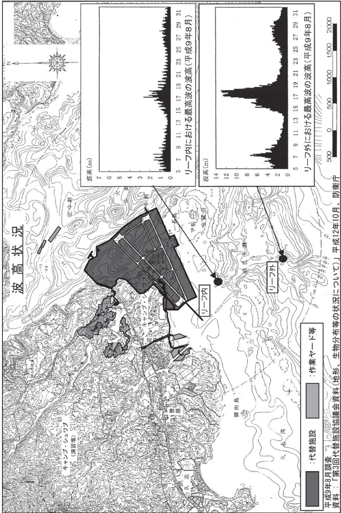
図-3.1.2.2 波高状況
