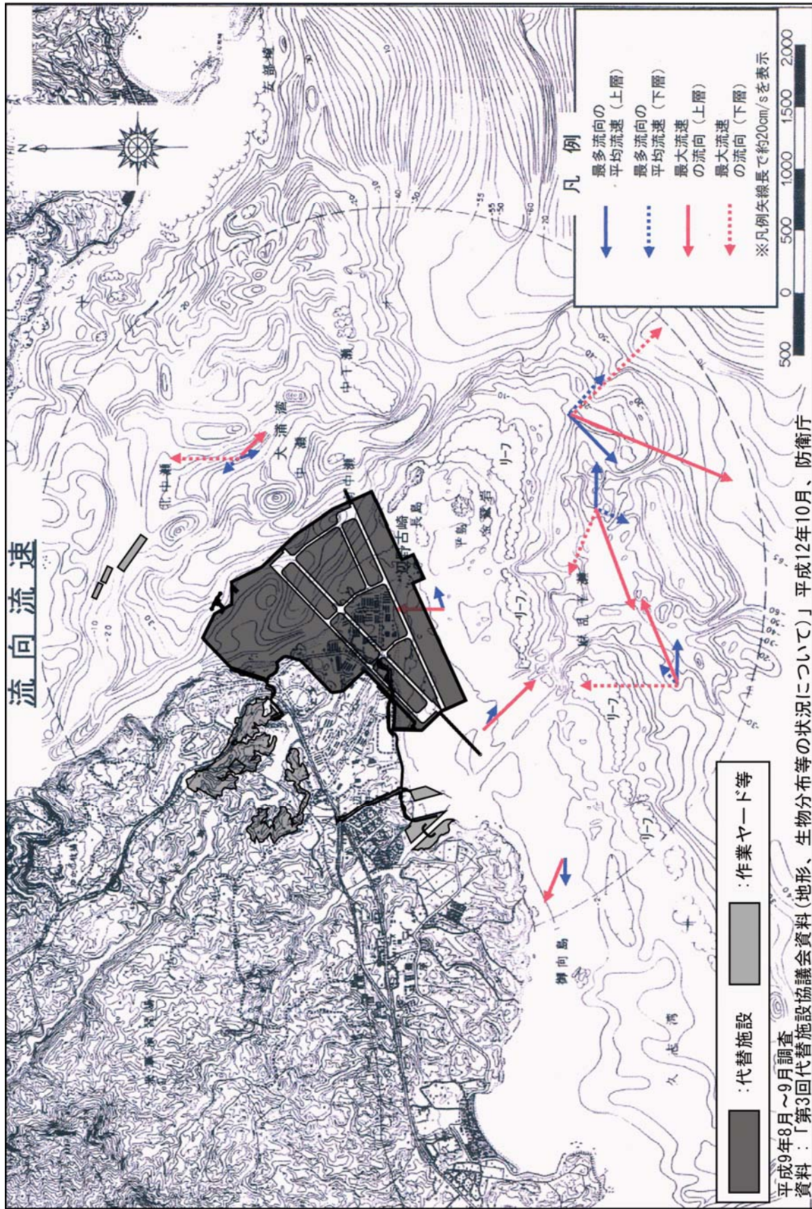
図-3.1.2.3 流向流速
