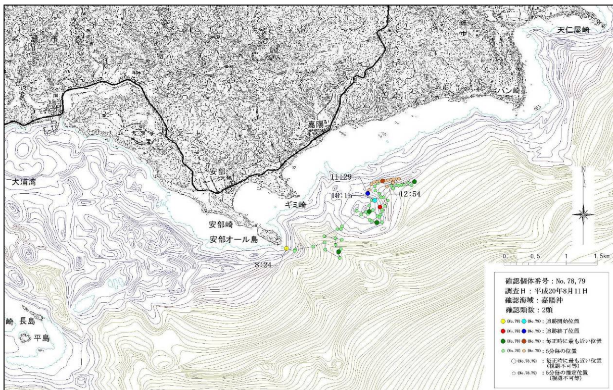
図-6. 16. 1. 7(29) 嘉陽沖で確認された個体の行動軌跡(平成 20 年 8 月 11 日、No.78、79)
