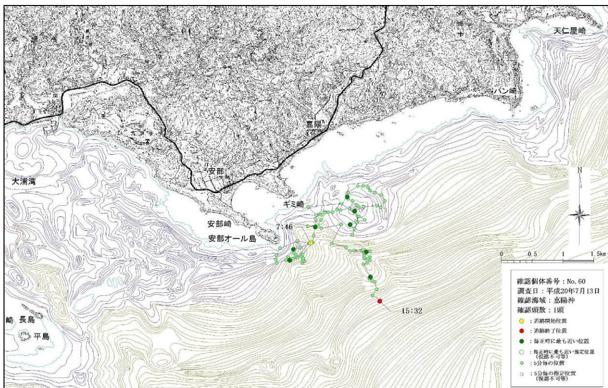
図-6. 16. 1. 7(21) 嘉陽沖で確認された個体の行動軌跡（平成20年7月13日、No.60）
