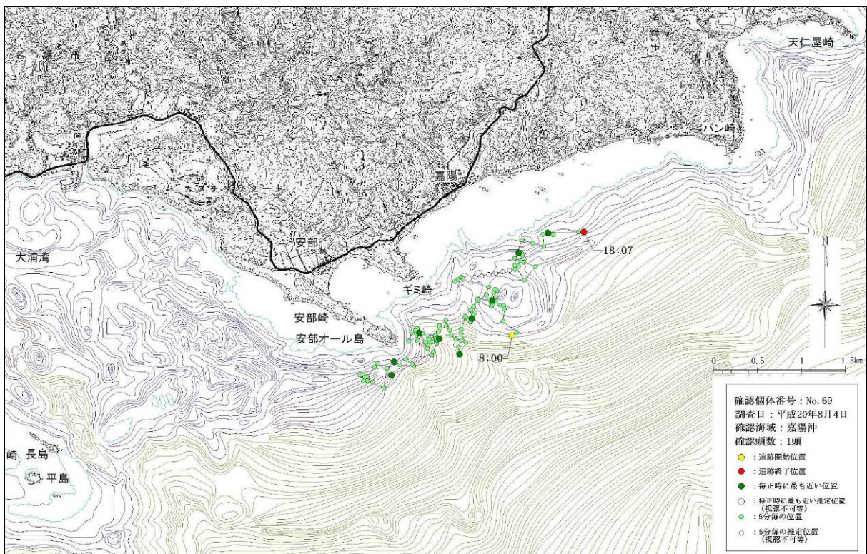
図-6. 16. 1. 7(25) 嘉陽沖で確認された個体の行動軌跡（平成 20 年 8 月 4 日、No.69）
