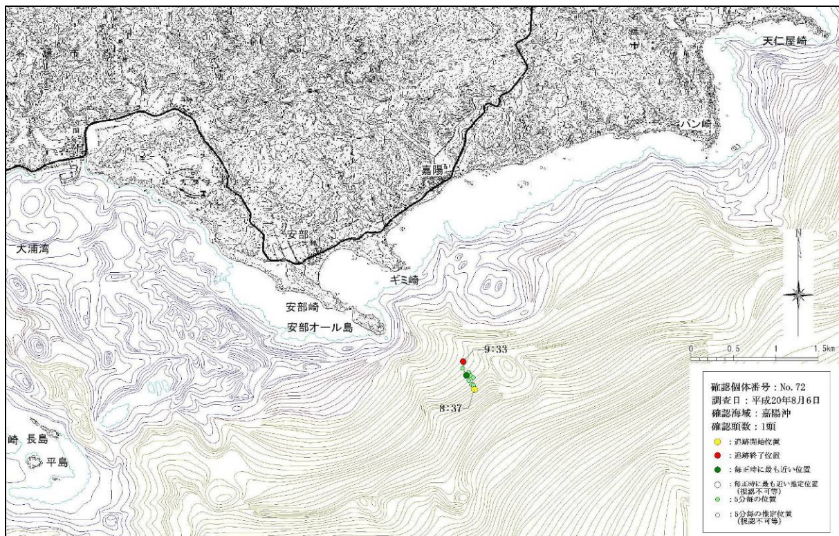
図-6. 16. 1. 7(26) 嘉陽沖で確認された個体の行動軌跡 (平成 20 年 8 月 6 日、No.72)
