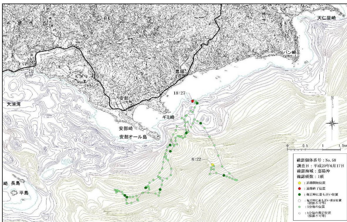
図-6. 16. 1. 7(19) 嘉陽沖で確認された個体の行動軌跡 (平成 20 年 6 月 17 日、No.58)
