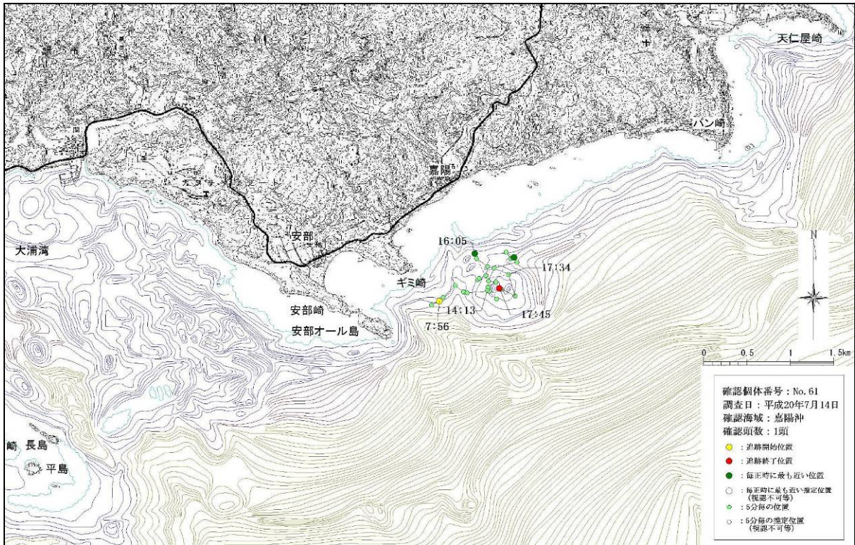
図-6. 16. 1. 7(22) 嘉陽沖で確認された個体の行動軌跡（平成20年7月14日、No.61）
