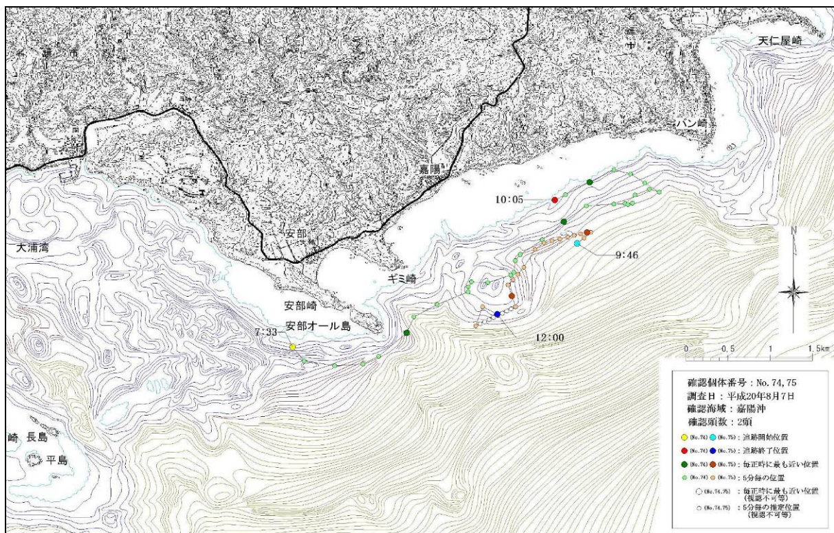
図-6. 16. 1. 7(27) 嘉陽沖で確認された個体の行動軌跡(平成 20 年 8 月 7 日、No.74、75)
