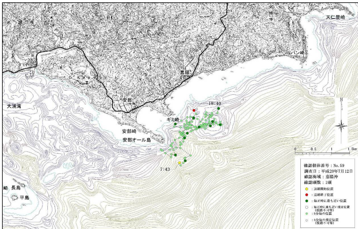
図-6. 16. 1. 7(20) 嘉陽沖で確認された個体の行動軌跡（平成20年7月12日、No.59）
