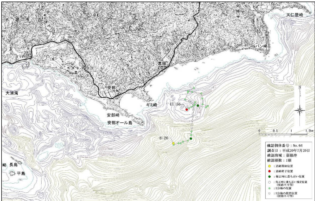
図-6. 16. 1. 7(23) 嘉陽沖で確認された個体の行動軌跡（平成20年7月20日、No.64）
