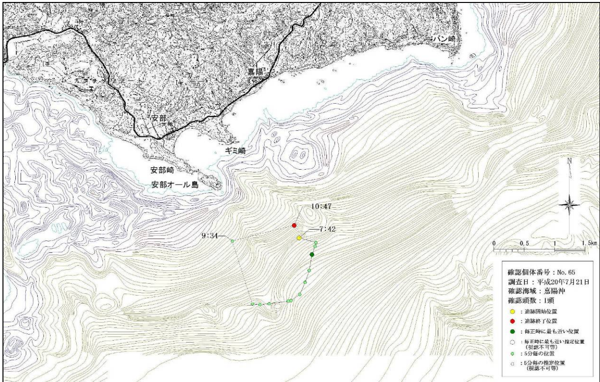
図-6. 16. 1. 7(24) 嘉陽沖で確認された個体の行動軌跡（平成 20 年 7 月 21 日、No.65）
