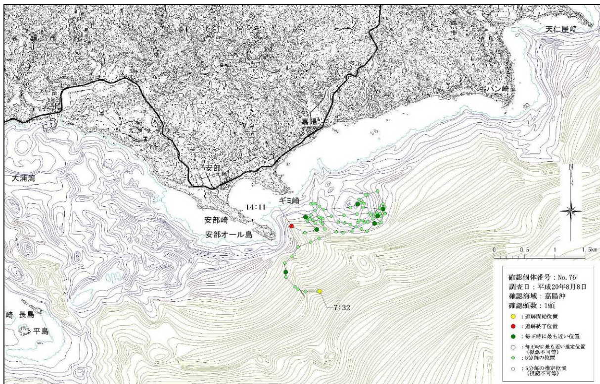
図-6. 16. 1. 7(28) 嘉陽沖で確認された個体の行動軌跡 (平成 20 年 8 月 8 日、No.76)
