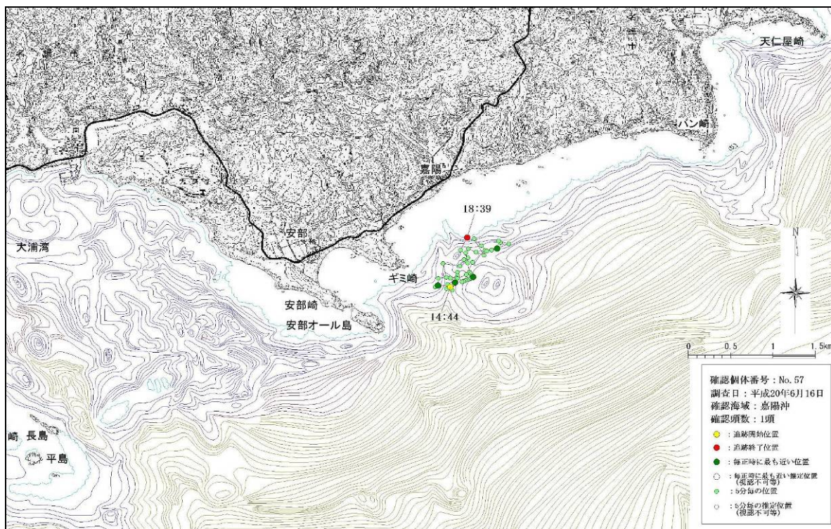
図-6. 16. 1. 7(18) 嘉陽沖で確認された個体の行動軌跡 (平成 20 年 6 月 16 日、No.57)
