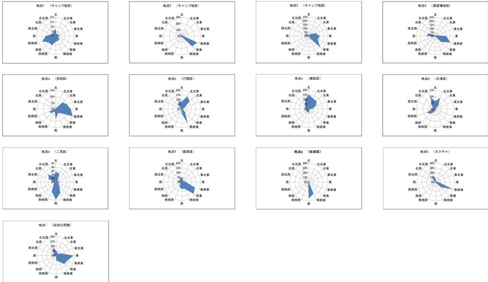
図-6. 11. 13 気象状況調査に基づく風配図
