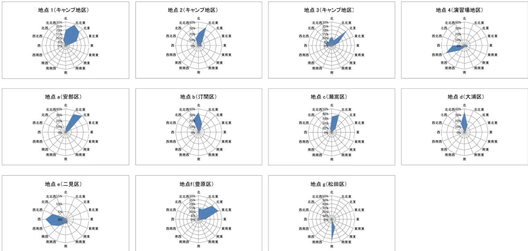
図-6.11.3 気象状況調査に基づく風配図
