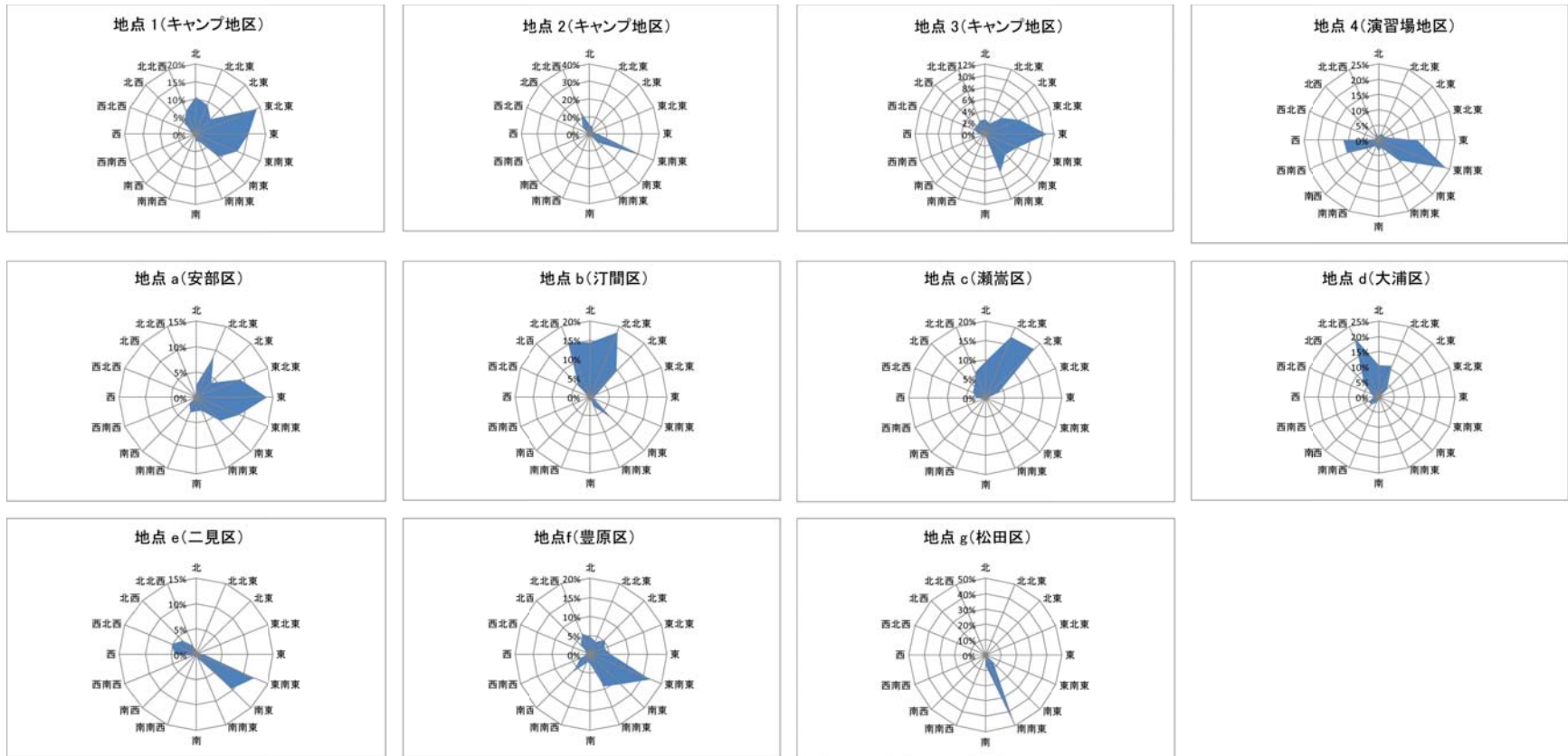
図-6.11.1 気象状況調査に基づく風配図
