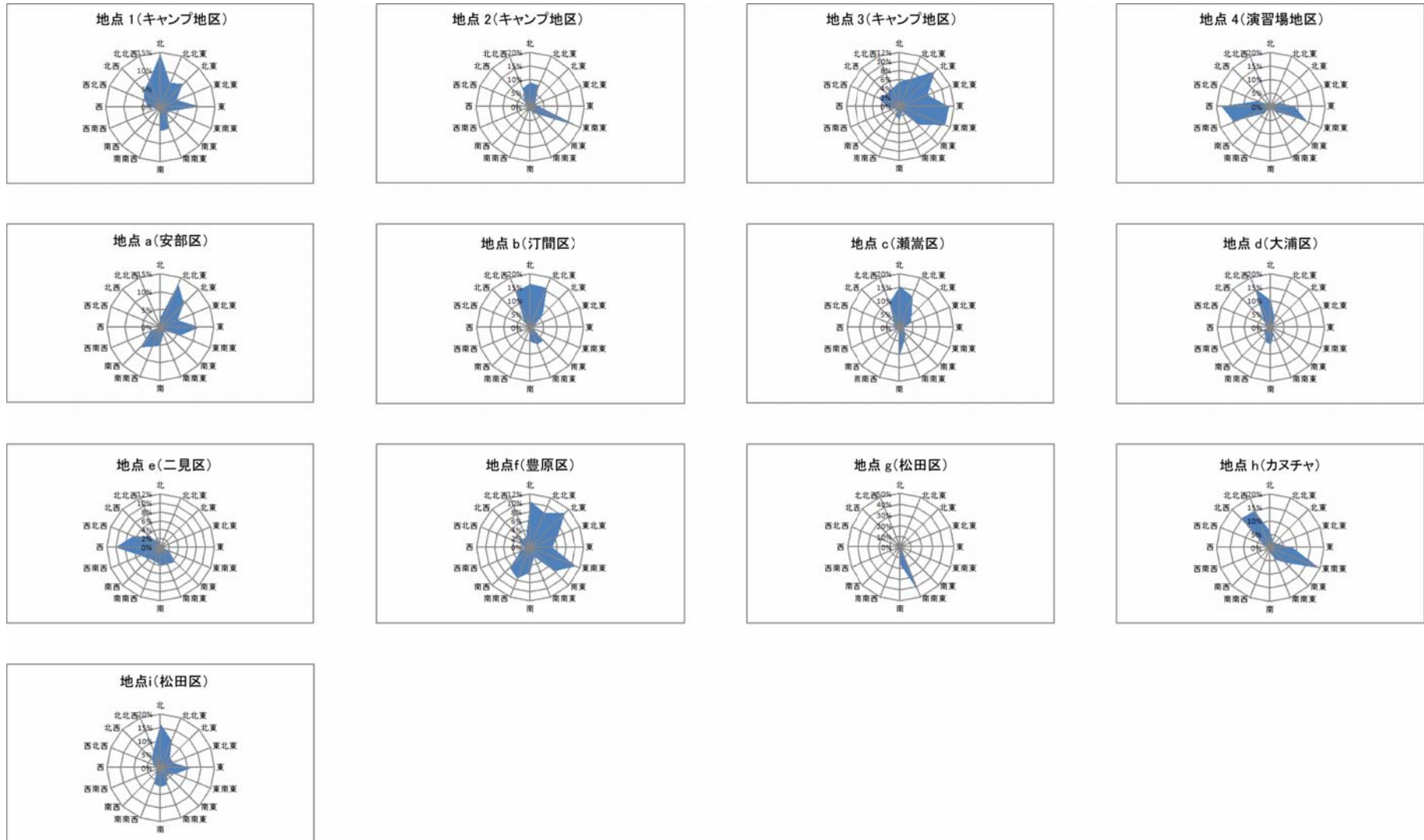
図-6. 11. 9 気象状況調査に基づく風配図
