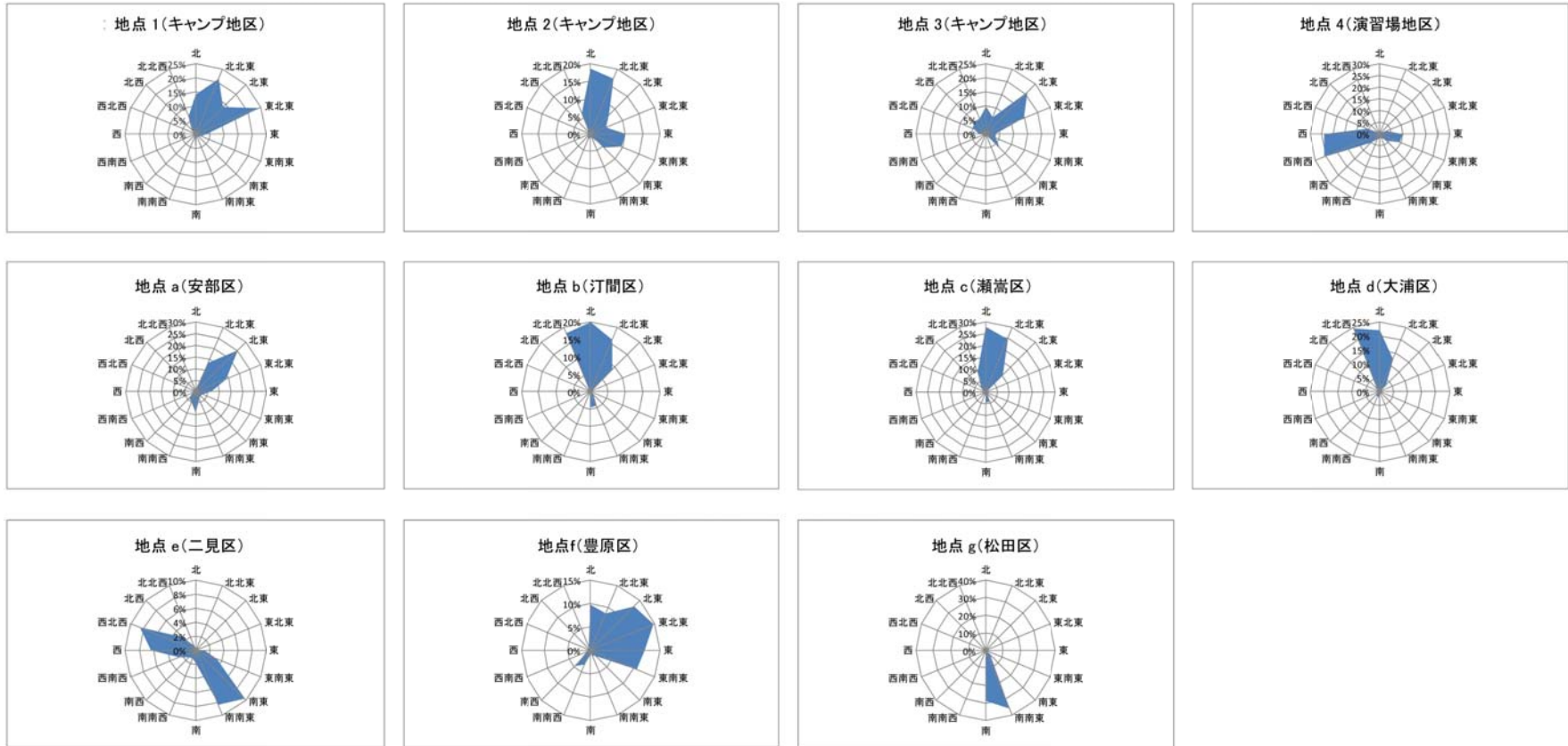
図-6.11.2 気象状況調査に基づく風配図
