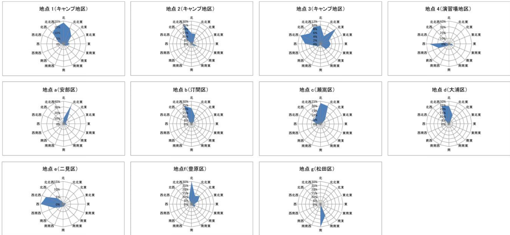
図-6. 11. 4 気象状況調査に基づく風配図
