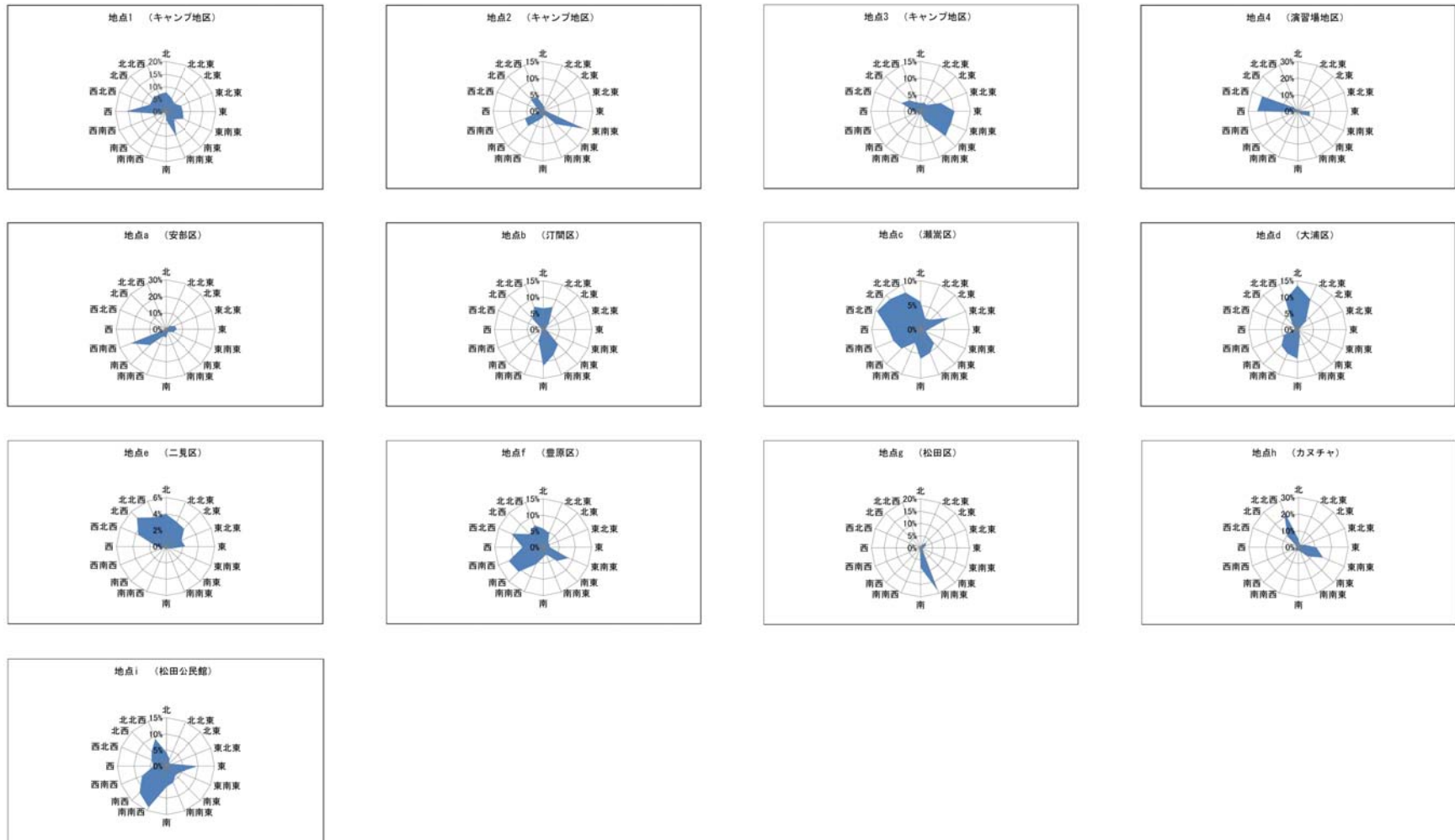
図-6. 11. 12 気象状況調査に基づく風配図
