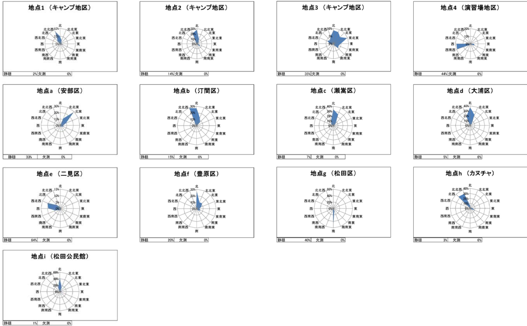
図-6. 11. 16 気象状況調査に基づく風配図
