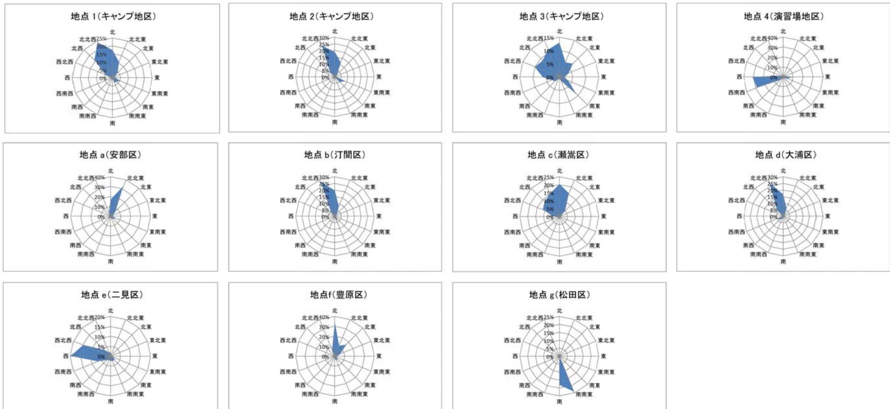
図-6.11.5 気象状況調査に基づく風配図
