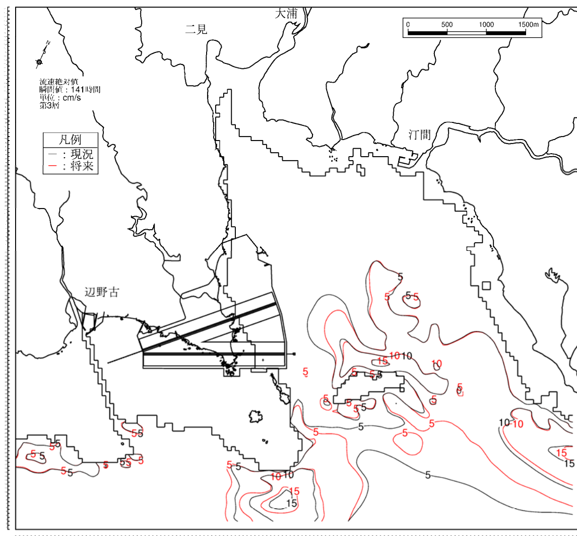
図-6.9.2.2.21(3) 供用時の流速分布の変化（冬季、上げ潮時） 第3層[4~6m]
