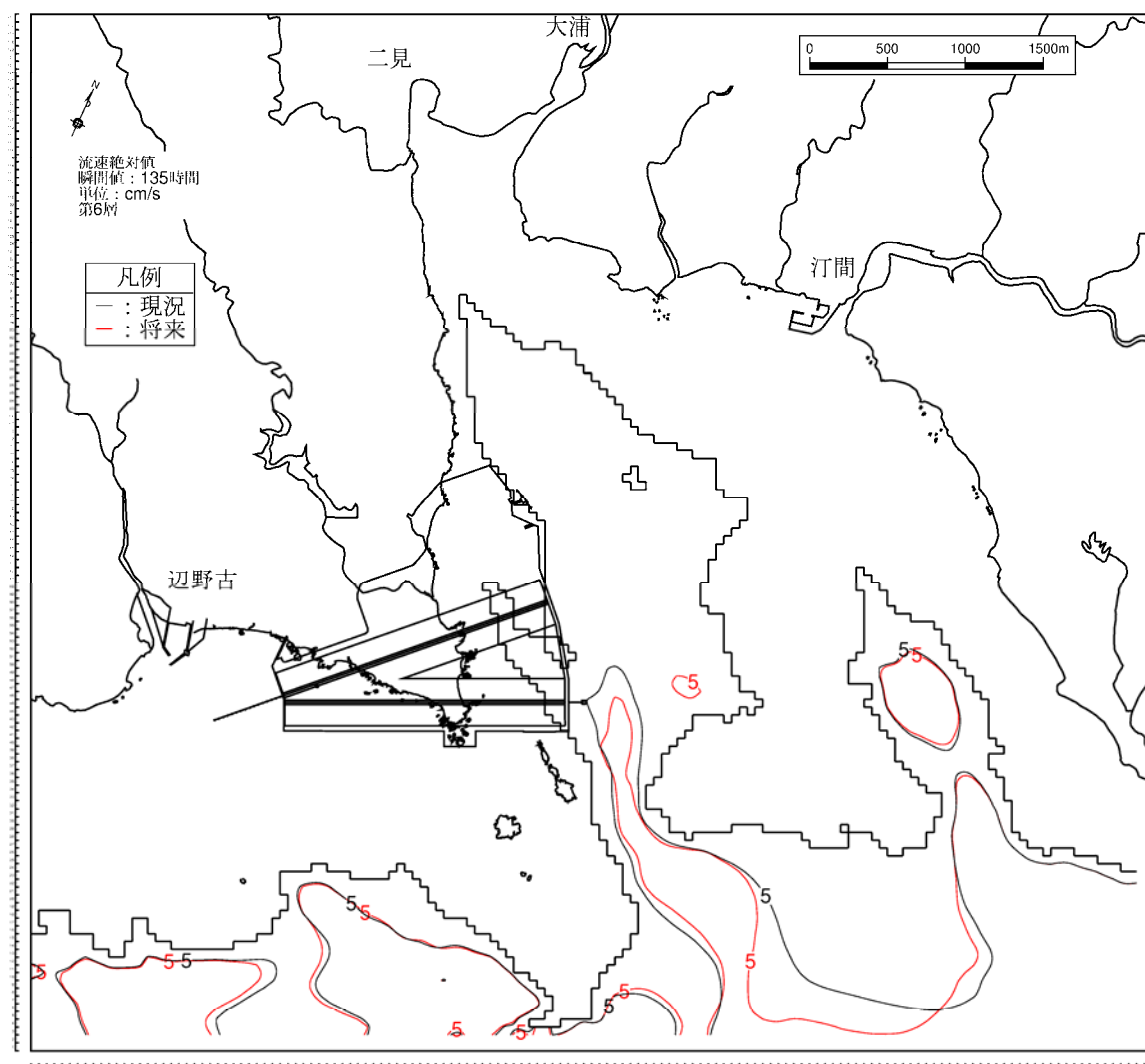
図-6.9.2.2.20(6) 供用時の流速分布の変化 (冬季、下げ潮時) 第6層[20m以深]
