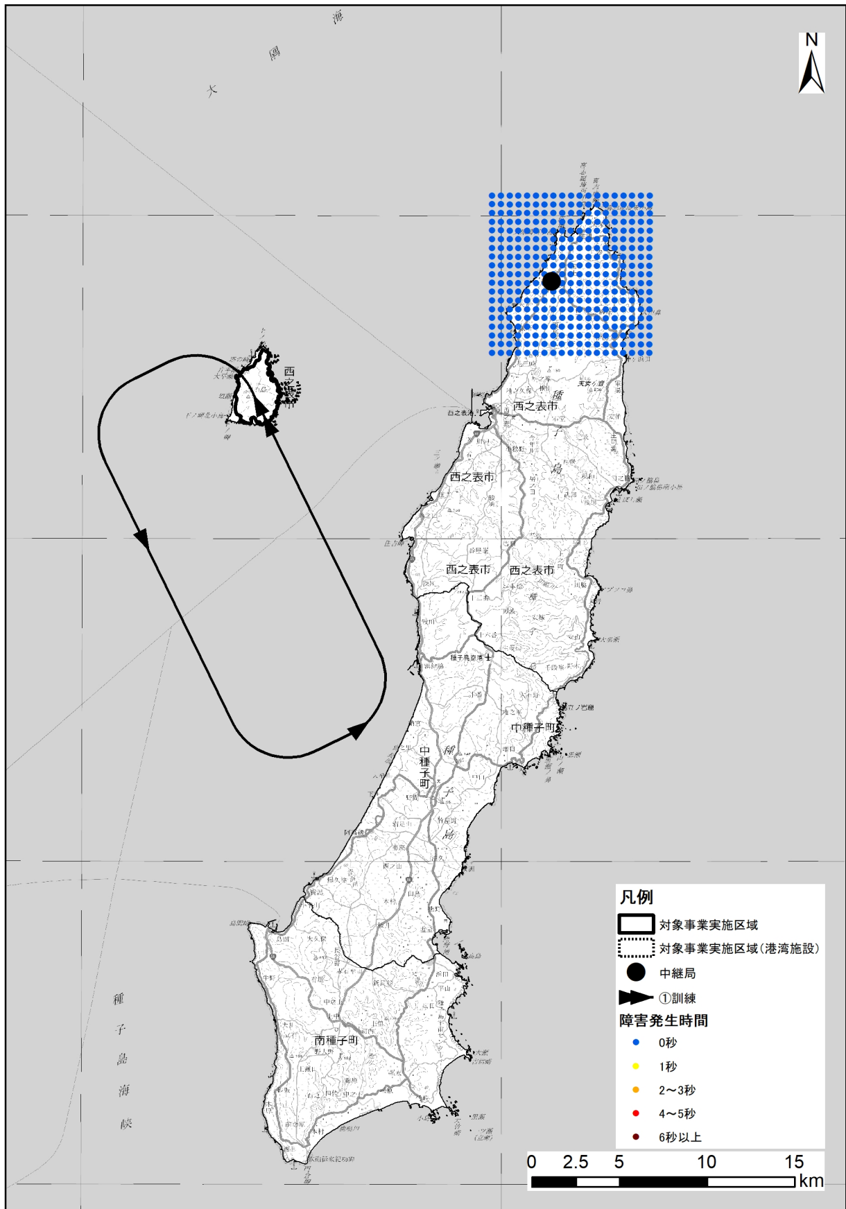
図-6.10.7(3) ケース 2 (ルート①訓練：高度 1,500ft) 予測結果 (国上中継局)
