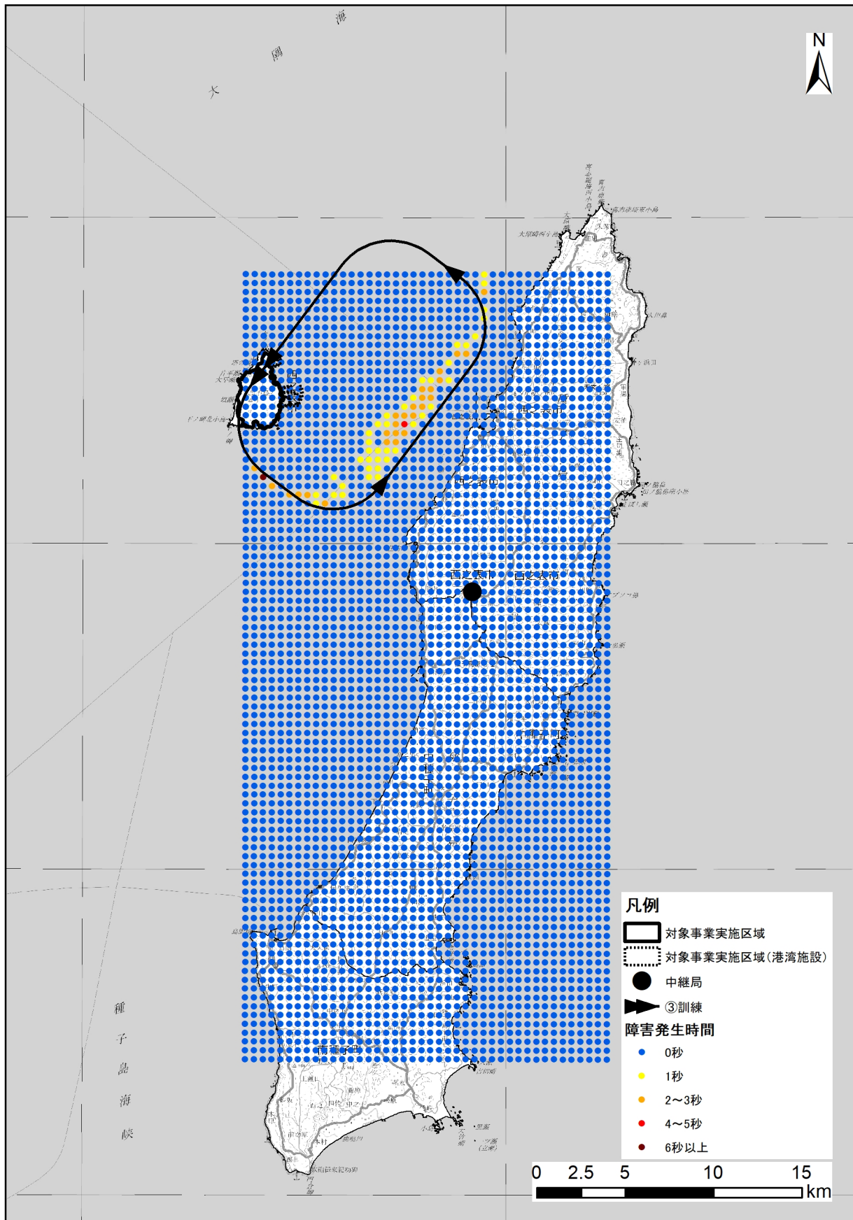
図-6.10.10(1) ケース5 (ルート③訓練：高度1,200ft) 予測結果 (種子島中継局)
