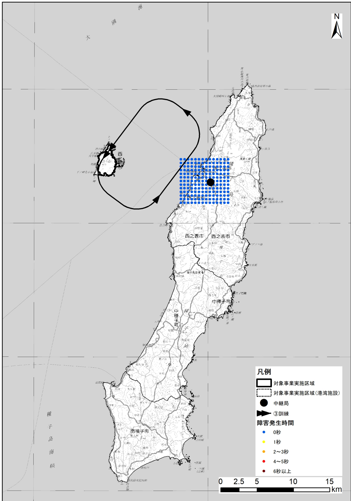
図-6.10.10(2) ケース5 (ルート③訓練：高度1,200ft) 予測結果 (西之表東中継局)
