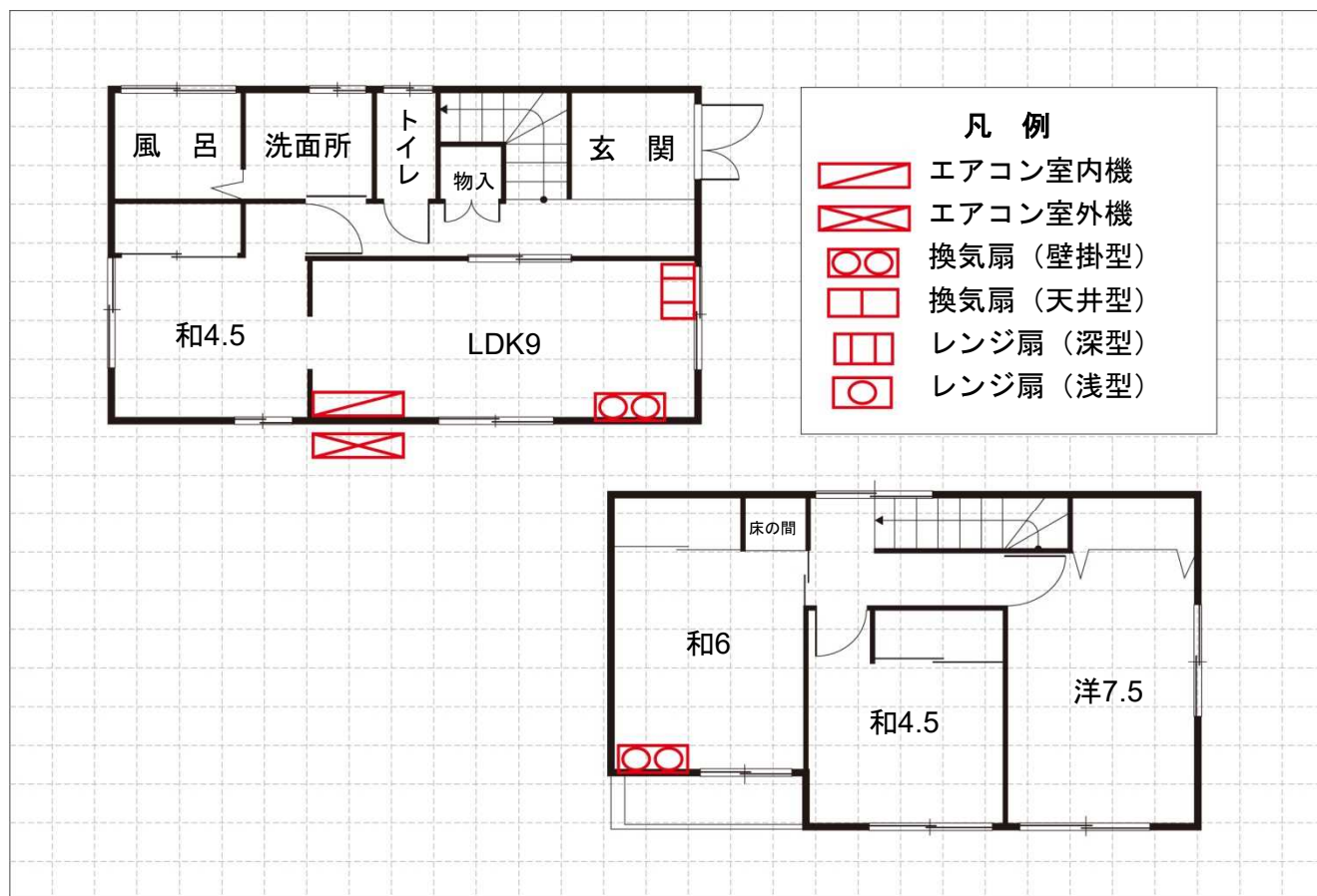
見取図の例
