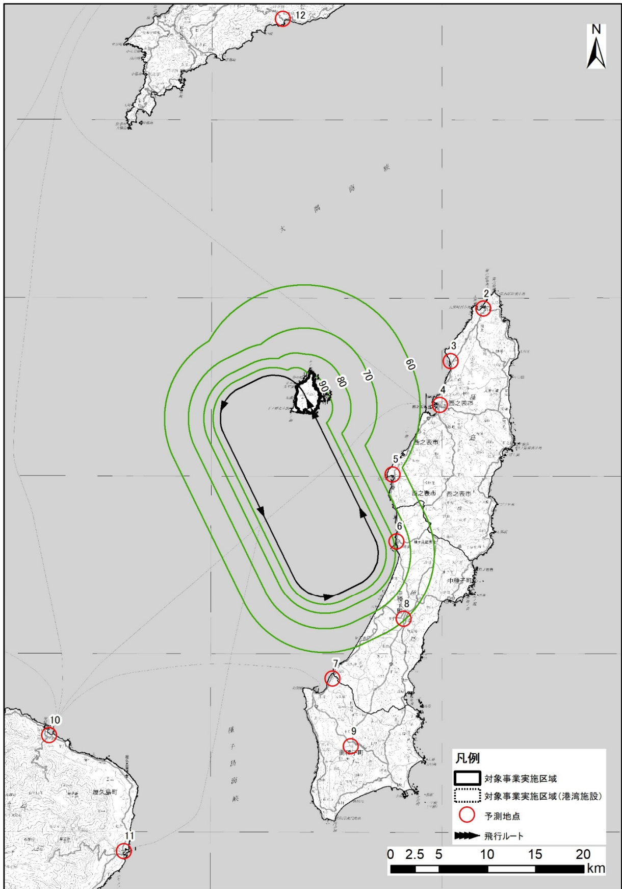
図-6.3.7(1) 最大騒音レベル (LA, Smax) の予測コンター (飛行経路①) : 単位 dB
