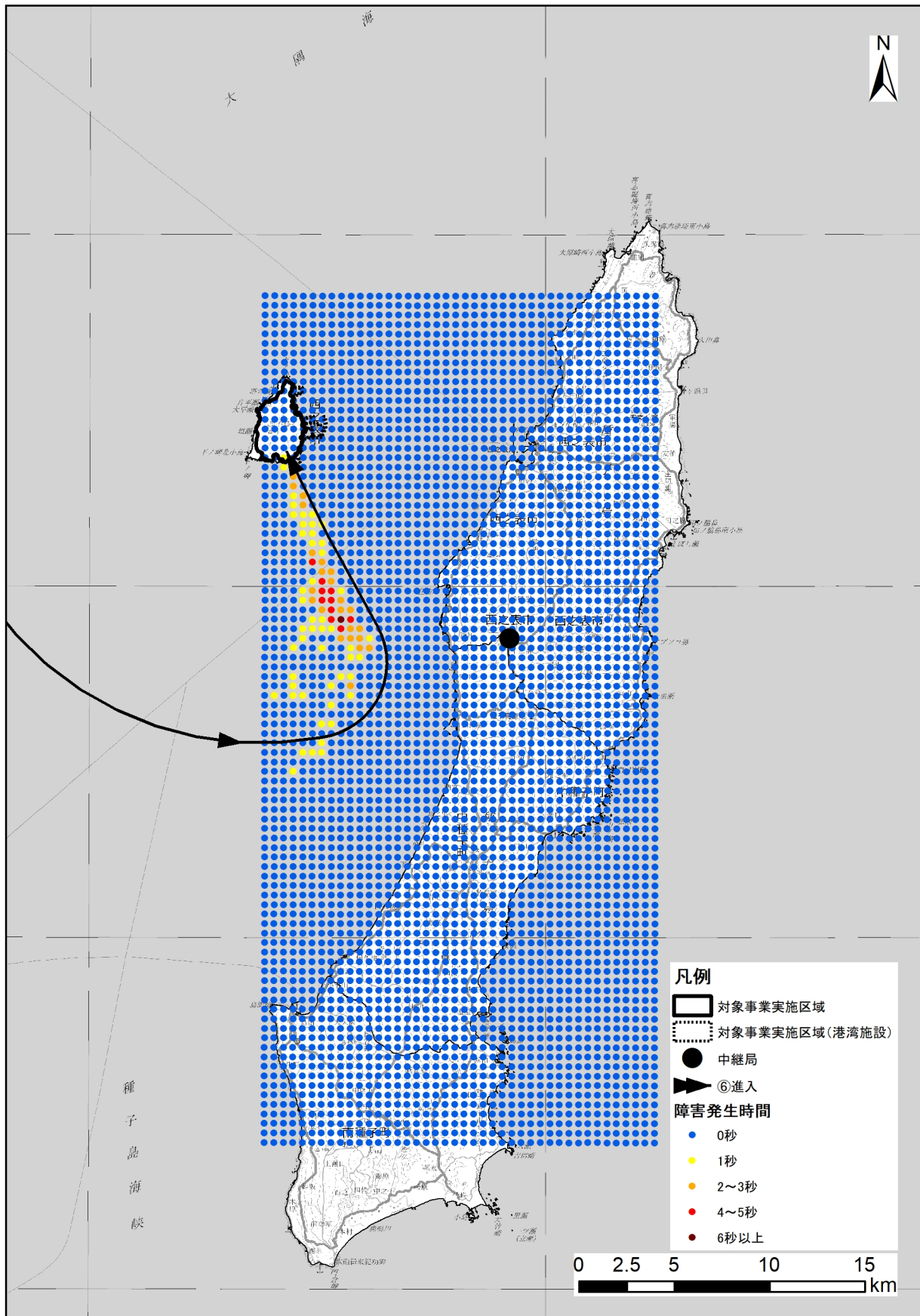
図-6.10.16(1) ケース 11 (ルート⑥進入：速度 220 ノット) 予測結果 (種子島中継局)
