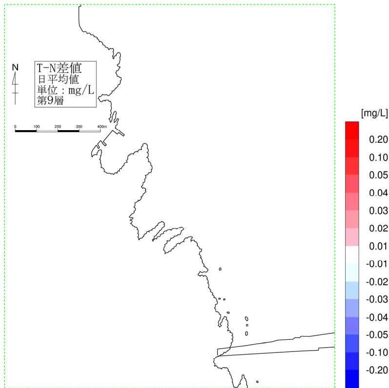
図-6. 6. 23(9) 供用時の水質濃度変化（夏季、T-N、第9層[50~100m]）
