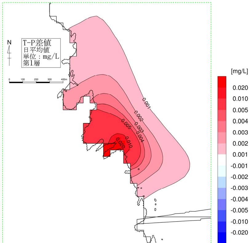
図-6. 6. 24(1) 供用時の水質濃度変化（夏季、T-P、第1層[0~2m]）
