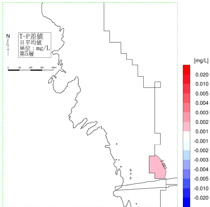
図-6. 6. 30(5) 供用時の水質濃度変化（冬季、T-P、第5層[10~15m]）
