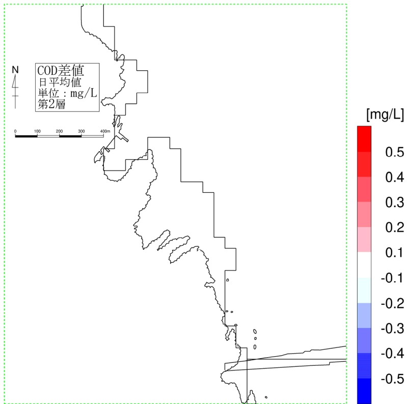
図-6. 6. 22(2) 供用時の水質濃度変化（夏季、COD、第2層[2~4m]）
