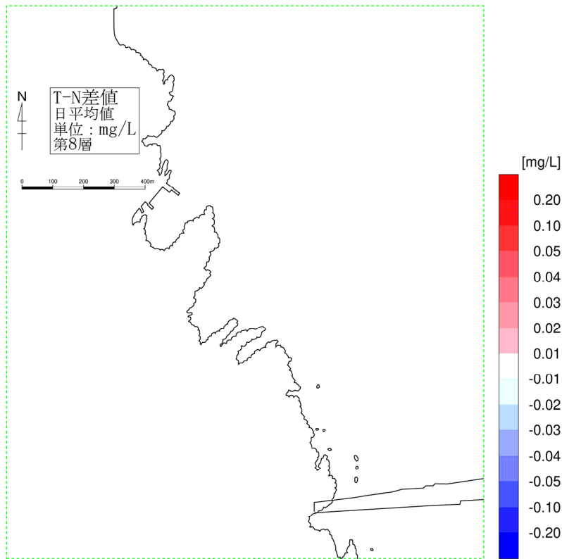
図-6. 6. 29(8) 供用時の水質濃度変化 (冬季、T-N、第8層[30~50m])
