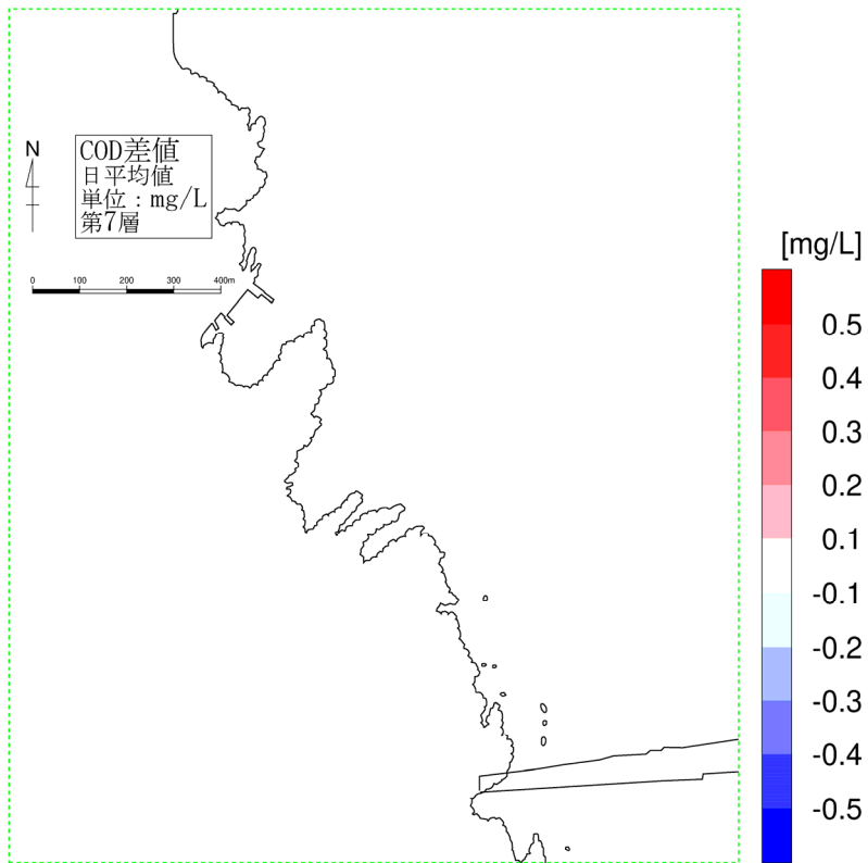
図-6. 6. 22(7) 供用時の水質濃度変化 (夏季、COD、第7層[20~30m])
