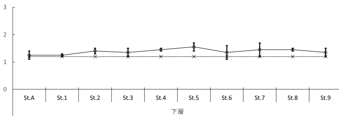
下層COD(mg/L)
