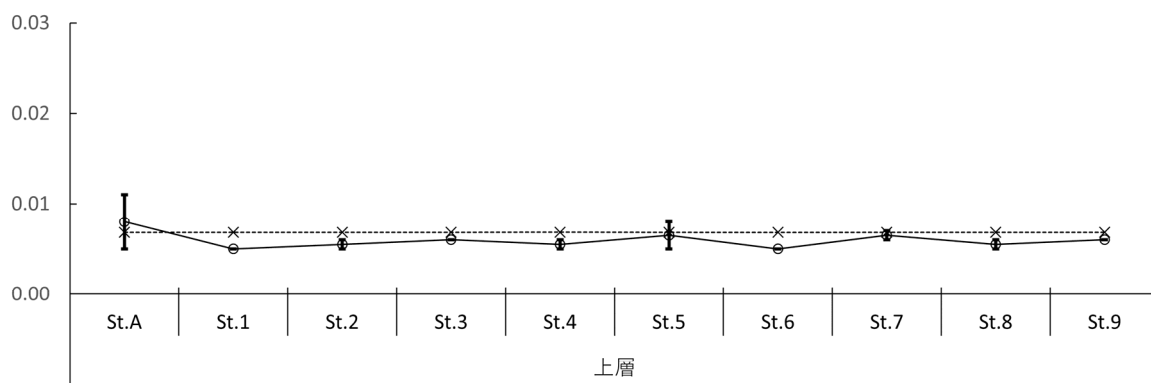
上層T-P(mg/L)
