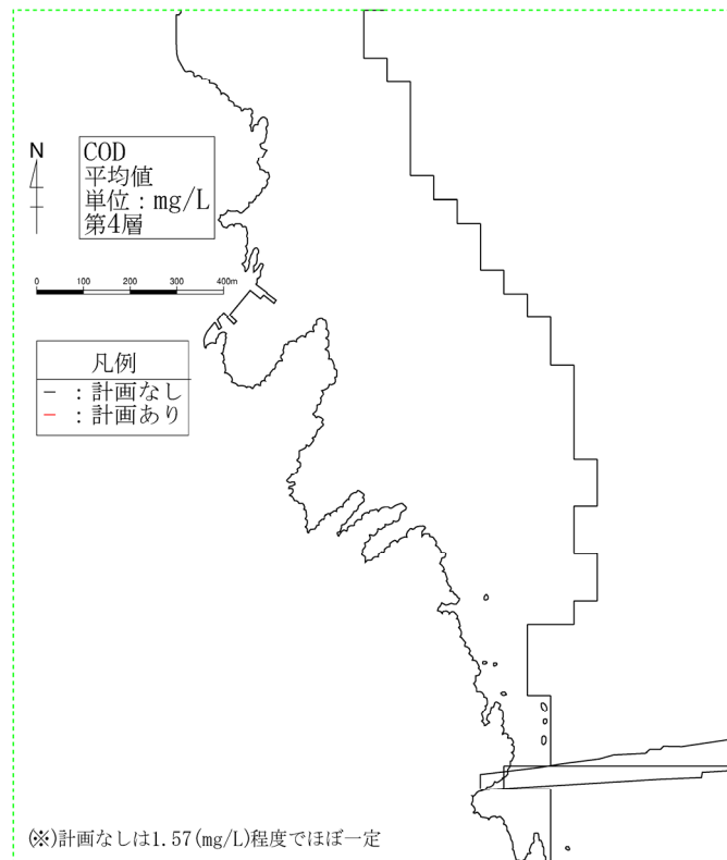
図-6.6.25(4) 供用時の水質濃度分布 (冬季COD、第4層[7~10m])
