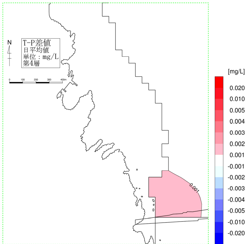
図-6.6.30(4) 供用時の水質濃度変化（冬季、T-P、第4層[7~10m]）
