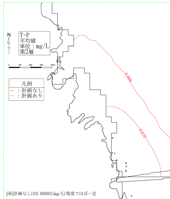
図-6.6.27(2) 供用時の水質濃度分布 (冬季 T-P、第2層[2~4m])
