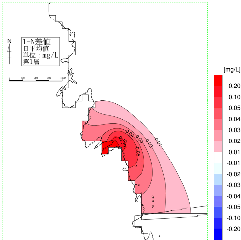
図-6. 6. 29(1) 供用時の水質濃度変化 (冬季、T-N、第1層[0~2m])
