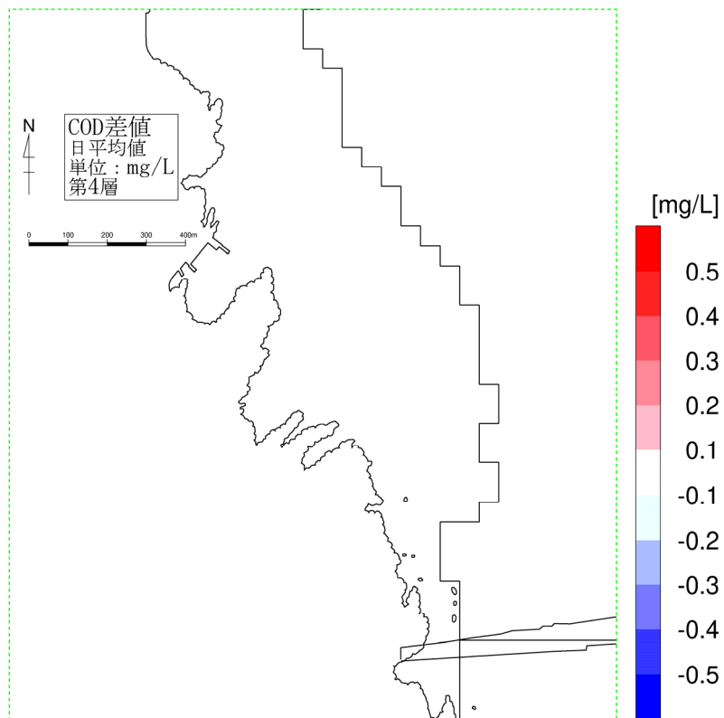
図-6.6.28(4) 供用時の水質濃度変化 (冬季、COD、第4層[7~10m])
