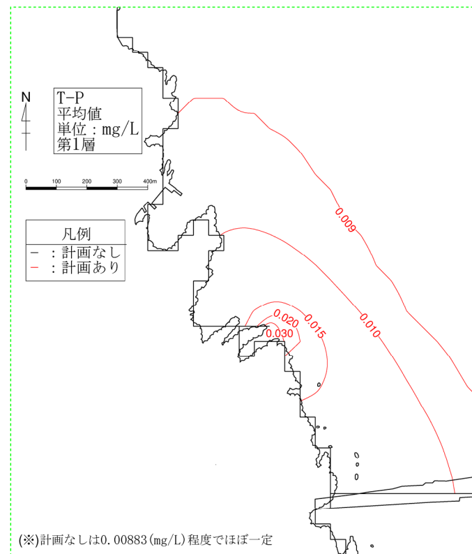
図-6.6.27(1) 供用時の水質濃度分布 (冬季T-P、第1層[0~2m])
