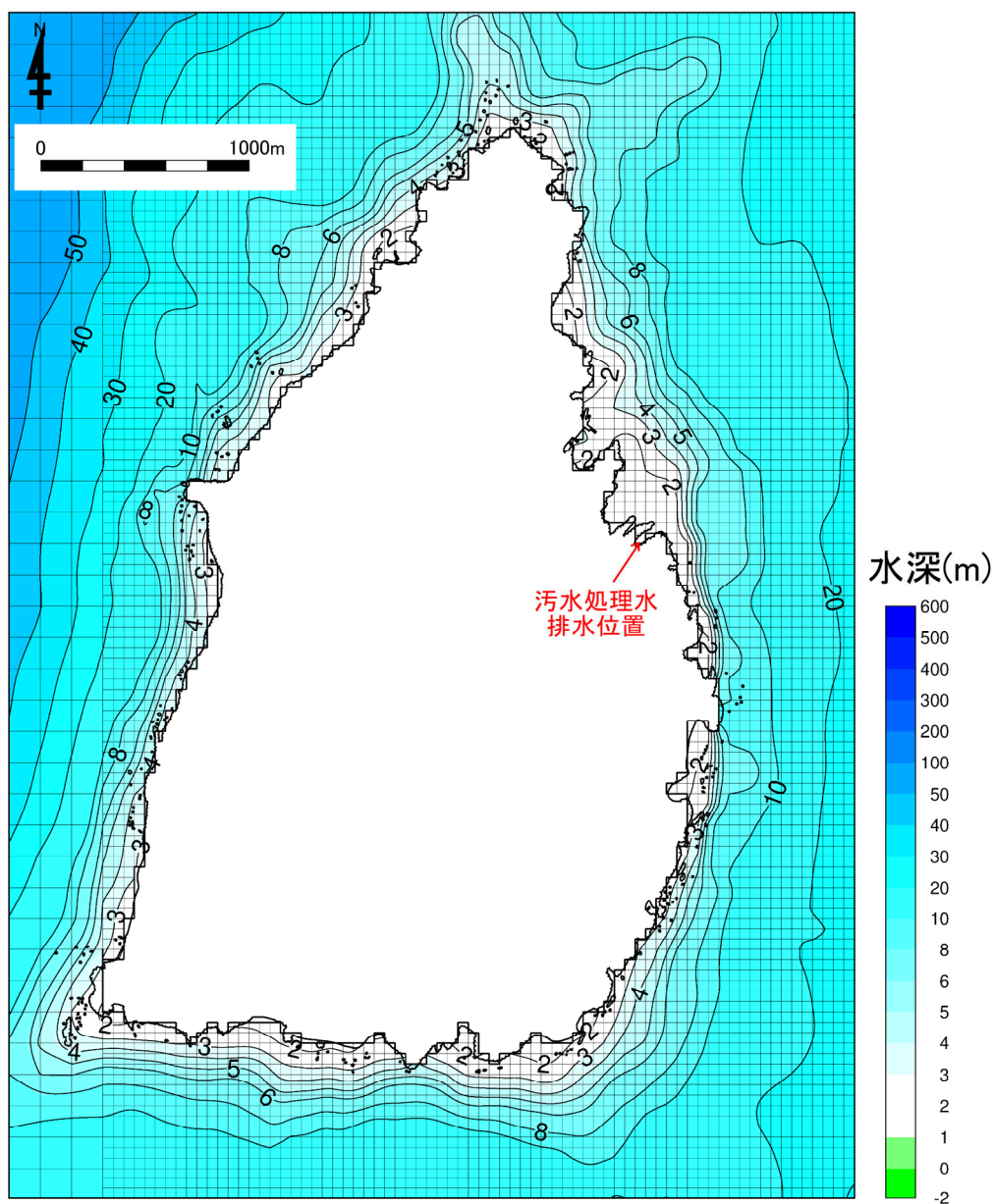
図-6.6.5 汚水処理水の排水位置 (存在及び供用時)
