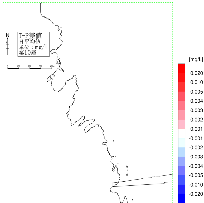
図-6.6.30(10) 供用時の水質濃度変化（冬季、T-P、第10層[100m以深]）
