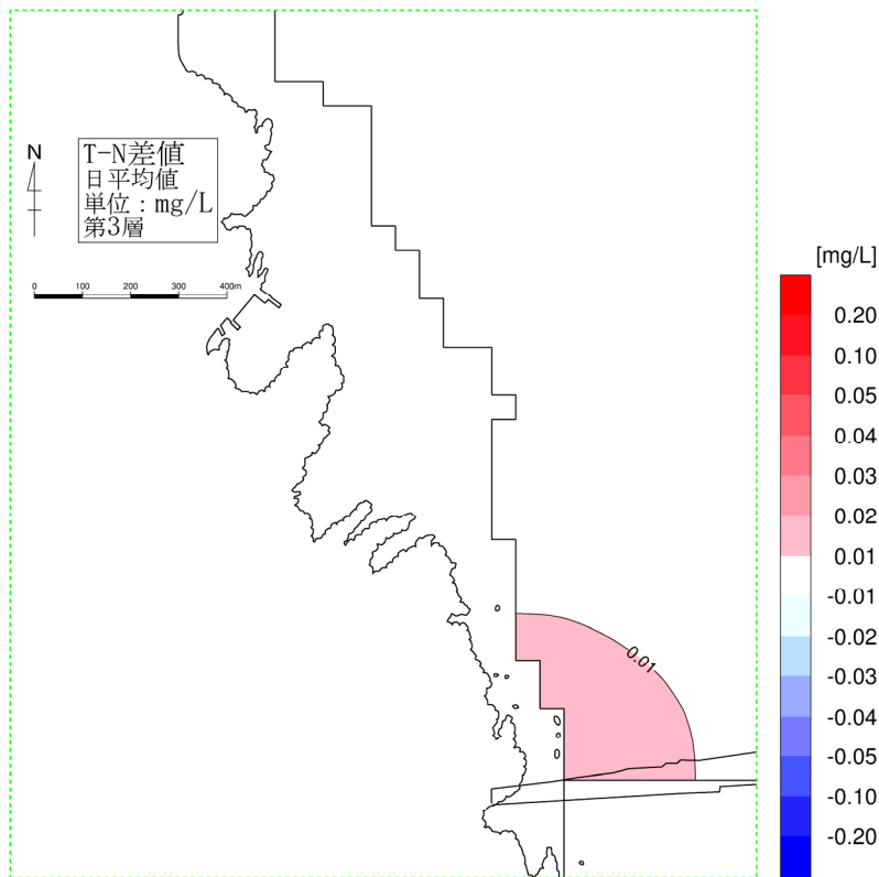
図-6. 6. 29(3) 供用時の水質濃度変化 (冬季、T-N、第3層[4~7m])
