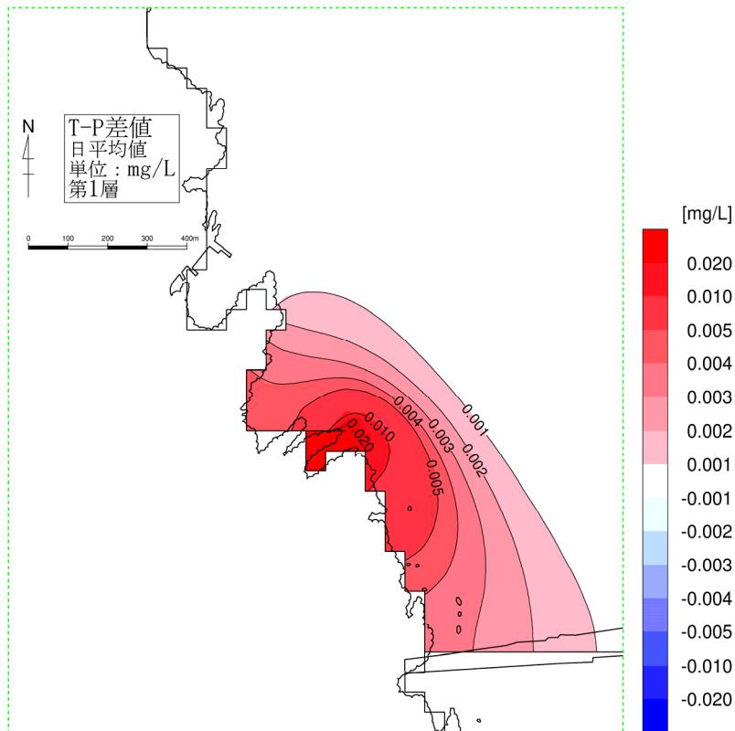
図-6. 6. 30(1) 供用時の水質濃度変化 (冬季、T-P、第1層[0~2m])
