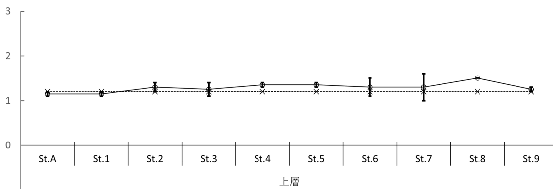
上層COD(mg/L)
