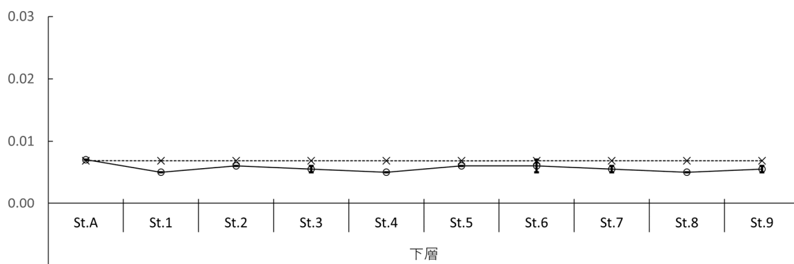
下層T-P(mg/L)
