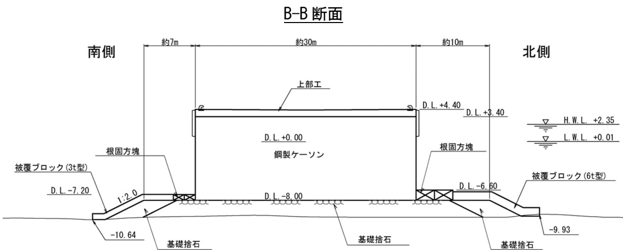
図-2.2.31(2) 仮設栈橋の平面図及び標準断面
