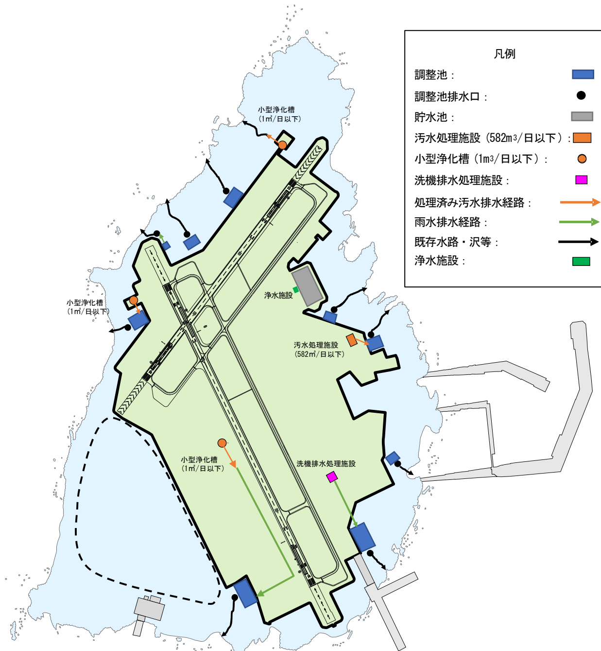
図-2. 2. 18 汚水処理水、雨水の放流位置
