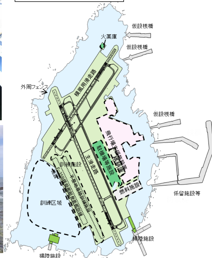
施設全体配置図
