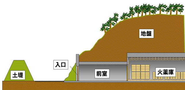
地中式
