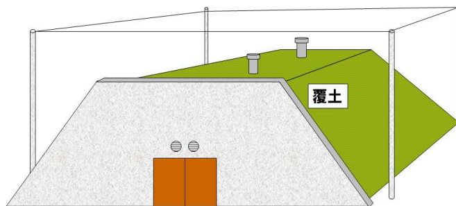
地上覆土式
