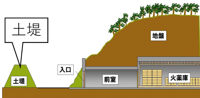
地中式
