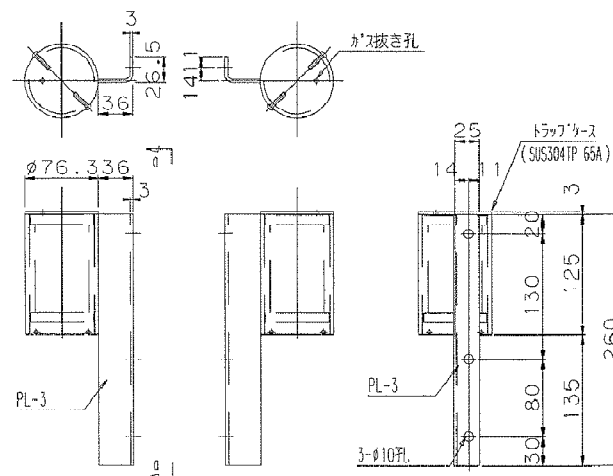
トラップ取付詳細図 S=1/5
