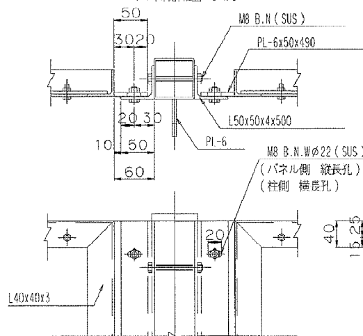
パネル取付詳細図 5-1/5
