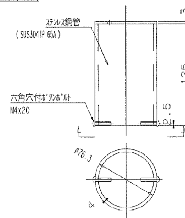
ト ラ ッ プ ケ ー ス S=1/3
