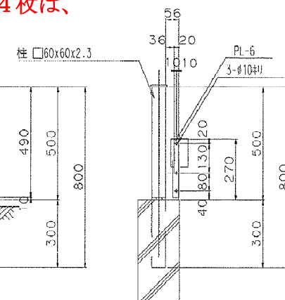
側面圖 S=1/15
