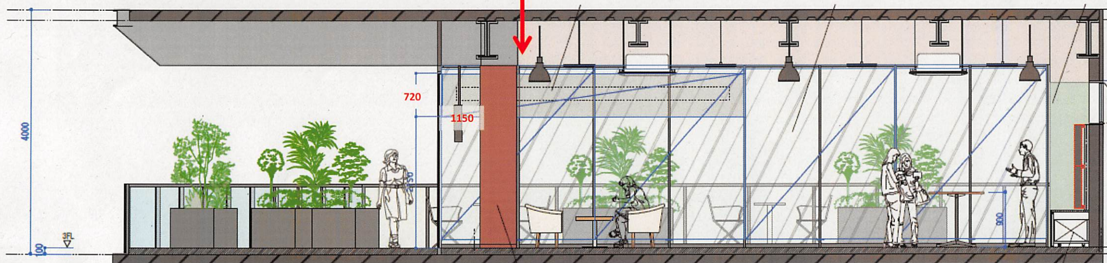
立面図（内装側）
