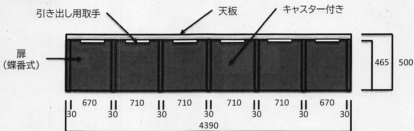
正面図
