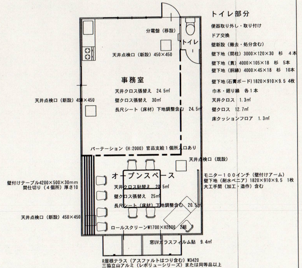
【改修平面図 1】
