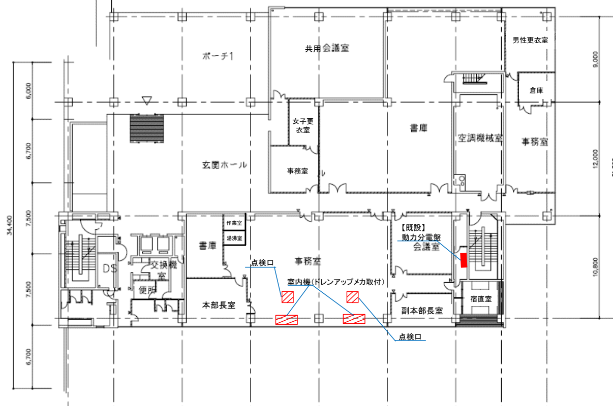
1階平面図
