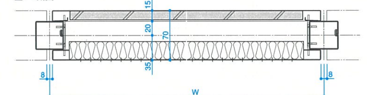
■G-G断面
