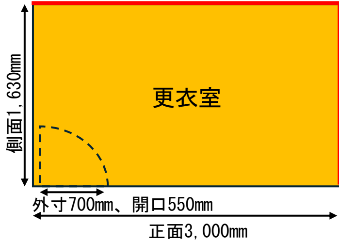
【平面図】
