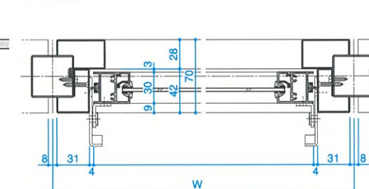
■F-F断面
