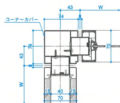
■L型コーナー
