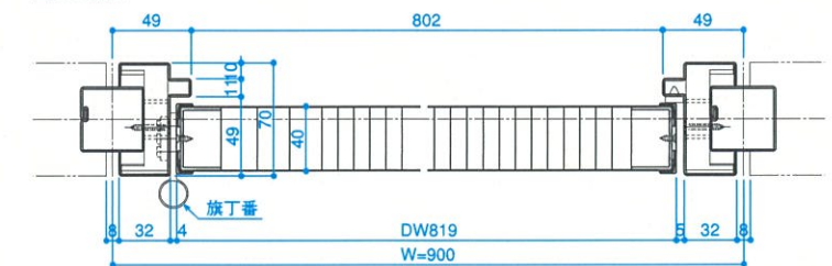
■H-H断面
