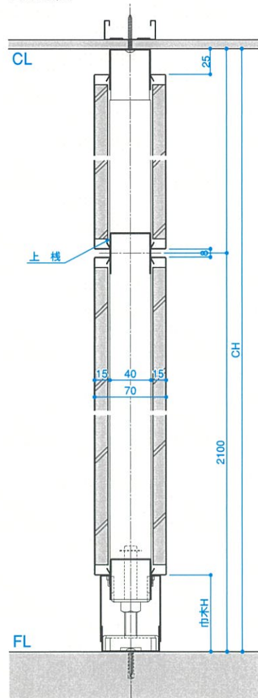
■B-B断面
