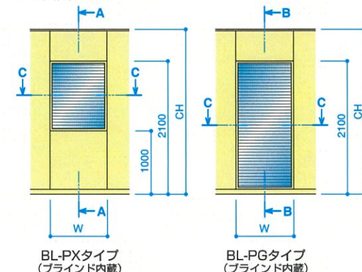
■立面図
