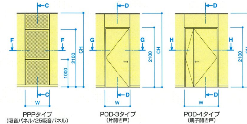
■製品寸法
