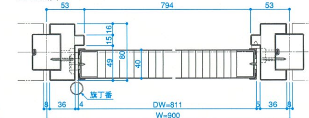
■E-E断面
