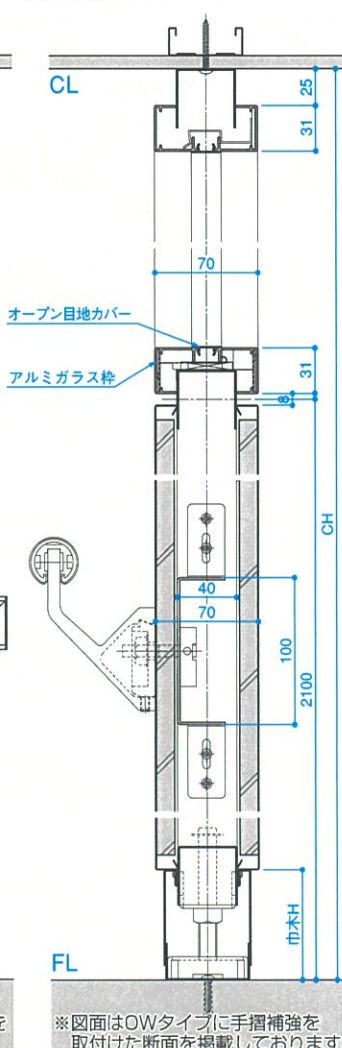
■E-E断面
