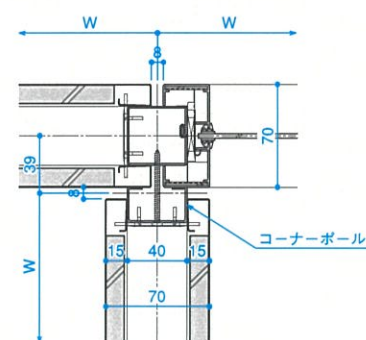
■T型コーナー
