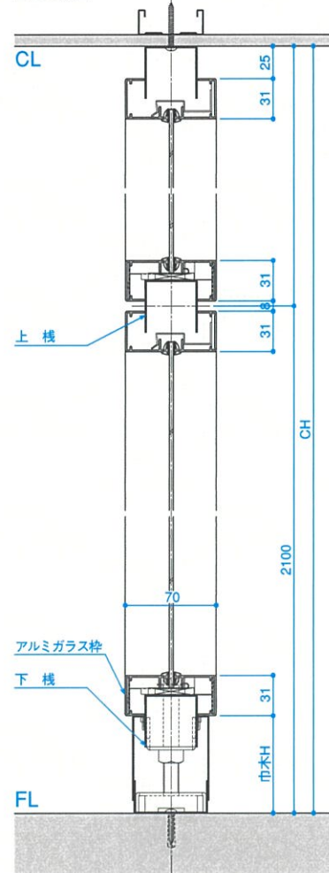
■B-B断面
