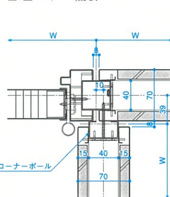
■T型コーナー（偏芯）
