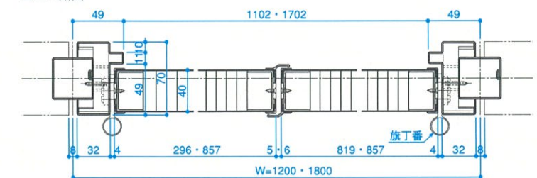
■H-H断面
