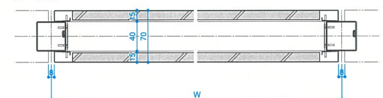
■F-F断面
