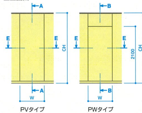
■立面図
