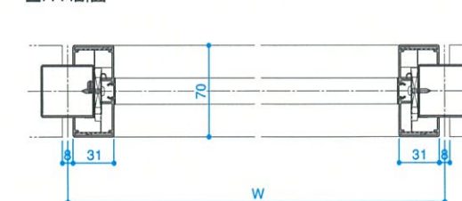
■H-H断面
