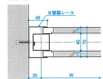
■壁面納まりB
