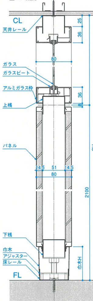
■A-A断面
