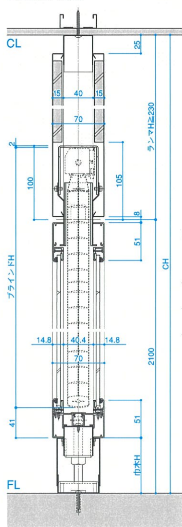
■B-B断面 (電動)
