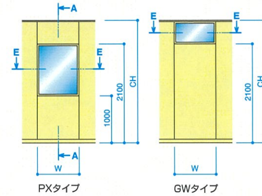
■立面図
