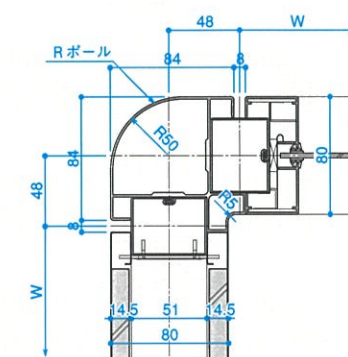
■C-C断面
