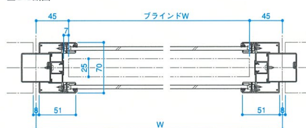
■C-C断面
