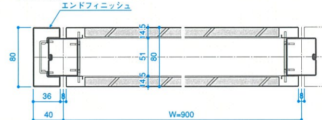
■D-D断面
