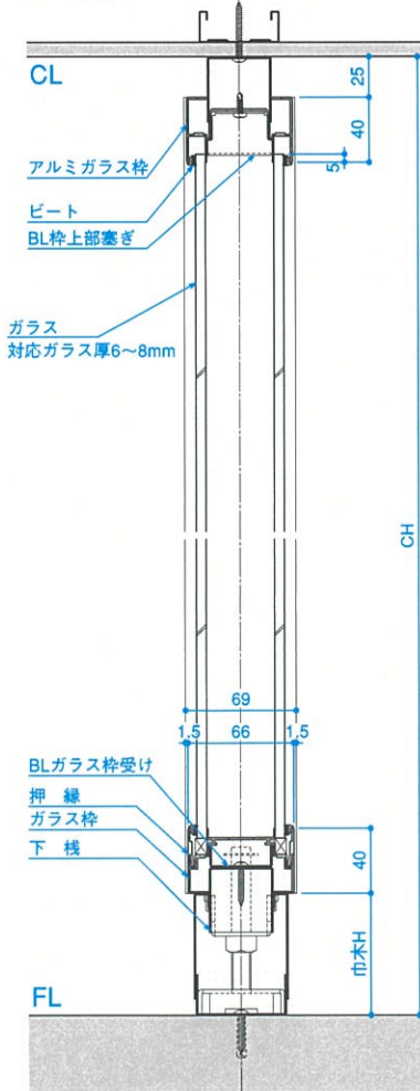
■D-D断面
