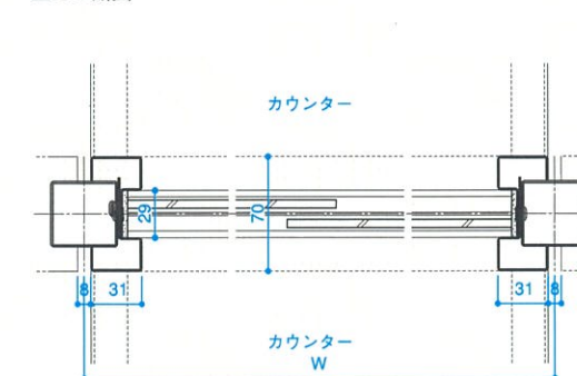
■G-G断面
