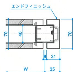
■エンドフィニッシュ
