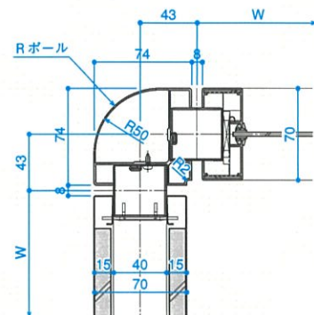
■Rボールコーナー
