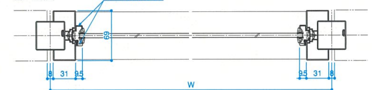
■F-F断面
