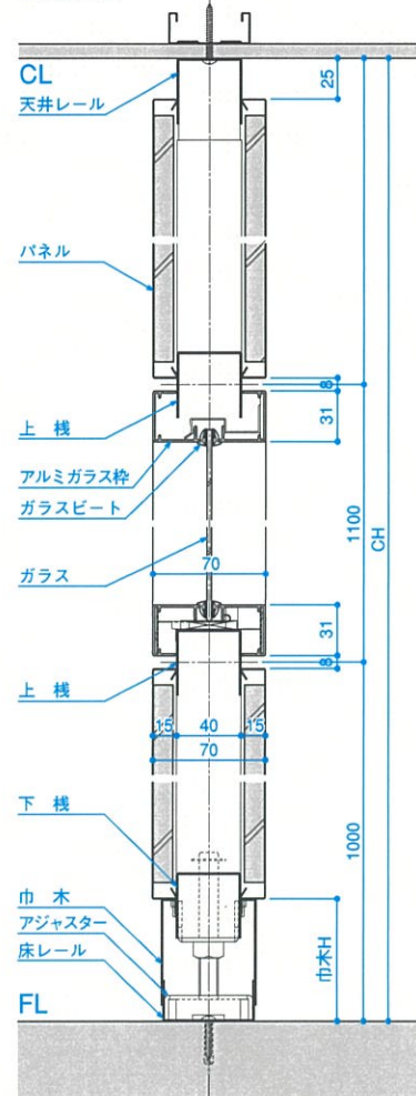
■A-A断面
