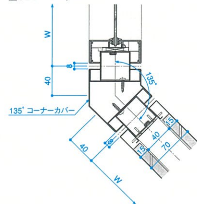
■135°コーナー
