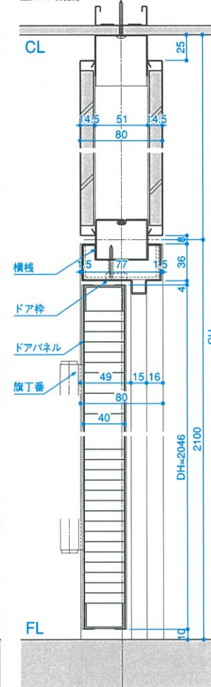
■B-B断面
