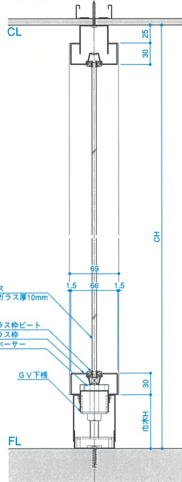
■C-C断面
