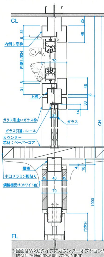
■D-D断面
