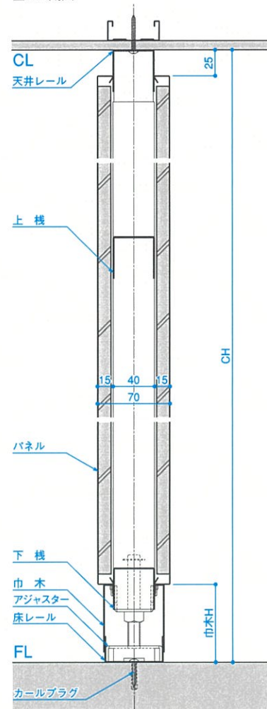
■A-A断面
