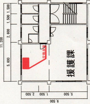
4 階平面図 1/200
