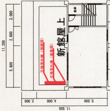
4 階平面図 1/200
