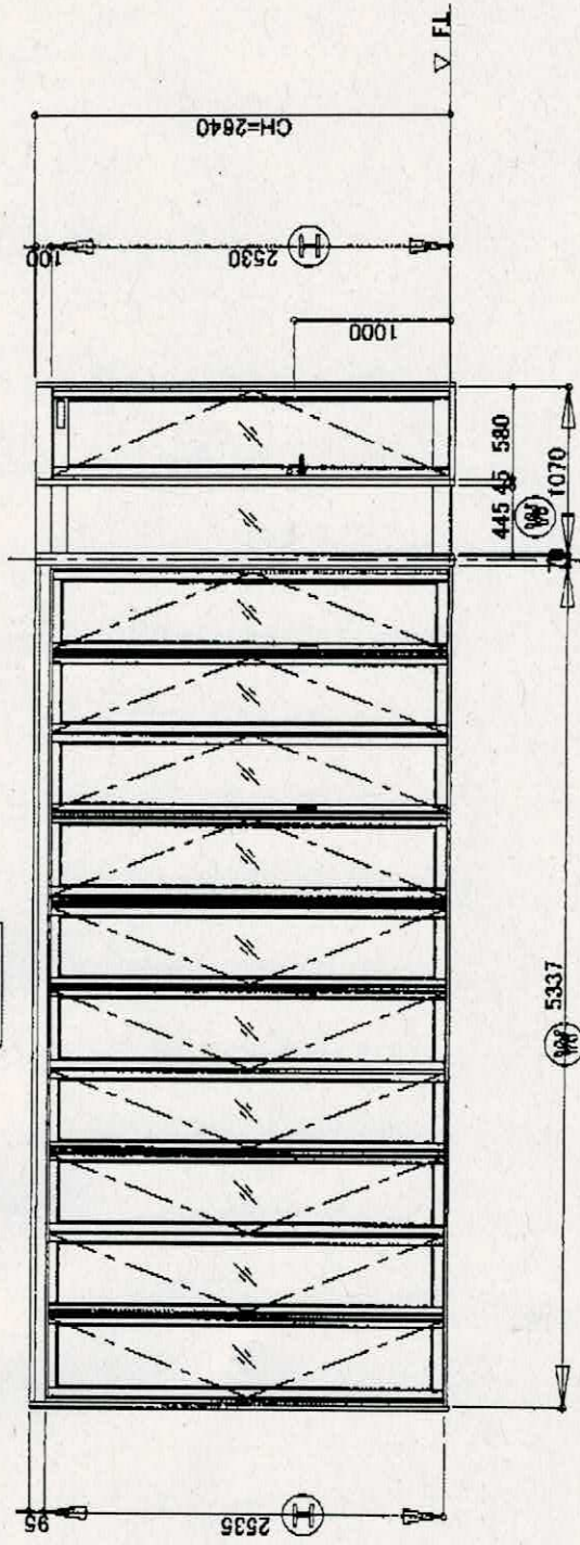
内観図
