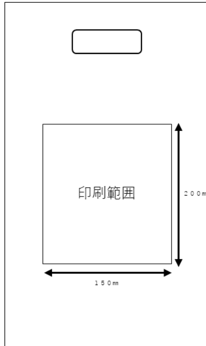
図2—ポリ袋規格
