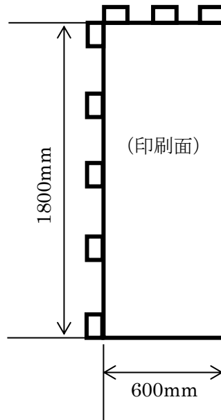
図1-のぼり寸法
