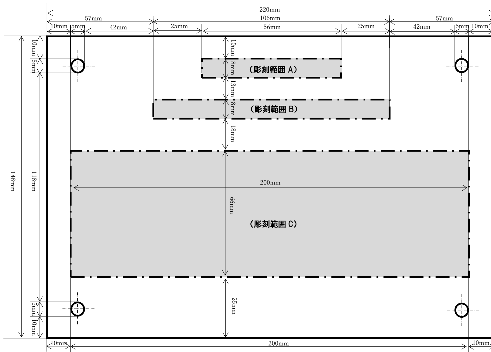
プレート寸法
