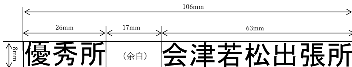
図2 彫刻寸法（彫刻範囲B）
