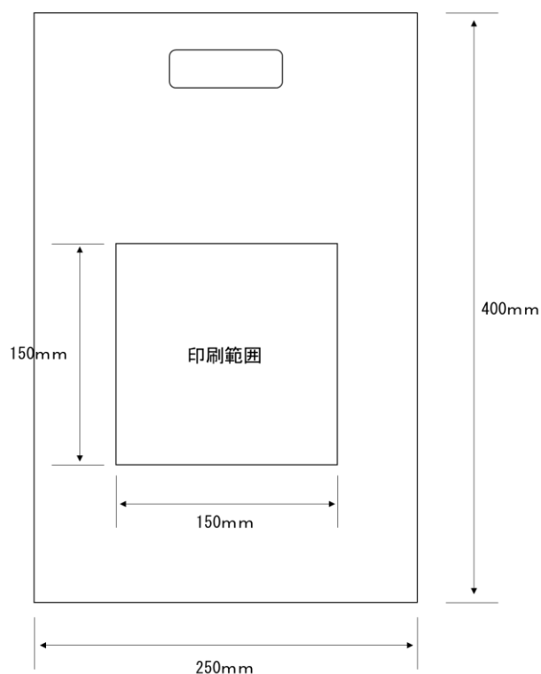
図2—ポリ袋規格
