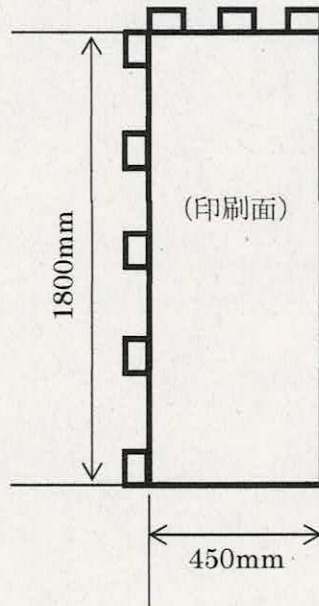
図1-のぼり寸法
