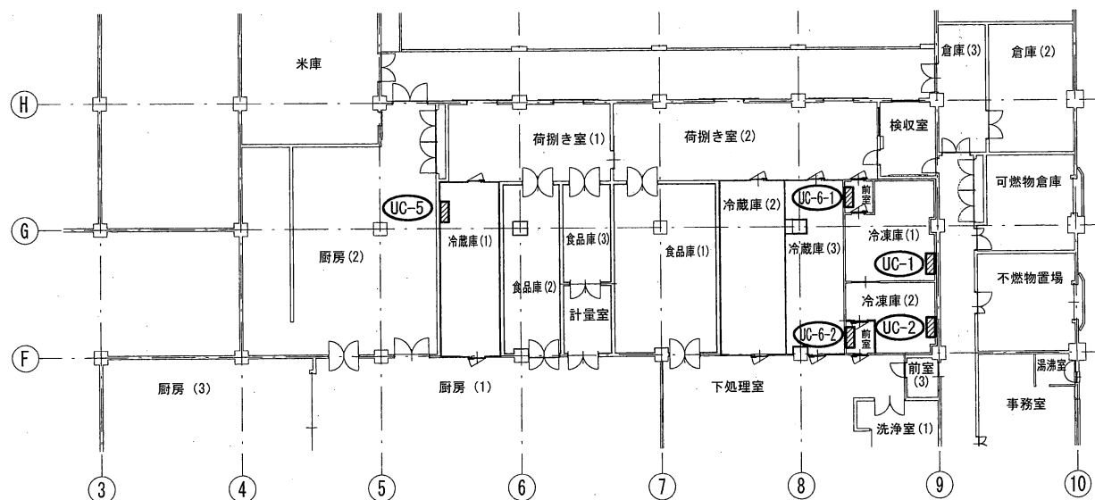
食堂棟1階冷凍庫前室平面図 S=N/S
