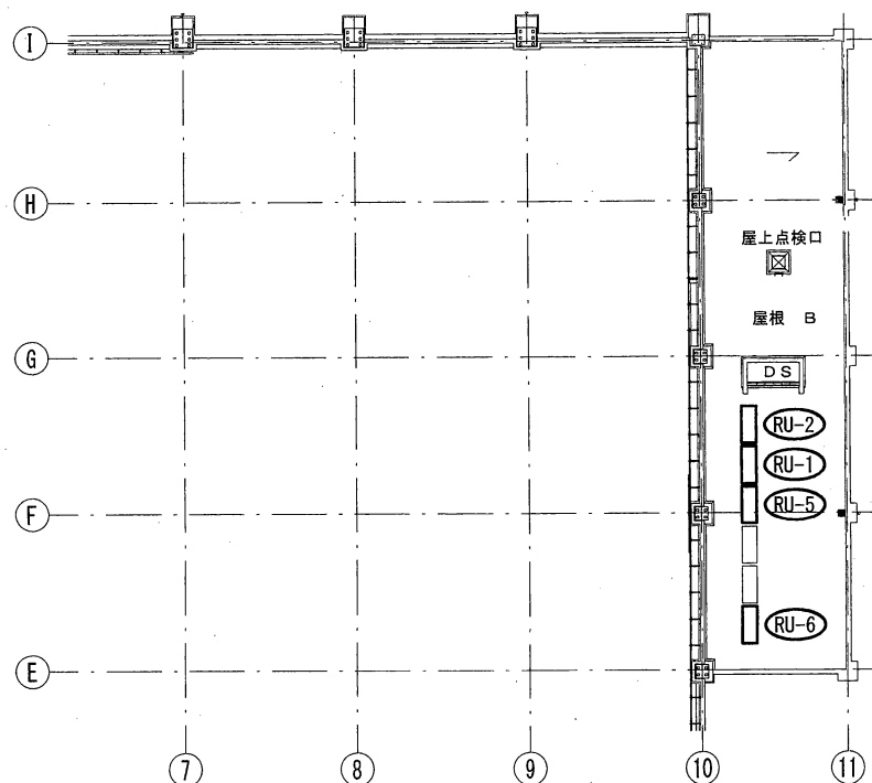
食堂棟屋上平面図 S=N/S
