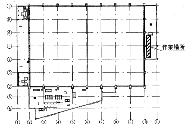
食堂棟屋上平面図 S=N/S
