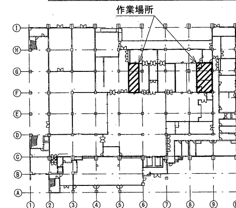
食堂棟1階平面図 S=N/S
