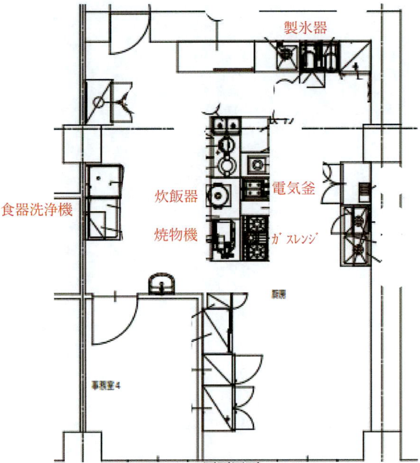
厨房図面
