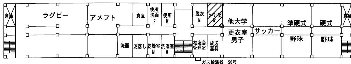
学生教育2号棟 2階平面図 S=N/S
