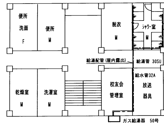
学生教育2号棟 2階詳細平面図 S = N/S
