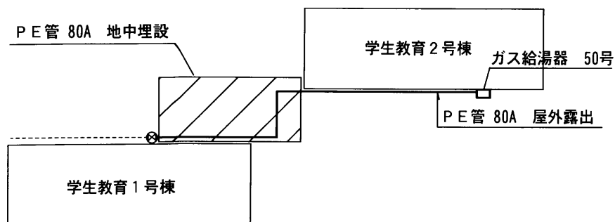
屋外配管図 S=N/S
