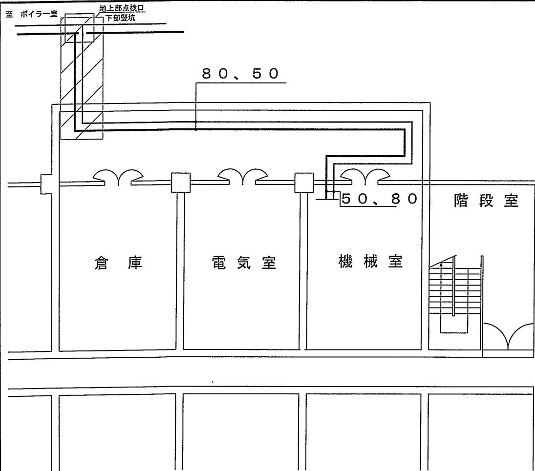
第3学生舎地下1階平面図 S=N/S
