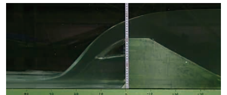
水理学：堤防を越える流れの性質を理解する。
