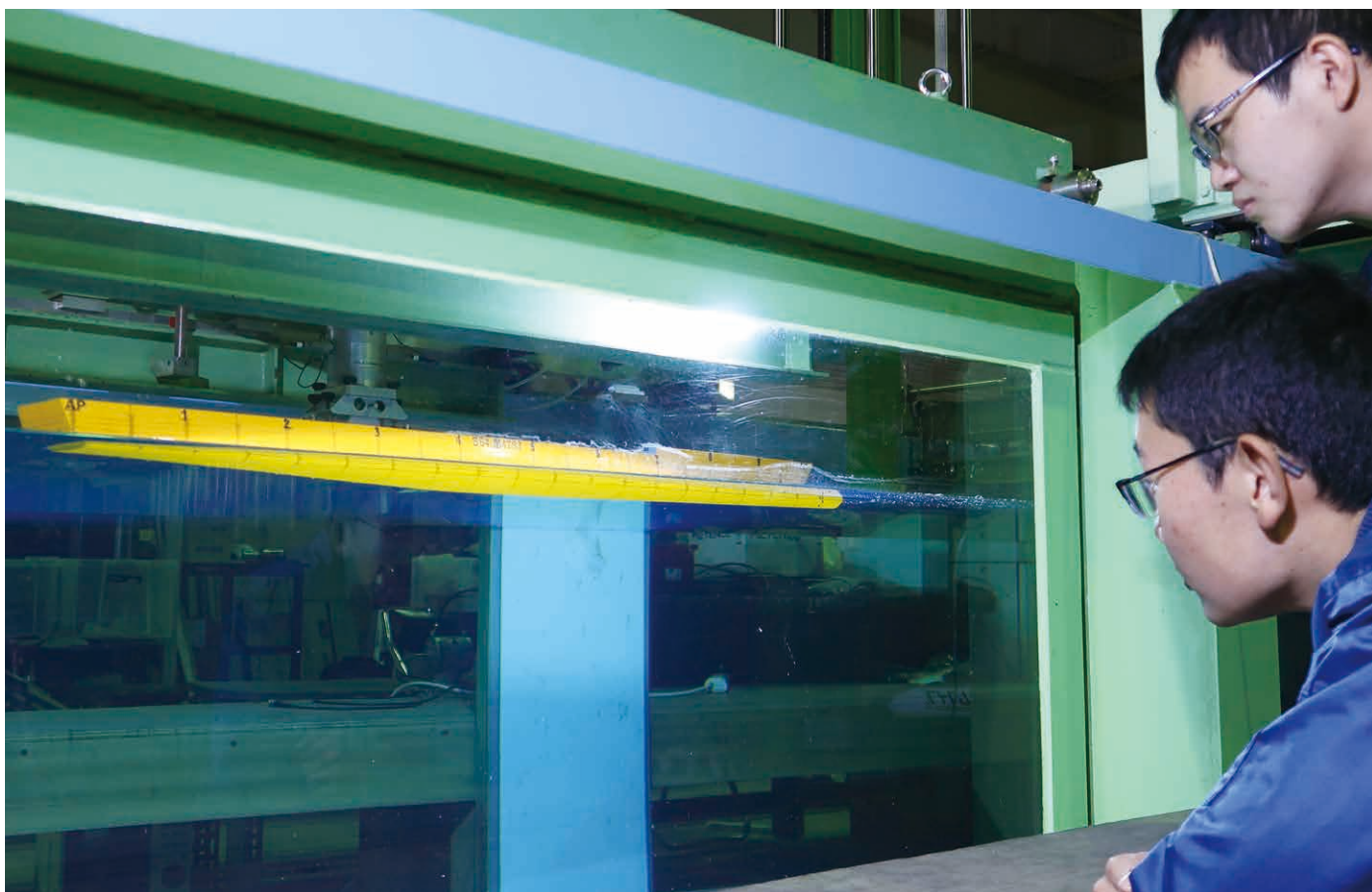
卒業研究（船舶工学講座）：高速回流水槽を用いた模型船の実験
