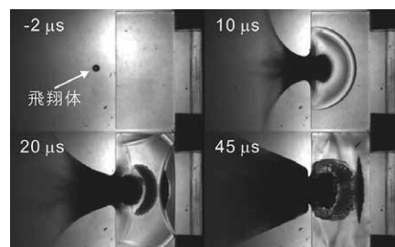
ポリカーボネート球が秒速6kmでポリカーボネートブロックに衝突した時の超高速撮影画像(高速弾道学研究室)
