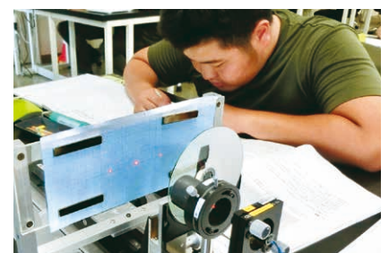
レーザー光の干渉の実験
