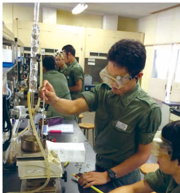
基礎科学実験(化学分野: 酢酸エチルの合成) 合成した酢酸エチルは精製した後、ガスクロマトグラフィーで分析します。
