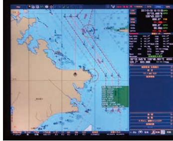
卒業研究（レーダ信号処理工学講座）：電子海図情報表示装置による観測実験
